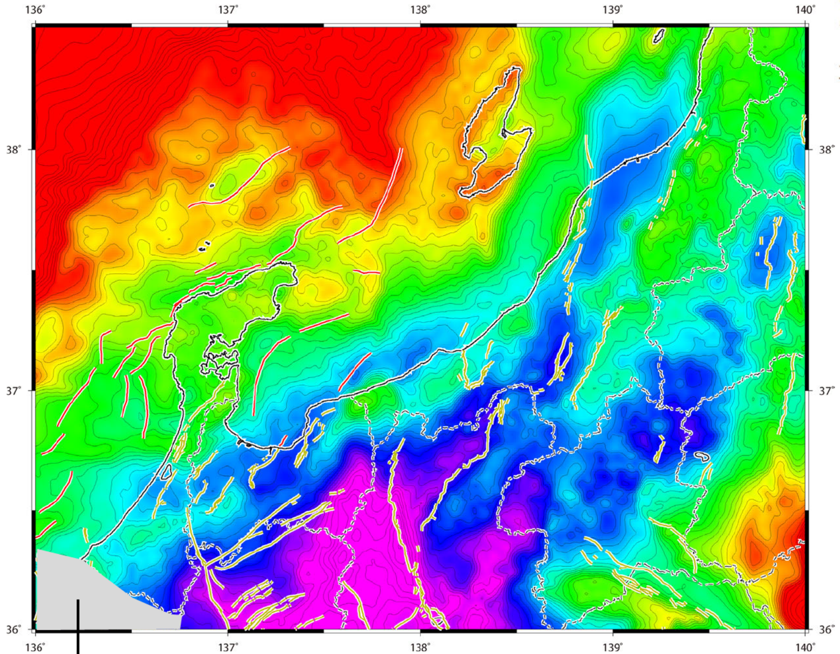
ブーゲー異常 (mgal) -50 -25 0 25 50 75 100 125
