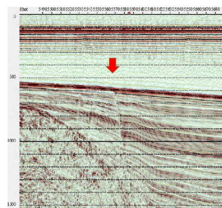
(d) 浦島礁北方冲断層
