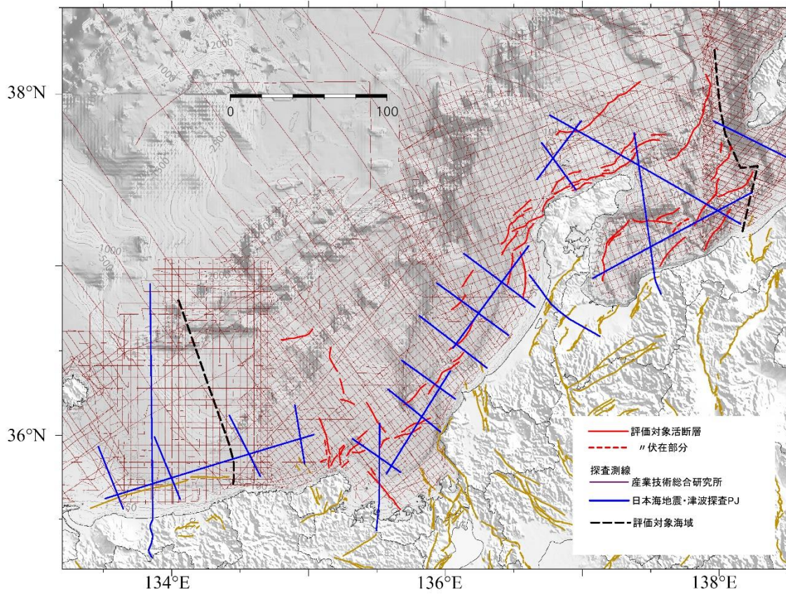
図3 評価対象海域の主な反射法地震探査測線
