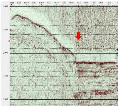
(s) 富山トラフ西縁断層帯
