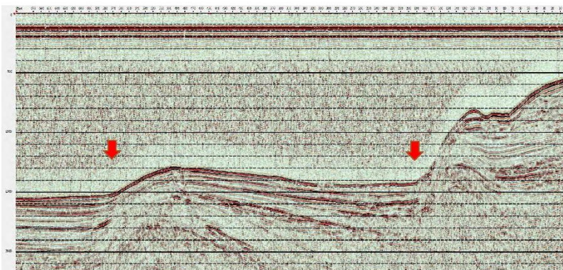
図4 海域活断層の反射断面例
