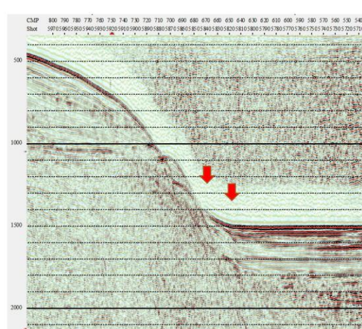
(q)-2 城ヶ崎沖区間
