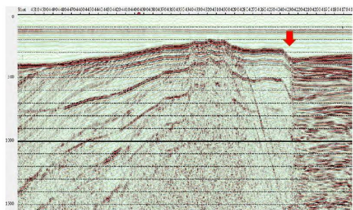
(d) 浦島礁北方冲断層
