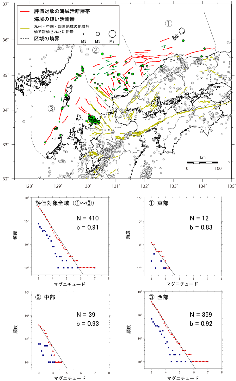
図 15 1997 年 10 月から 2024 年 3 月の評価対象海域における深さ 25 km 以浅の地震 (M3.0 以上) の規模 (マグニチュード) と規模別度数の経験式的回帰の結果 (データは気象庁提供)
