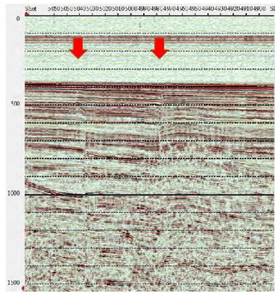
(a) 沖ノ礁北方断層
