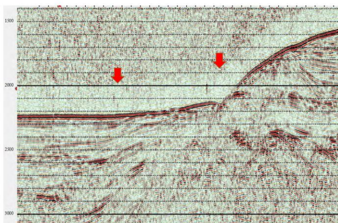
図5 海域活断層の反射断面例
