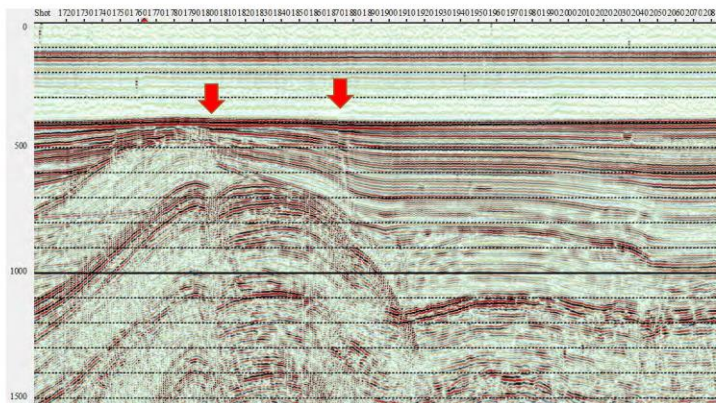
(f) 越前岬西方沖北断層
