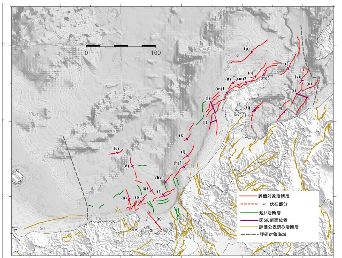
図4 図5に示した評価対象の海域活断層における反射断面の位置
