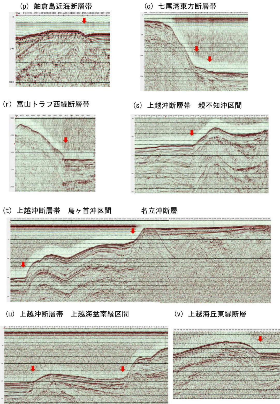
図5 海域活断層の反射断面例
