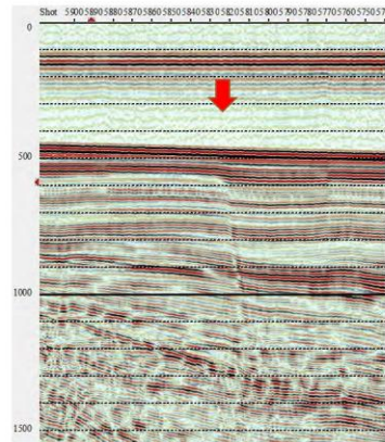
(g) 浦島礁北東断層
