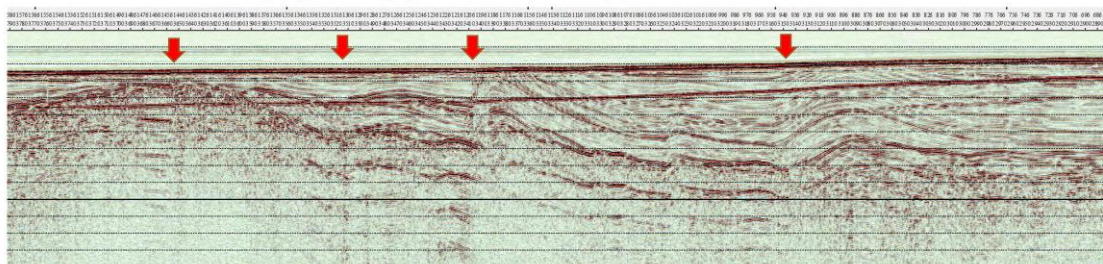
図5 海域活断層の反射断面例
