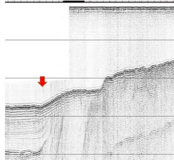
(m)-3 珠洲沖区間
