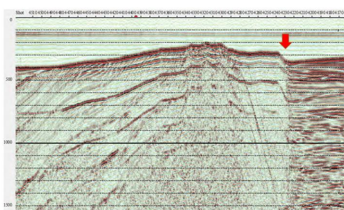
(d) 浦島礁北方冲断層
