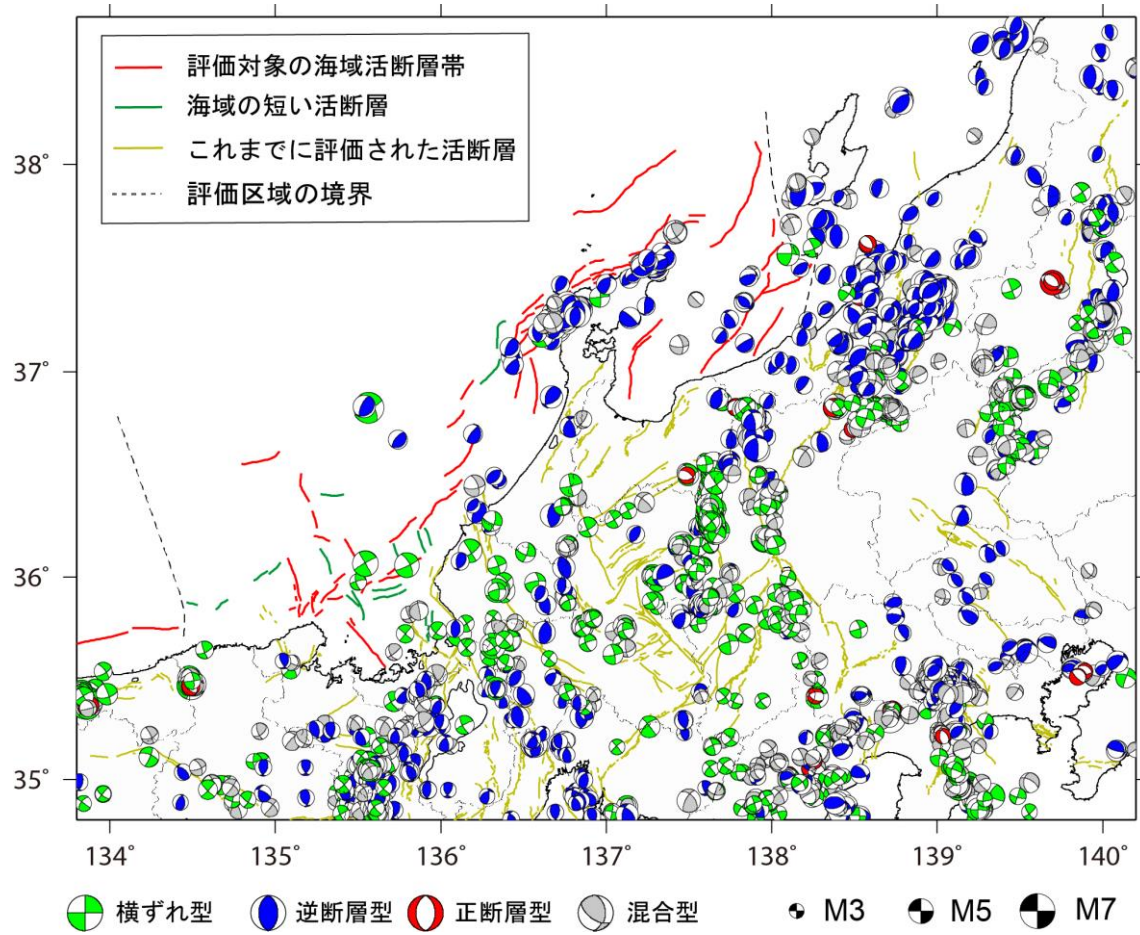
図8 評価海域周辺で発生した浅い地震の発震機構 (P波初動解、下半球投影) (1997年10月1日から2023年5月31日、深さ0から25km、 M \geq 3.0 、データは気象庁提供) 発震機構解の色は、Frohlich (2001) による断層型別の分類に基づき、逆断層型を青色、正断層型を赤色、横ずれ断層型を緑色、混合型を灰色で示した。
