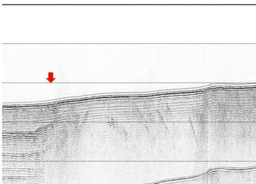
図5 海域活断層の反射断面例
