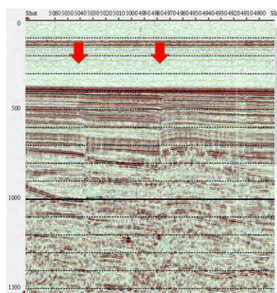
(a) 沖ノ礁北方断層
