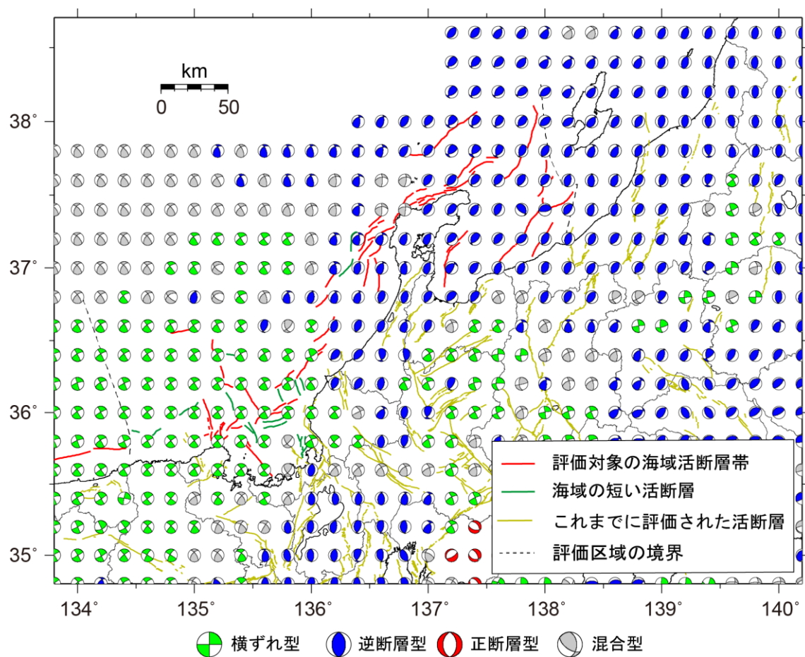
図9 評価海域周辺に分布する断層と三次元広域応力場（深さ 10km）
