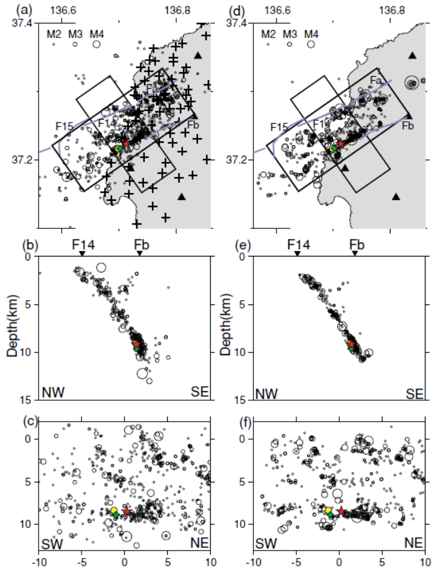
図7 海陸観測網による2007年能登半島地震の余震活動分布 (Sakai et al. 2008)
