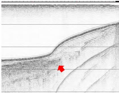
(m) 能登半島北岸断層帯 (m)-1 猿山沖区間
