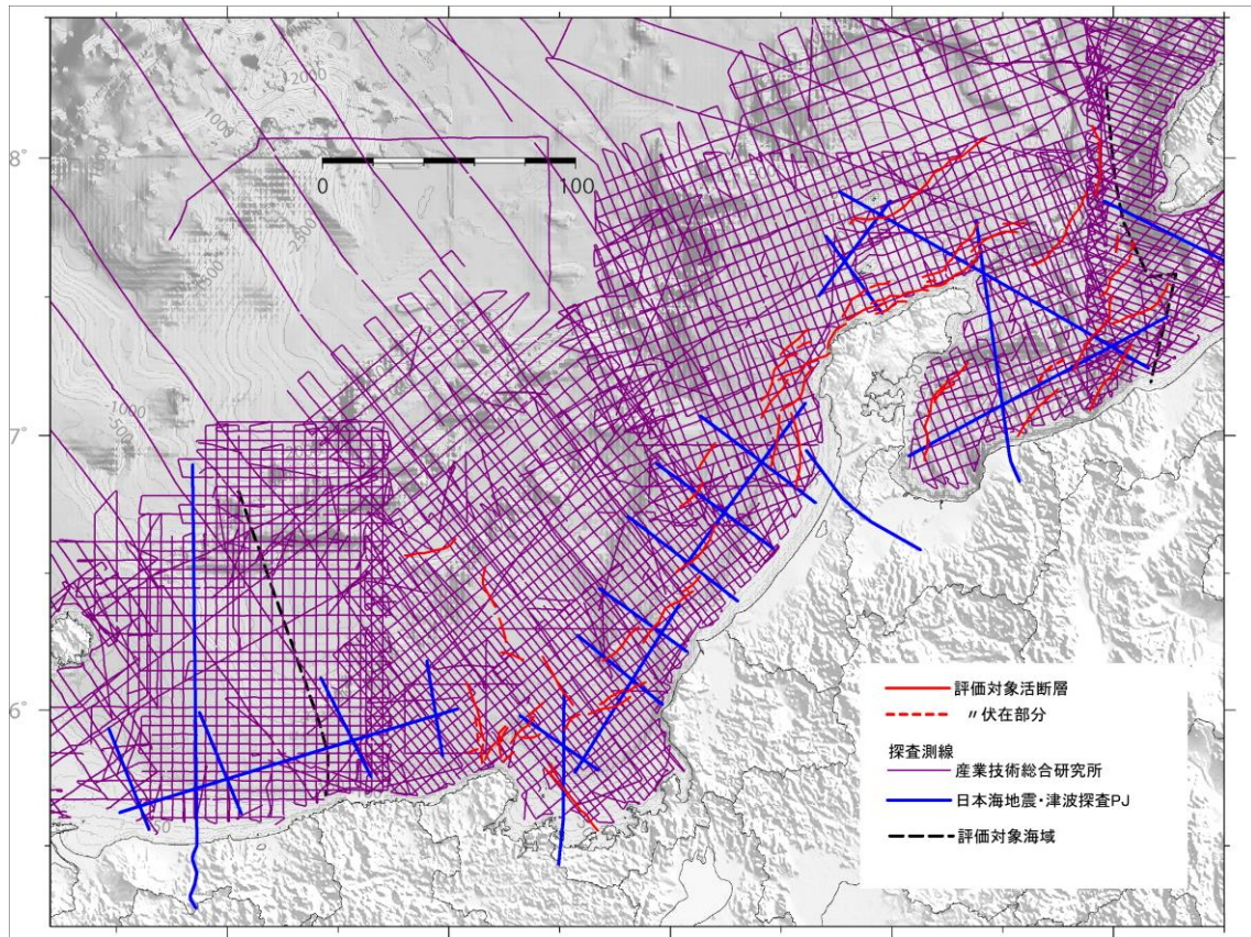
図3 評価に用いた主な反射法地震調査測線
