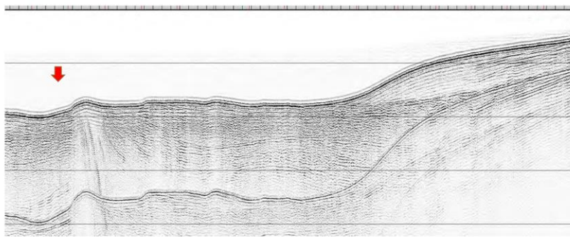
(n) 輪島はるか沖断層
