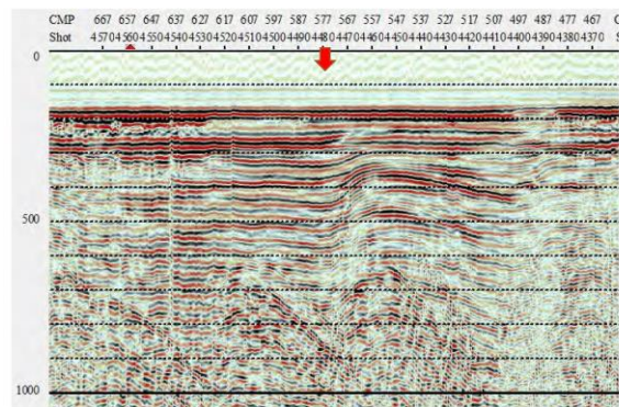
図5 海域活断層の反射断面例
