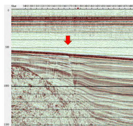
(d) 浦島礁北方冲断層
