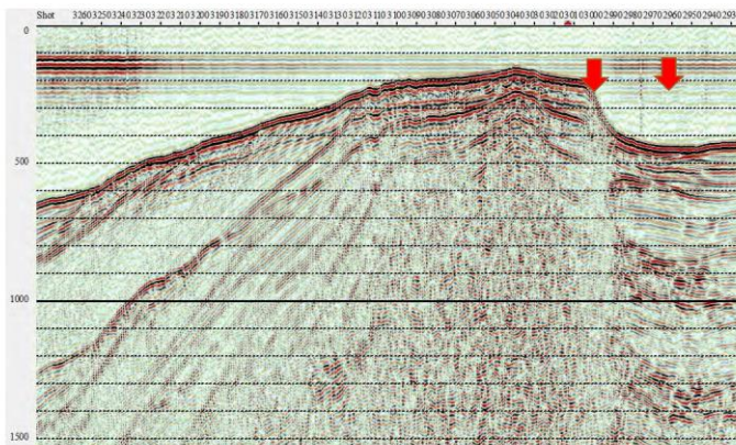
(h)-2 大グリ区間
