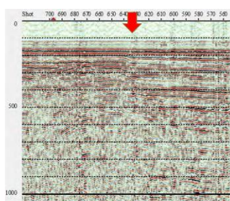
(e) 若狭海丘列北縁断層
