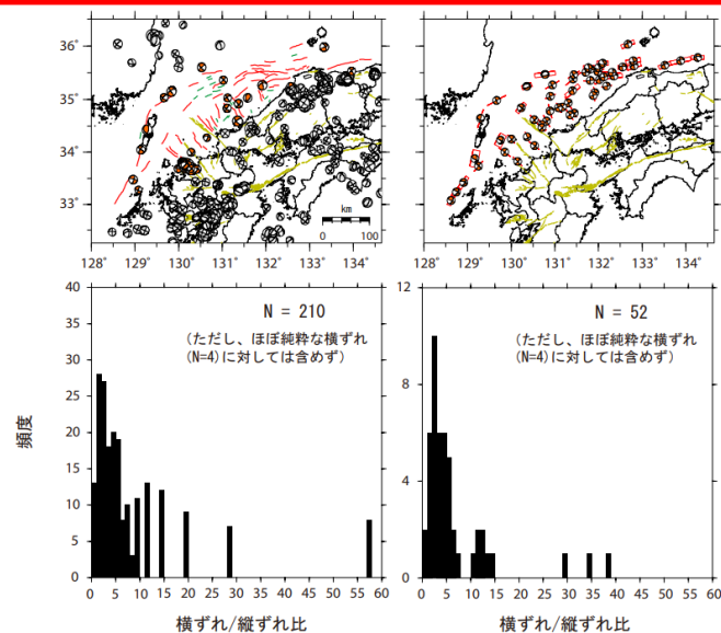
日本海南西部の横ずれ／縦ずれ比の推定手法
