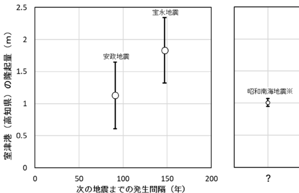
図5 室津港（高知県）における南海地震時の隆起量と次の地震発生間隔までの期間との関係 階段状丸印とエラーバーは各々の赤線の縦軸が地震によって隆起した量より室津港の隆起量の確率密度分布の期待値と同分布の標準偏差（ 1\sigma ）をそれぞれ示す。水色の線は宝永地震時および安政地震の積算隆起量と次の平均隆起速度。このモデル
