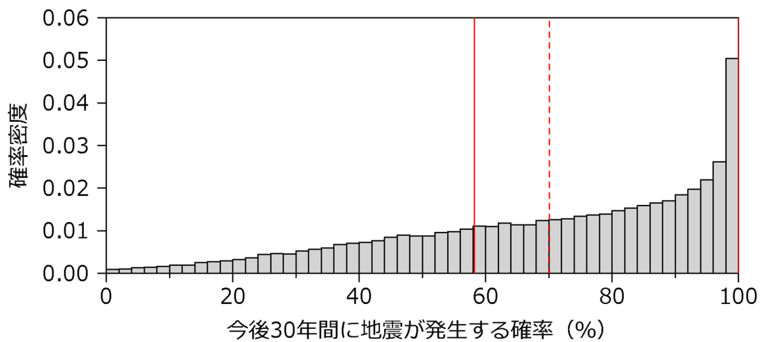
図 4-4 時間予測モデルによる 今後 30 年間に南海トラフで大地震が発生する確率の事後分布 (SSD-BPT) 評価時点 (2025 年 1 月 1 日) における 30 年以内確率の頻度分布。赤色の実線は 70%信用区間、赤色の破線は期待値 (平均値) を示す。
