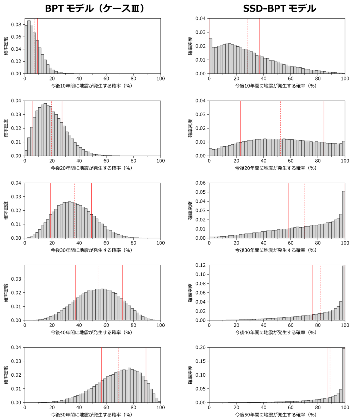
図 4-8 BPT モデルと SSD-BPT モデルによる発生確率の事後分布を使用し、ばらつきの比較 評価時点（2025 年 1 月 1 日）から今後 10、20、30、40、50 年間に地震が発生する確率の頻度分布。左側が BPT モデル（ケースⅢ）、右側が SSD-BPT モデルによる確率を表すパラメータ \alpha の値が 0.24 と 0.20 の時の確率値の時間推移を各々赤線、青線で。各分布において、赤色の実線は 70%信用区間、赤色の破線は期待値（平均値）を示す。
