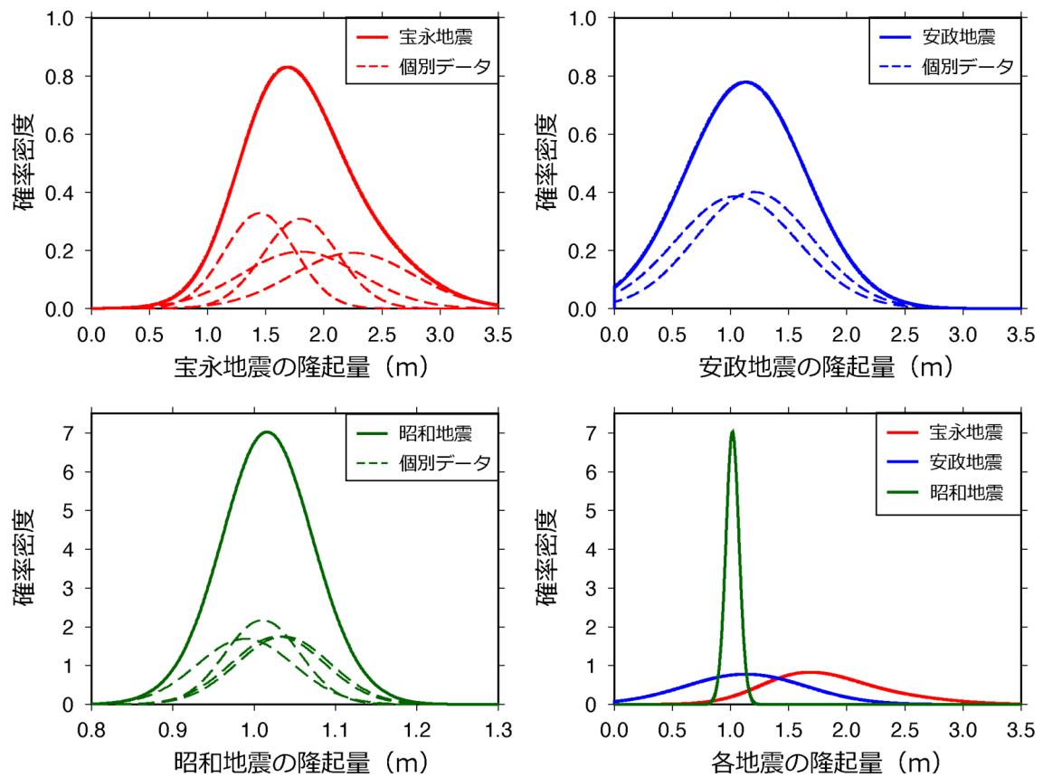
図 4-4 各南海トラフ地震における南海地震時室津港の隆起量と地震発生間隔とデータの関係確率分布
