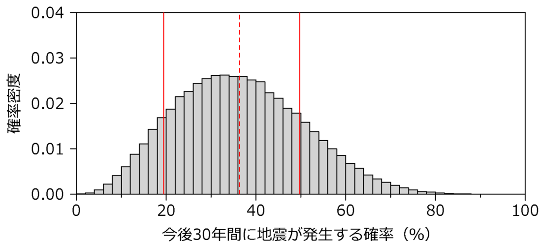
図 4-2 南海トラフにおける今後 30 年間に地震南海トラフで大地震が起きる発生する確率と、前地震からの経過時間の関係（赤線：事後分布（BPT、ケースⅠ、緑線：ケースⅡ、青線：ケースⅢ、シアン：ケースⅣ、マゼンタ：ケースⅤⅢ）線上の●は各ケースにおいて実際に地震が起きた時の経過時間とその時の評価時点（2025 年 1 月 1 日）における 30 年確率。橙色の頻度分布。赤色の実線は 70%信用区間、赤色の破線は評価した時点（2013 年 1 月 1 日）の経過時間期待値（平均値）を示す。
