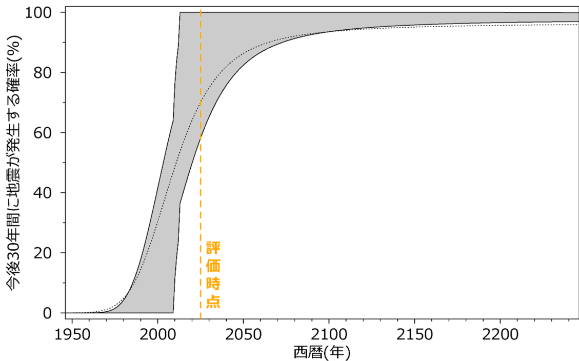
図 4-6 今後 30 年間に南海トラフで大地震が発生する確率の時間推移 (SSD-BPT) 70%信用区間の範囲を灰色、上限と下限を黒の実線で示す。黒色の波線は期待値の推移を示す。橙色の破線は評価時点 (2025 年 1 月 1 日)、山吹色の破線は前回評価時点 (2001 年 1 月 1 日) を示す。なお、図中の確率分布として推移は評価時点で得られたパラメータの事後分布に基づく。
