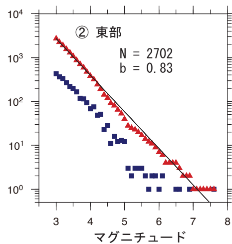
図9 1997年10月から2024年12月の日本海中南部における深さ30 km 以浅の地震（M3.0以上）の規模（マグニチュード）と規模別度数の経験式の回帰の結果（データは気象庁提供）
