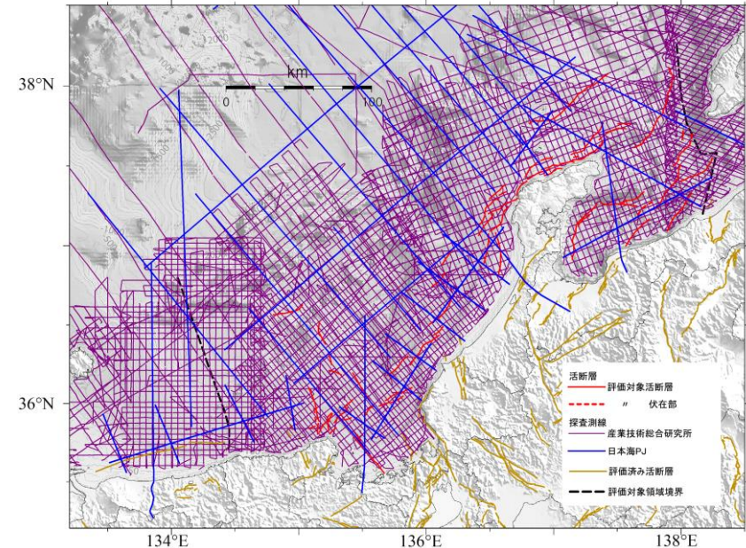
評価対象海域の主な反射法地震調査測線
