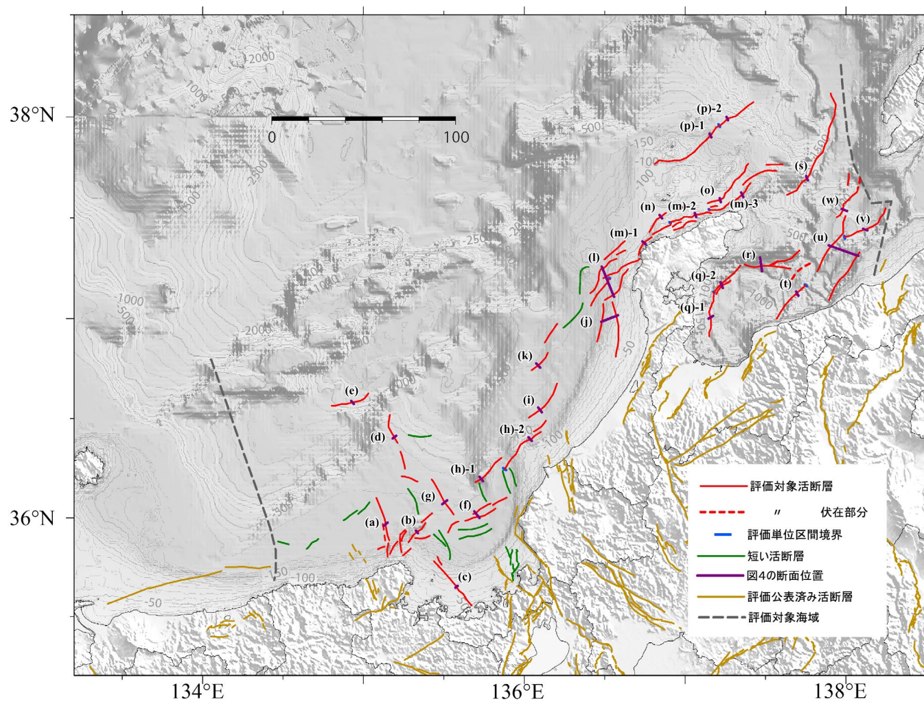
図5 図4-1～図4-6に示した評価対象の海域活断層における反射断面の位置
