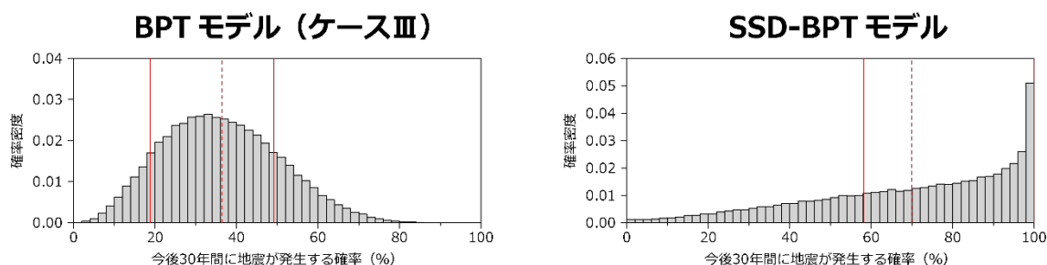
図6 南海トラフにおける今後30年間に地震が発生する確率の事後分布の比較 ・評価時点（2025年1月1日）から今後30年間に地震が発生する確率の事後分布。 左側がBPTモデル（ケースⅢ）、右側がSSD-BPTモデルによる確率を表す。各分布に おいて、赤色の実線は70%信用区間、赤色の破線は期待値（平均値）を示す。
