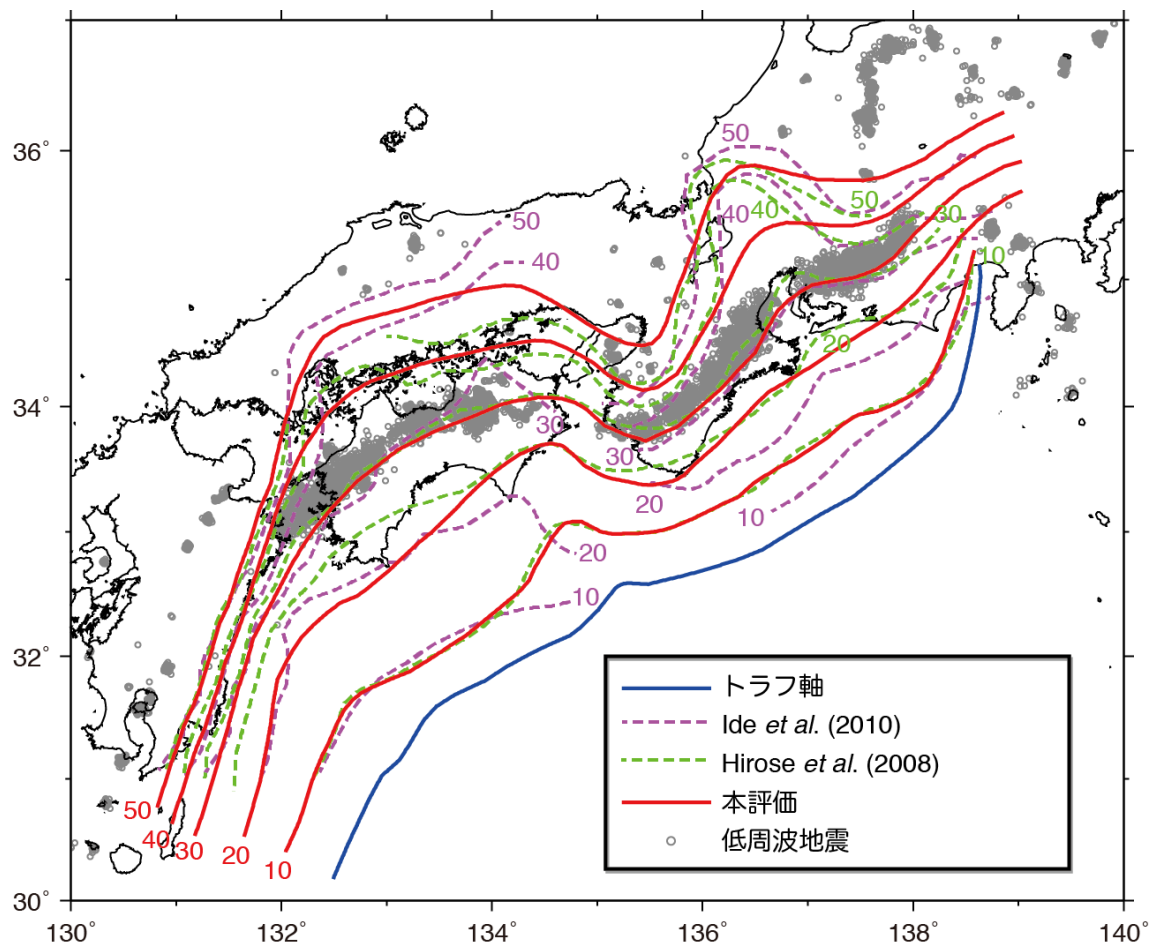
図 2-3 南海トラフから沈み込むフィリピン海プレートの上層深度 (本評価 (第二版及びその一部改訂の評価) で用いた深度は内閣府 (2011) による)
