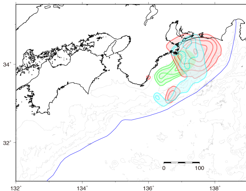
5 6 図3-17 1944年昭和東南海地震のすべり量分布図 7 最大すべりの半値以上すべった領域を塗りつぶした。すべり量のコンター間隔は0.4m。 8 緑：Kikuchi et al. (2003)、水色：Ichinose et al. (2003)、赤色：山中 (2006) のす 9 べり量分布。すべり量の半値は各々、2.2 m、1.2 m、1.6 mとなる。
