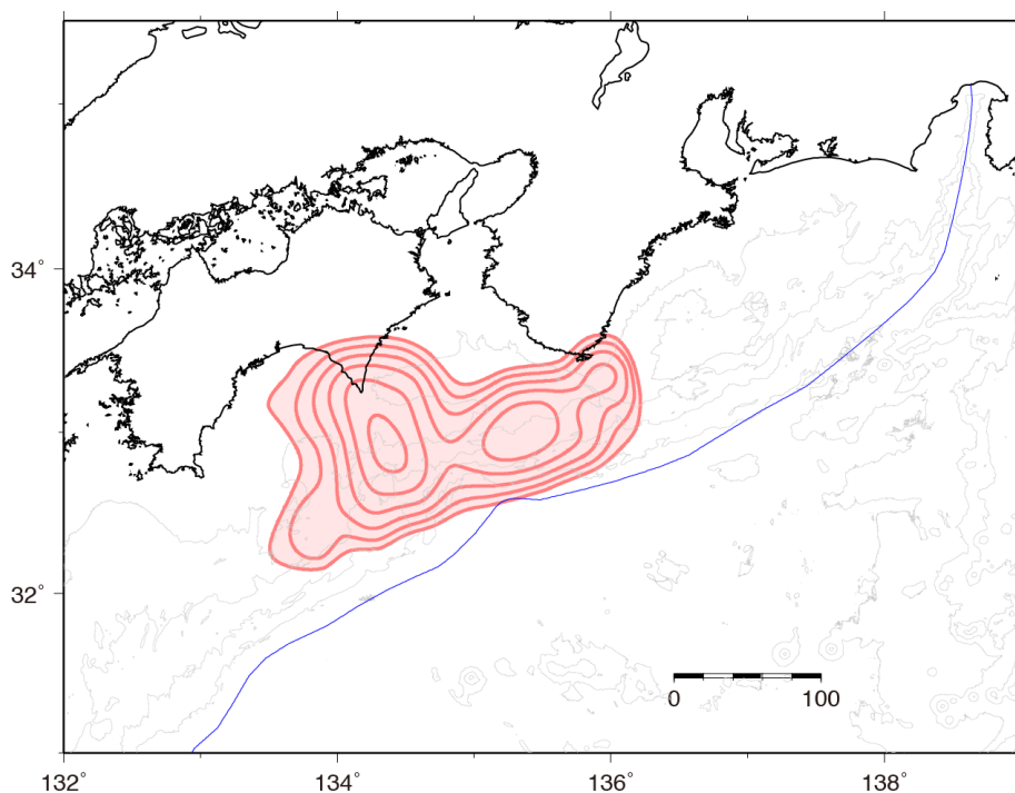
1 2 図 3-16 1946 年昭和南海地震のすべり量分布図 (Murotani, 2007) 3 最大すべりの半値 (2.5 m) 以上すべった領域を塗りつぶした。すべり量のコンター間隔 4 は 0.5 m。
