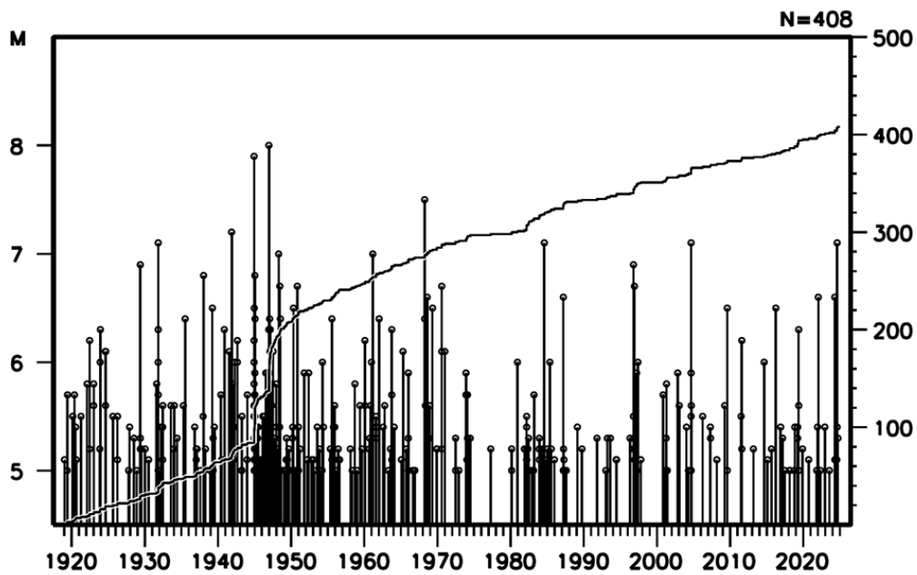
図 3-30 南海トラフの地震活動の M-T 図及び回数積算図（気象庁作成）
