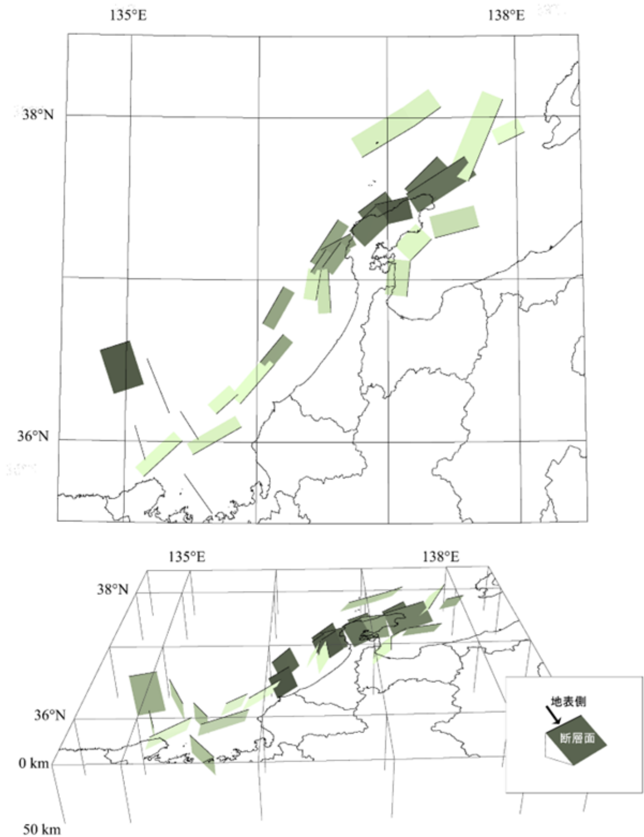
図18 評価対象の海域活断層（帯）の矩形断層モデル
