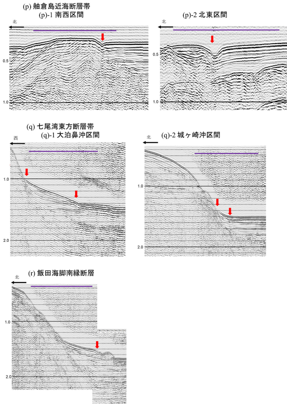
図4-5 海域活断層の反射断面例
