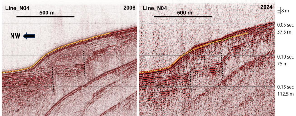
図3 2008年（左）及び2024年（右）のN04測線（猿山岬沖セグメント）ブーマー断面。断層（黒点線）の南東側に3～4mの隆起が認められる。
