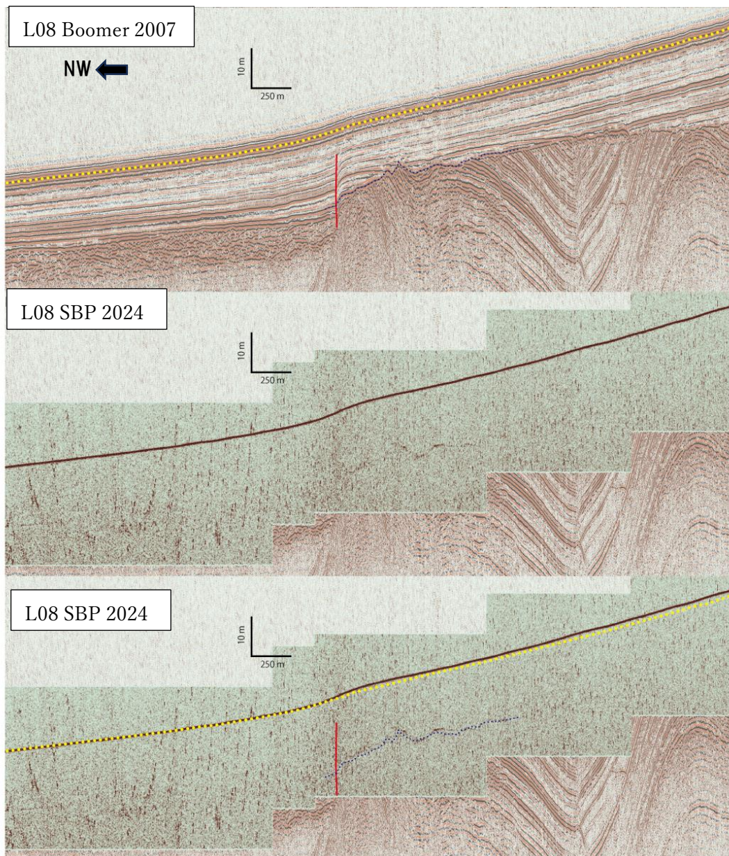
図2 L08 測線（門前沖セグメント）の 2007 年ブーマー断面（上）及び 2024 年 SBP 断面（中）で、下段に 2024 年 SBP 断面に黄色点線で 2008 年以前の地形断面（以下同じ）を示す。断層（赤線）の南東側に 1m 前後の隆起が認められる。
