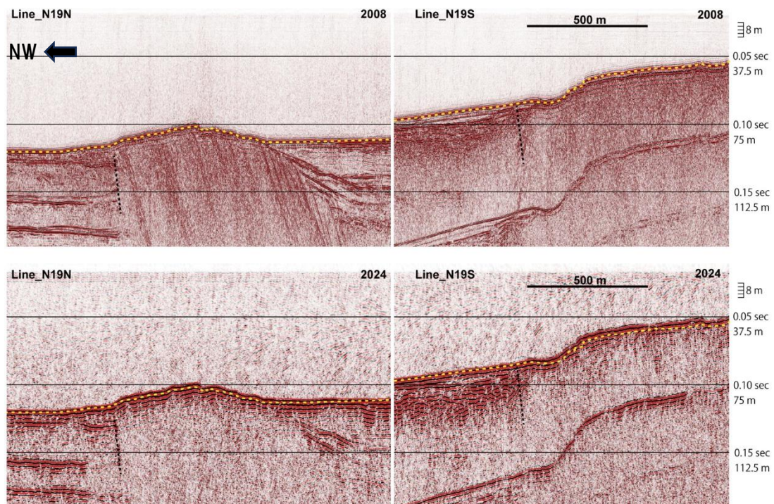
図5 2008年（上）及び2024年（下）のN19測線ブーマー断面（輪島沖セグメント）。北側（N19N）及び南側（N19S）の断層（黒点線）の南東側に1～2 mの隆起が認められる。
