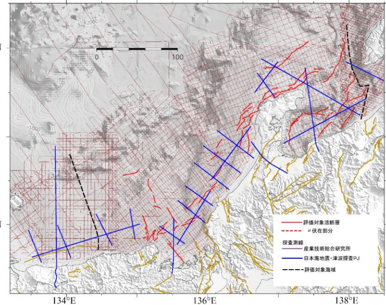
評価対象海域の主な反射法地震探査測線
