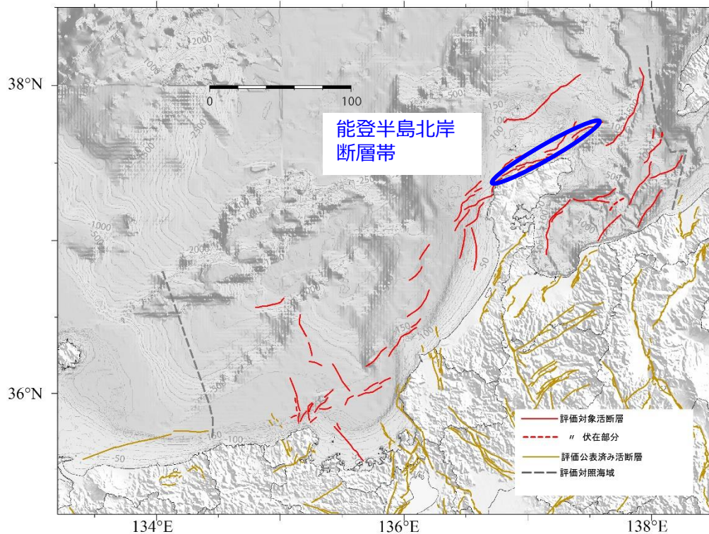
評価対象の海域活断層帯のトレース（赤線）
