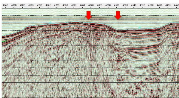
(h)-2 大グリ区間
