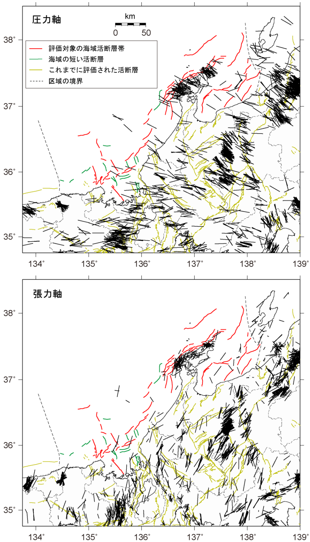
図9 評価対象領域内の発震機構の圧力軸（上）と張力軸（下）の分布
