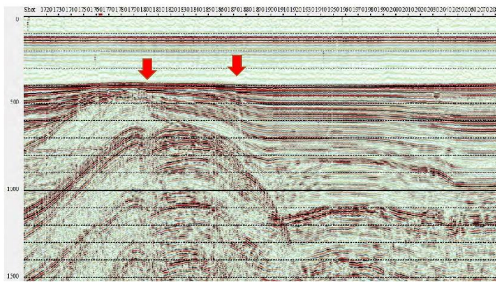
(h) ゲンタツ瀬・大グリ南東縁断層帯
