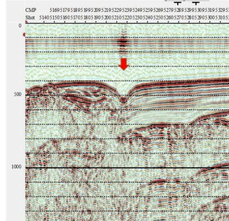
(q)-2 城ヶ崎沖区間
