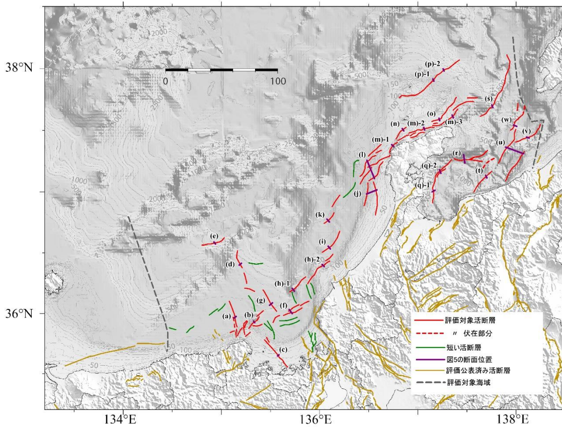
図5 図4に示した評価対象の海域活断層における反射断面の位置
