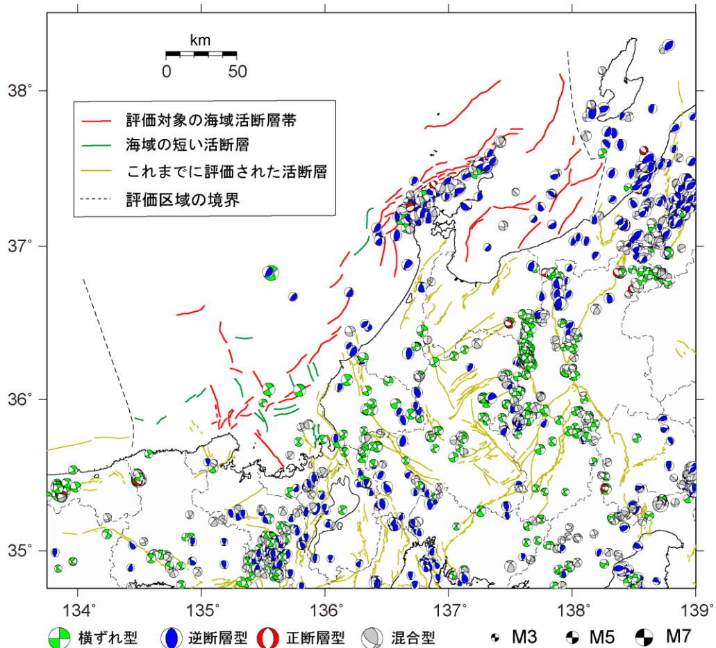
図 8－1 評価対象海域ならびにその周辺で発生した浅い地震の発震機構（P 波初動解、下半球投影）（1997 年 10 月 1 日から 2024 年 3 月 31 日、深さ 0 から 25km、 M \geq 3.0 、データは気象庁提供）発震機構解の色は、Frohlich (2001) による断層型別の分類に基づき、逆断層型を青色、正断層型を赤色、横ずれ断層型を緑色、混合型を灰色で示した。
