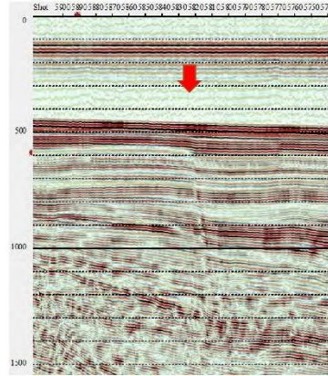
(g) 浦島礁北東断層
