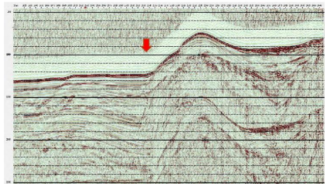
(t) 上越沖断層帯 親不知沖区間
