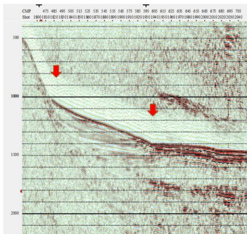
(q) 七尾湾東方断層帯 (q)-1 大泊鼻沖区間
