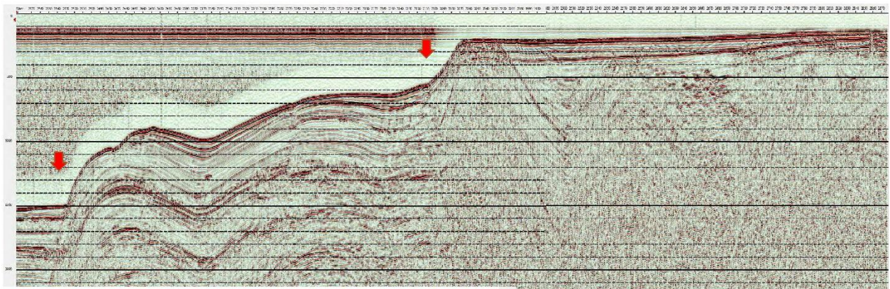
(u) 上越沖断層帯 鳥ヶ首沖区間
