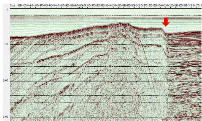
(d) 浦島礁北方沖断層
