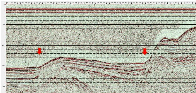
図4 海域活断層の反射断面例
