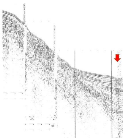
図4 海域活断層の反射断面例
