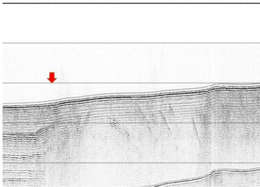
図4 海域活断層の反射断面例
