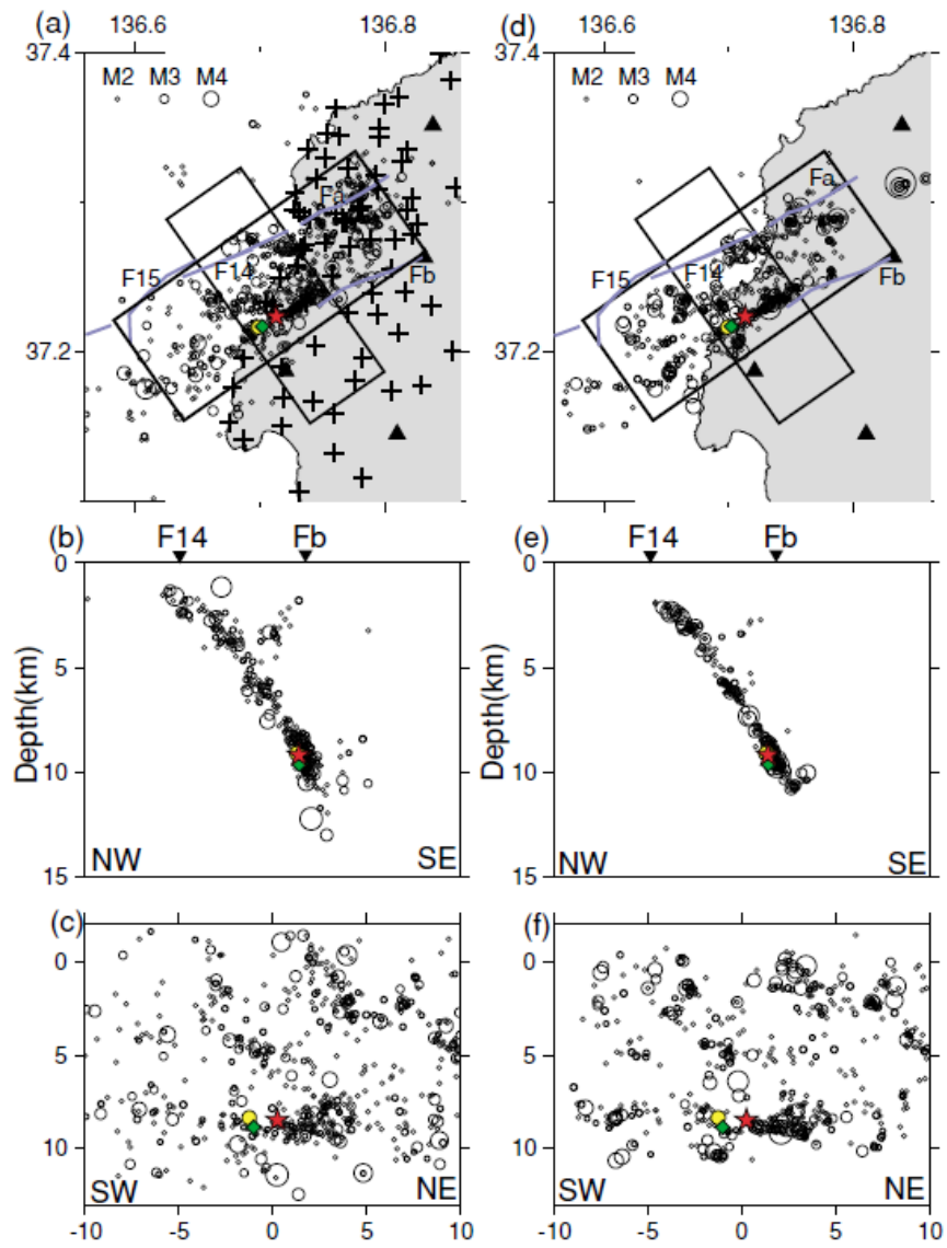
図7 海陸観測網による2007年能登半島地震の余震活動分布 (Sakai et al. 2008)
