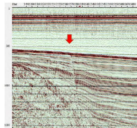
(d) 浦島礁北方沖断層
