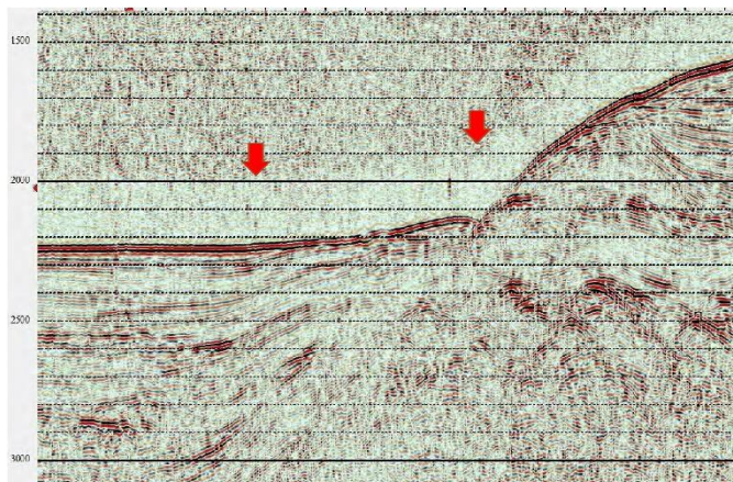
図4 海域活断層の反射断面例
