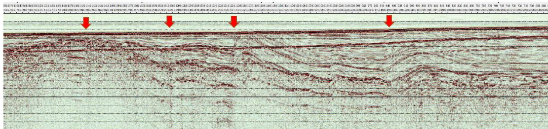
図4 海域活断層の反射断面例
