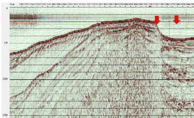
(h)-2 大グリ区間
