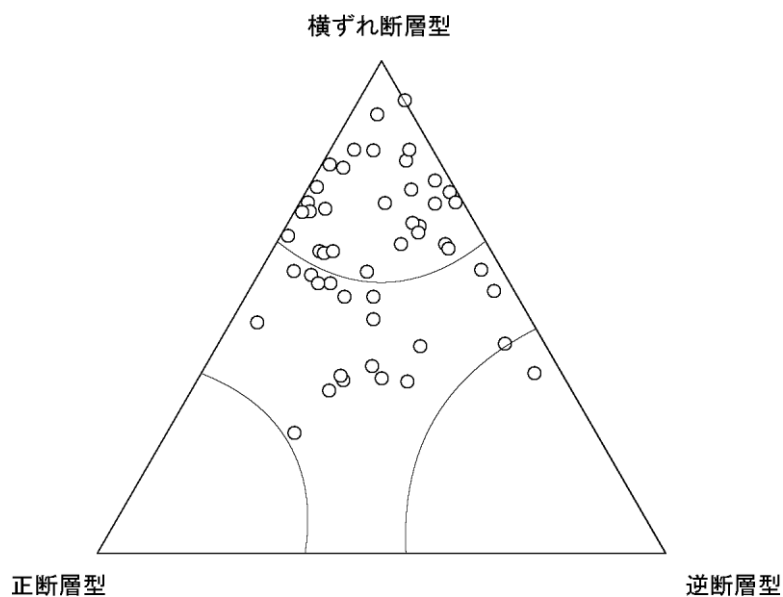
図 8－2 評価対象領域内で発生した地震の発震機構の分布（データは気象庁提供） （図は日本海南西部の海域活断層の長期評価（第一版）による。差し替え予定）
