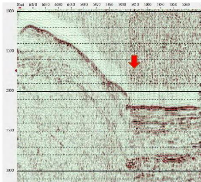
(u) 上越沖断層帯 鳥ヶ首沖区間
