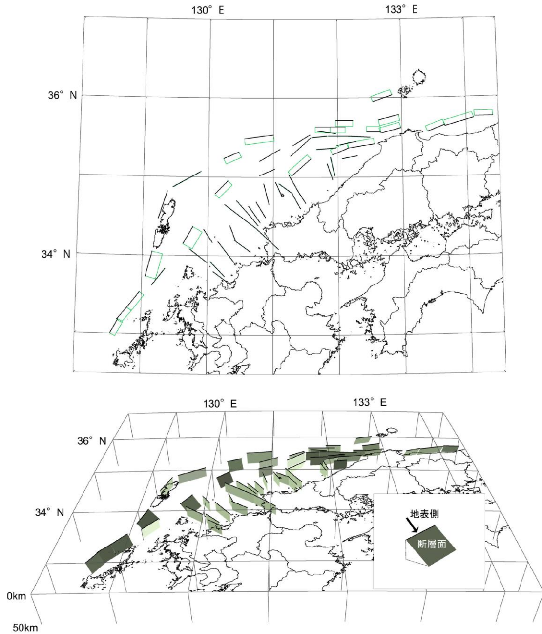
図 14 評価対象の海域活断層帯の矩形断層モデル
