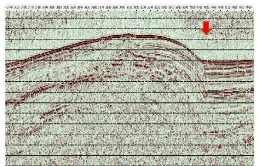
(w) 上越海丘東縁断層
