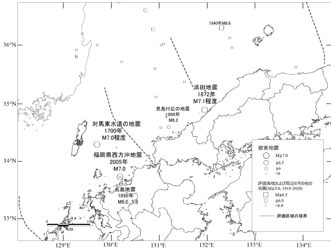
図 16 評価対象海域で発生したと考えられる主な歴史・被害地震
