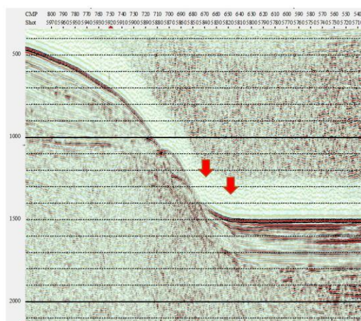
(q)-2 城ヶ崎沖区間
