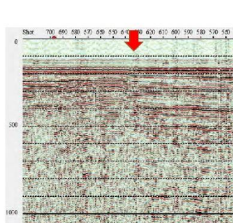
(e) 若狭海丘列北縁断層
