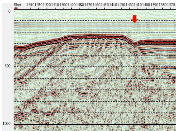
(q) 七尾湾東方断層帯 (q)-1 大泊鼻沖区間
