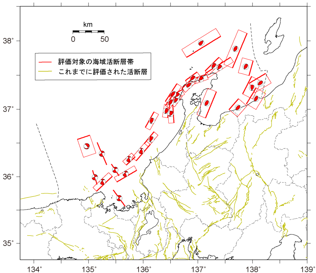
付図2 三次元広域応力場 (Terakawa and Matsu' ura 2010) から推定した断層すべり 角の分布 (特性表確定後、修正)
