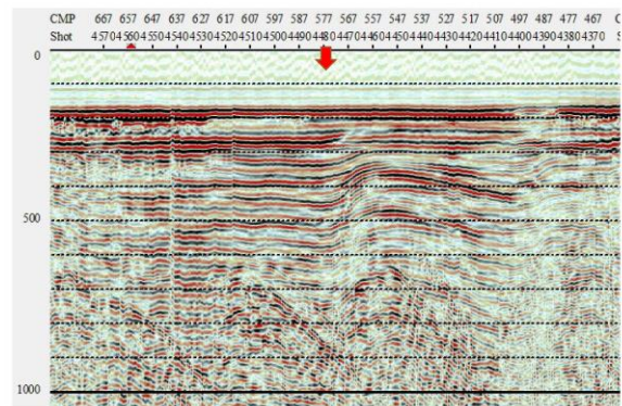
図4 海域活断層の反射断面例
