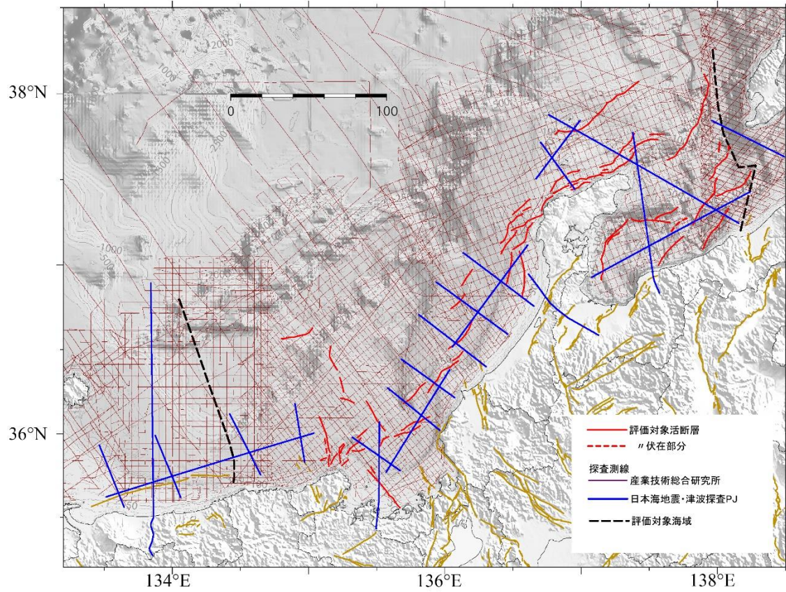
図3 評価対象海域の主な反射法地震調査測線
