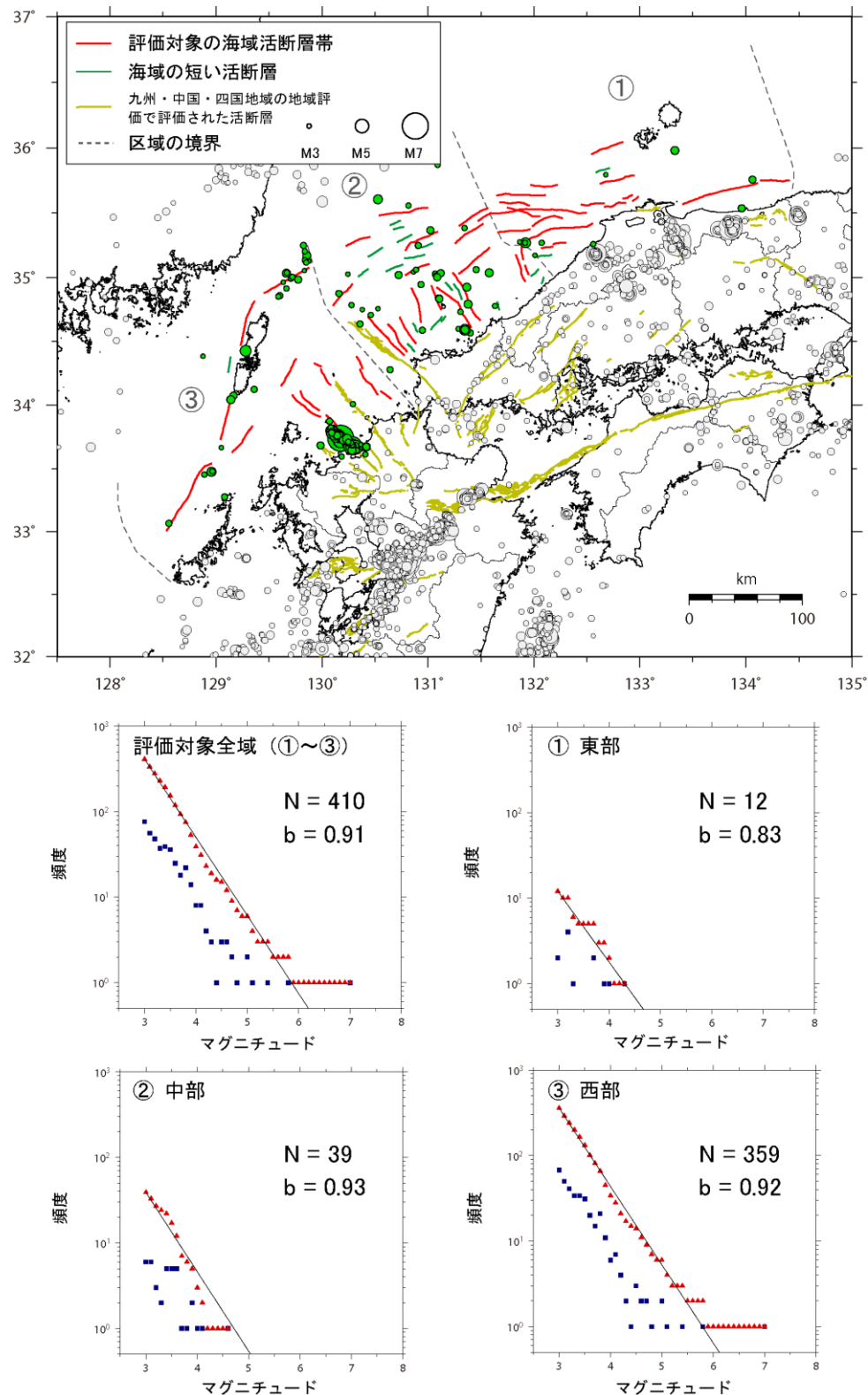
図 15 1997 年 10 月から 2024 年 3 月の評価対象海域における深さ 25 km 以浅の地震 (M3.0 以上) の規模 (マグニチュード) と規模別度数の経験式の回帰の結果 (データは気象庁提供)
