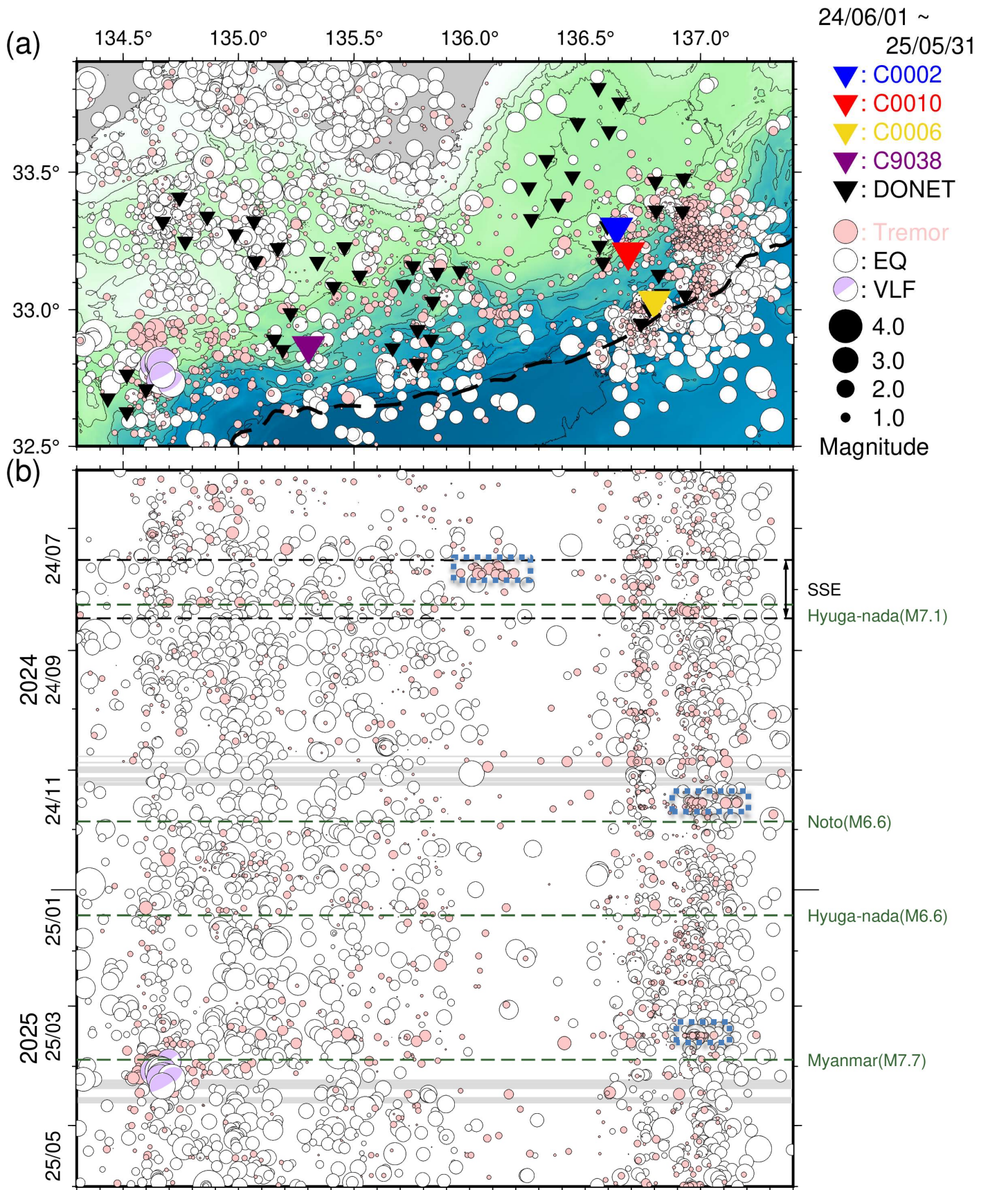
図 6 直近 1 年間に於いて熊野灘から室戸沖にて発生した低周波微動・通常地震・超低周波地震 (2024 年 6 月 1 日~2025 年 5 月 31 日)。図 4 と同様のシンボルにて表示。(a) 震央分布図。(b) a に示した震央を経度方向へ投影した時空間分布図。青点線の長方形領域は、これまでの評価文において言及した微動活動を示す。なお、過去資料の図 3 及び図 5 に緑点線で記した地震のうち、a の領域外かつ M6.5 未満のものは掲載していない。
