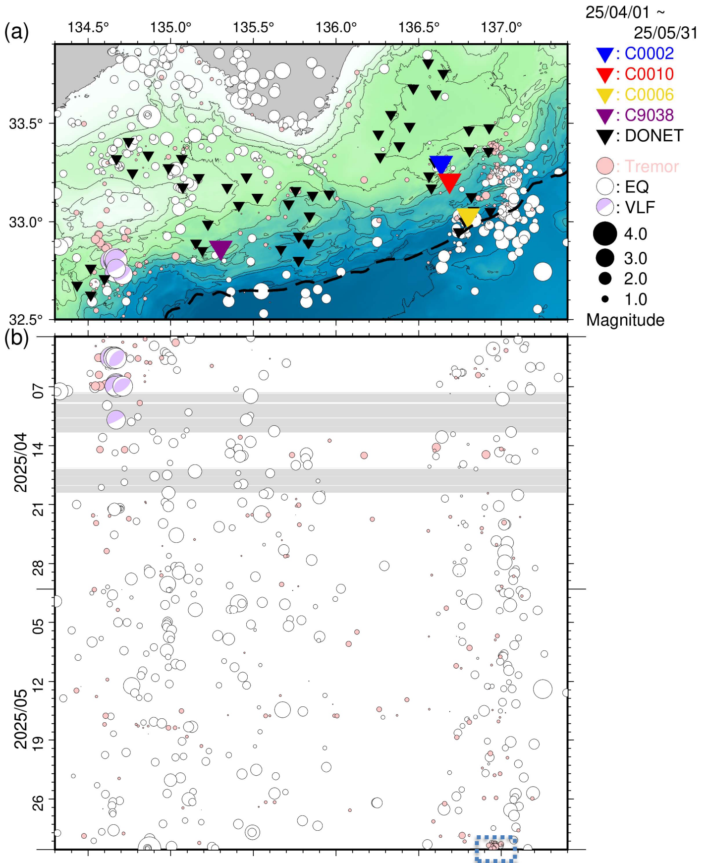
図5 直近2ヵ月間において熊野灘から室戸沖にて発生した低周波微動・通常地震・超低周波地震 (2025年4月1日~2025年5月31日)。図3と同様のシンボルにて表示。(a) 震央分布図。(b) aに示した震央を経度方向へ投影した時空間分布図。青点線の長方形領域は、これまでの評価文において言及した微動活動を示す。
