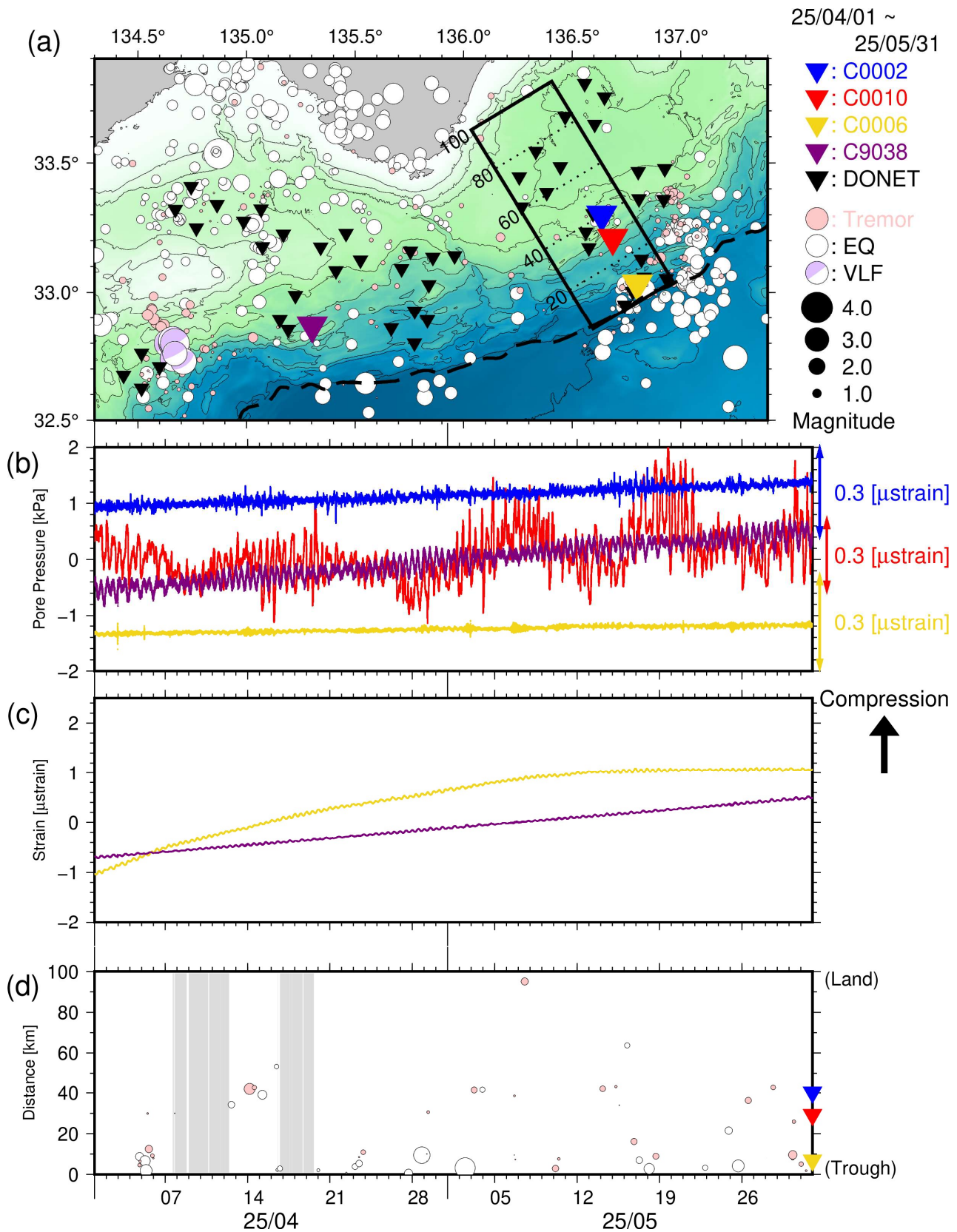
図3 直近2ヶ月間のSSE・低周波微動モニタリング(2025年4月1日~2025年5月31日)。(a)震央分布図(●:低周波微動(深さ0~15km)、○:通常地震(深さ0~60km)、●:超低周波地震のメカニズム解)。▼、▼、▼、▼、▼は、それぞれC0002・C0010・C0006・C9038・DONET観測点。破線はトラフ軸。(b)長期孔内観測点における間隙水圧変化(—:C0002、—:C0010、—:C0006、—:C9038)。(c)長期孔内観測点における体積歪計(—:C0010、—:C0006)および光ファイバ歪計(—:C9038)の変化。(d)図3a中に実線で示した矩形領域内における、低周波微動・通常地震・超低周波地震の時空間分布。縦軸は、トラフ軸からの距離(km)。
