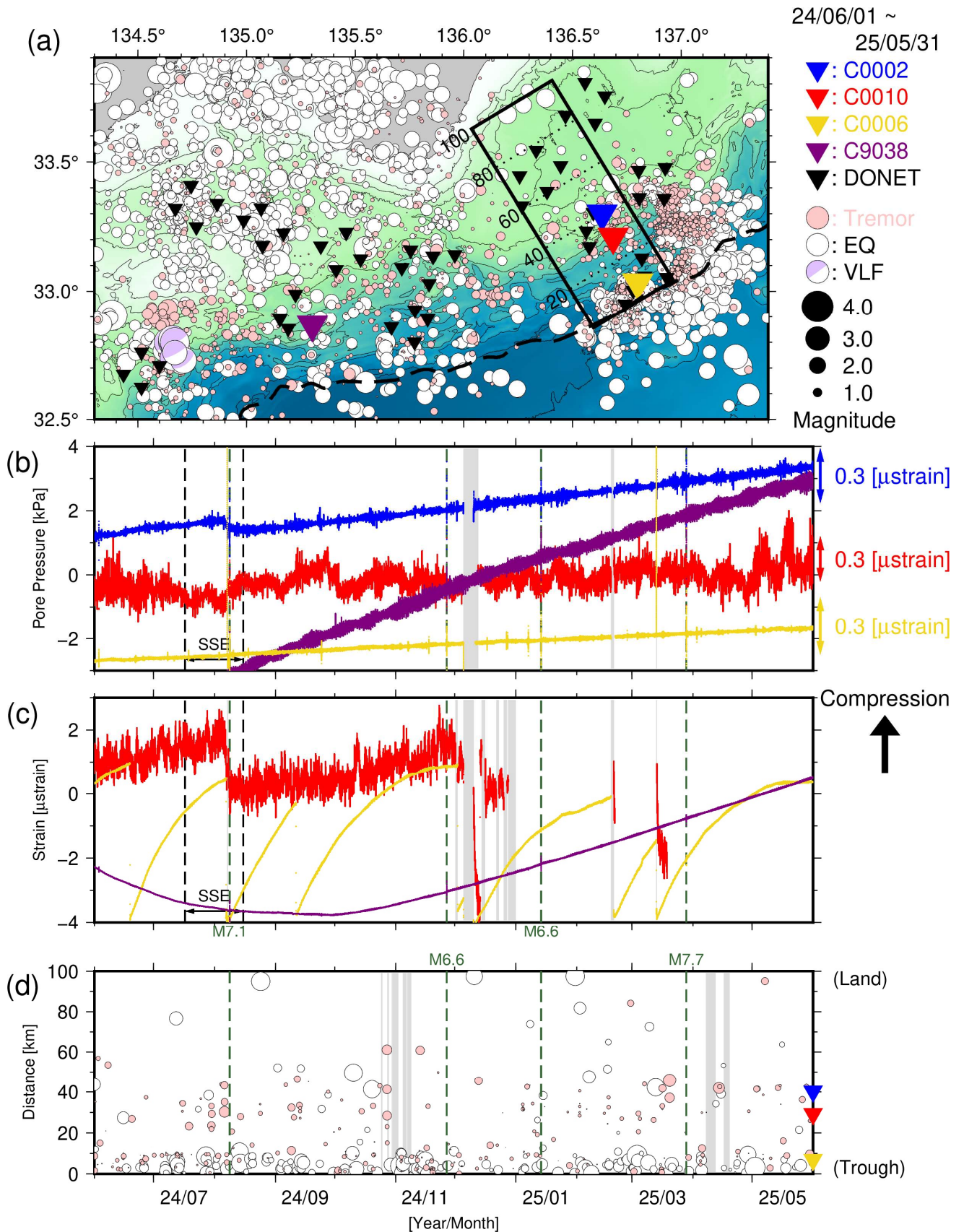
図4 直近1年間のSSE・低周波微動モニタリング(2024年6月1日~2025年5月31日)。(a)低周波微動・通常地震・超低周波地震の震央分布。(b)間隙水圧変化。(c)体積歪変化。(d)時空間分布。灰色は、エアガン発振期間あるいは停止期間のため、モニタリング対象外。緑点線は、日向灘の地震(8月8日M7.1、2025年1月13日M6.6)、能登地方の地震(11月26日M6.6)、およびミャンマー地震(3月28日M7.7)。なお、過去資料の図3に緑点線で記した地震のうち、aの領域外かつM6.5未満のものは掲載していない。
