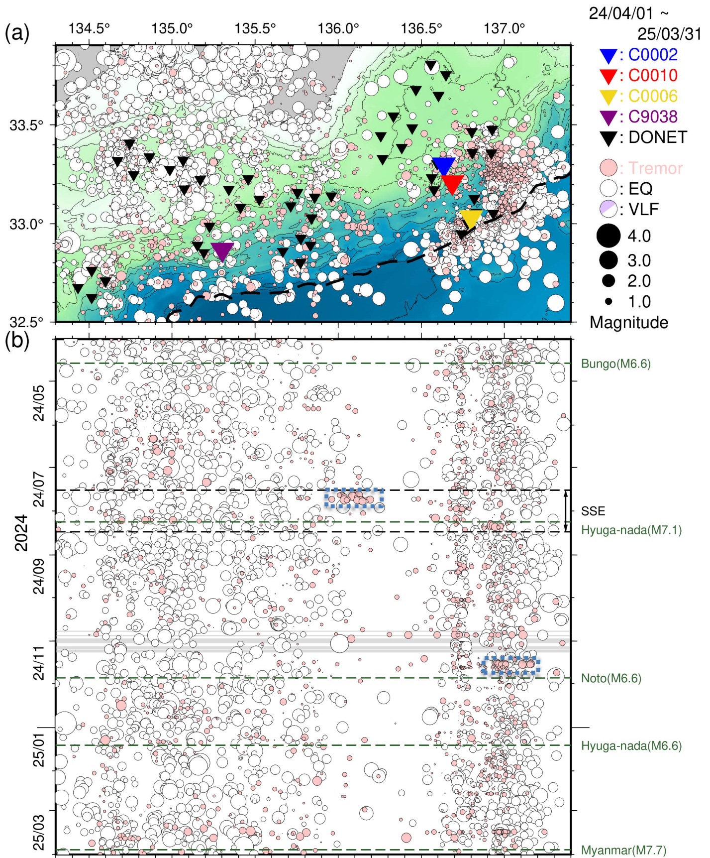
図 6 直近 1 年間に於いて熊野灘から室戸沖にて発生した低周波微動・通常地震・超低周波地震 (2024 年 4 月 1 日~2025 年 3 月 31 日)。図 4 と同様のシンボルにて表示。(a) 震央分布図。(b) a に示した震央を経度方向へ投影した時空間分布図。青点線の長方形領域は、これまでの評価文において言及した微動活動を示す。なお、過去資料の図 3 及び図 5 に緑点線で記した地震のうち、a の領域外かつ M6.5 未満のものは掲載していない。
