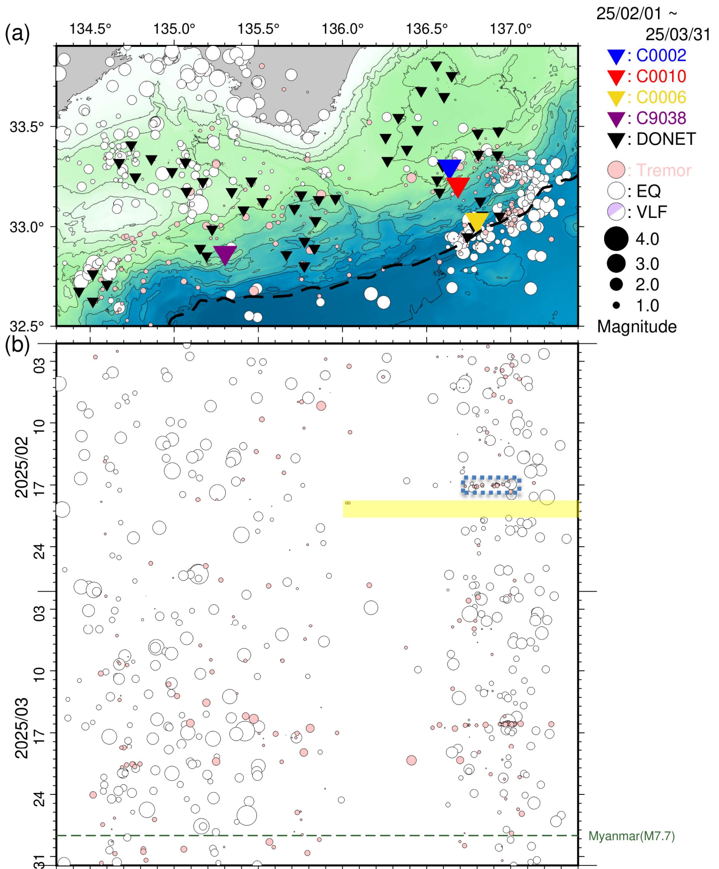
図5 直近2ヵ月間において熊野灘から室戸沖にて発生した低周波微動・通常地震・超低周波地震（2025年2月1日～2025年3月31日）。図3と同様のシンボルにて表示。(a) 震央分布図。(b) aに示した震央を経度方向へ投影した時空間分布図。青点線の長方形領域は、2月16日～2月17日頃にかけて発生した微動活動を示す。
