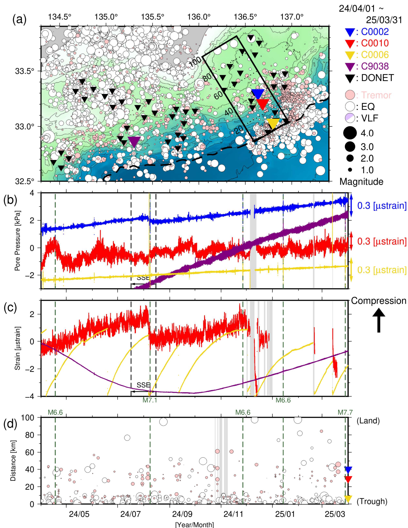
図4 直近1年間のSSE・低周波微動モニタリング（2024年4月1日～2025年3月31日）。(a) 低周波微動・通常地震・超低周波地震の震央分布。(b) 間隙水圧変化。(c) 体積歪変化。(d) 時空間分布。灰色は、エアガン発振期間あるいは停止期間のため、モニタリング対象外。緑点線は、豊後水道の地震（2024年4月17日M6.6）、日向灘の地震（8月8日M7.1、2025年1月13日M6.6）、能登地方の地震（11月26日M6.6）、およびミャンマー地震（3月28日M7.7）。なお、過去資料の図3に緑点線で記した地震のうち、aの領域外かつM6.5未満のものは掲載していない。
