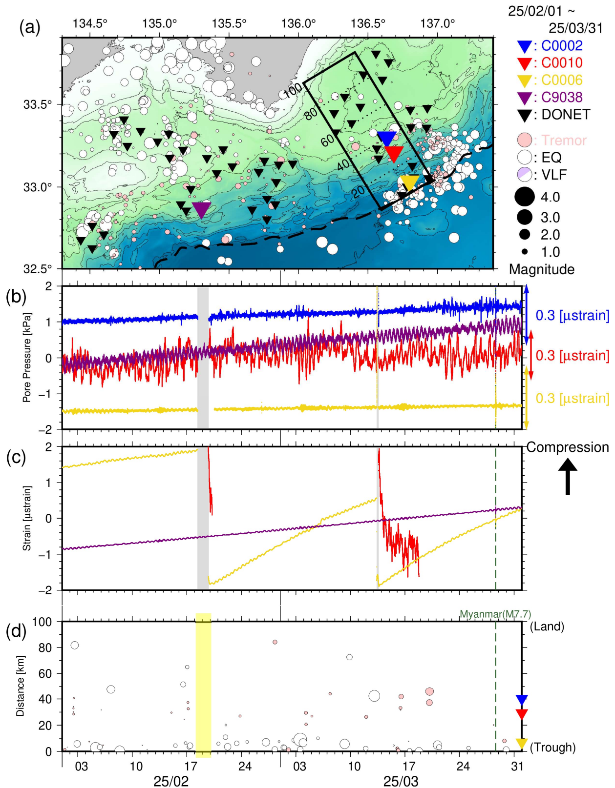
図3 直近2ヶ月間のSSE・低周波微動モニタリング(2025年2月1日~2025年3月31日)。(a) 震央分布図(●:低周波微動(深さ0~15km)、○:通常地震(深さ0~60km)、●:超低周波地震のメカニズム解)。▼は、それぞれC0002・C0010・C0006・C9038・DONET観測点。破線はトラフ軸。(b)長期孔内観測点における間隙水圧変化(—:C0002、—:C0010、—:C0006、—:C9038)。(c)長期孔内観測点における体積歪計(—:C0010、—:C0006)および光ファイバ歪計(—:C9038)の変化。(d)図3a中に実線で示した矩形領域内における、低周波微動・通常地震・超低周波地震の時空間分布。縦軸は、トラフ軸からの距離(km)。黄色背景は、DONET1休止期間(2025年2月18日~20日)のため、間隙圧の欠測・地震の検知能力低下が生じている。
