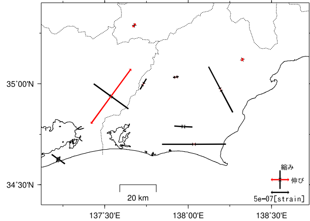
基準日: 2024/03/03 比較日: 2024/06/01
