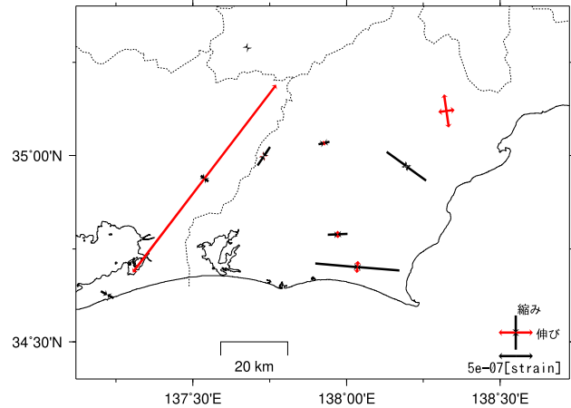
基準日: 2024/12/30 比較日: 2025/03/30
