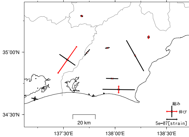
基準日: 2024/06/03 比較日: 2024/09/01
