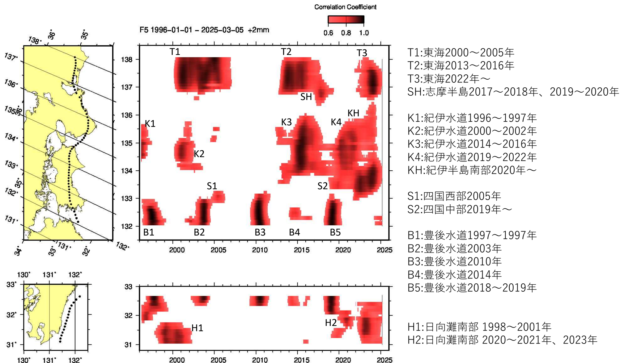
第1図 長期的スロースリップ客観検知図（1996年～2025年3月）
