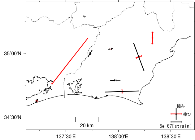
基準日: 2024/09/02 比較日: 2024/12/01
