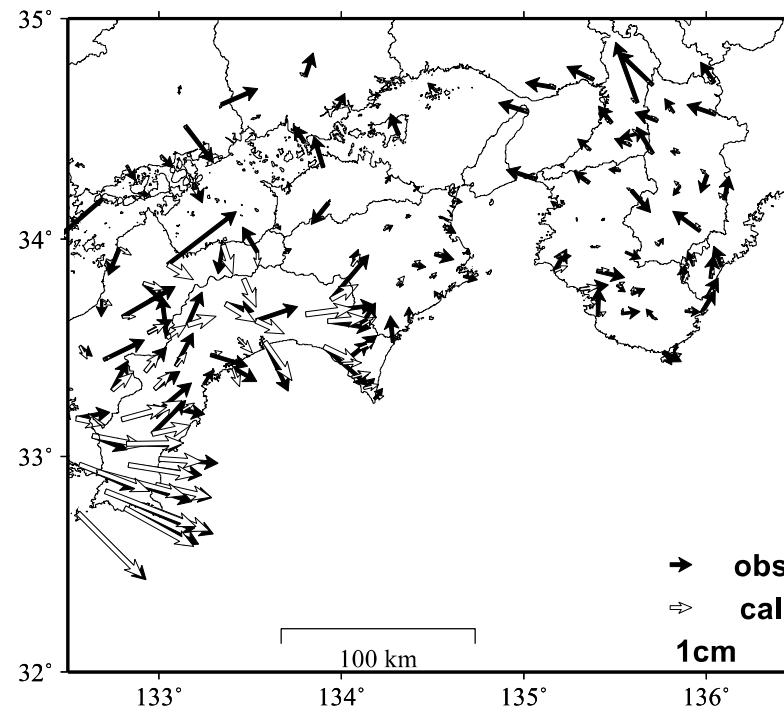
観測値（黒）と計算値（白）の比較 (2019-01-01/2025-03-07)
