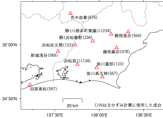
基準日: 2023/12/02 比較日: 2024/03/01
