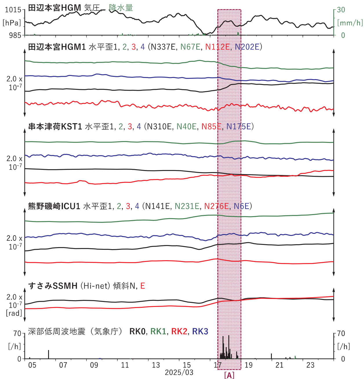
図2 紀伊半島における歪・傾斜の時間変化 (2025/03/05 00:00 - 2025/03/25 00:00 (JST))
