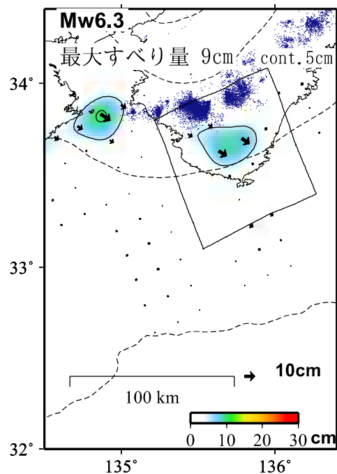
推定すべり分布 (2020-01-01/2025-03-09)
