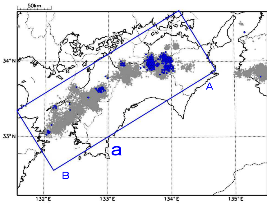
震央分布図（2019年3月1日～2025年4月1日、 深さ0～60km、Mすべて） 灰：2019年3月1日～2025年3月23日、 青：2025年3月24日以降
