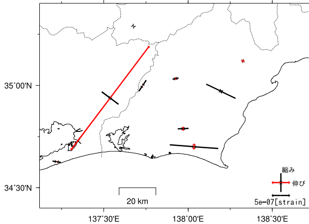
基準日: 2024/12/01 比較日: 2025/03/01
