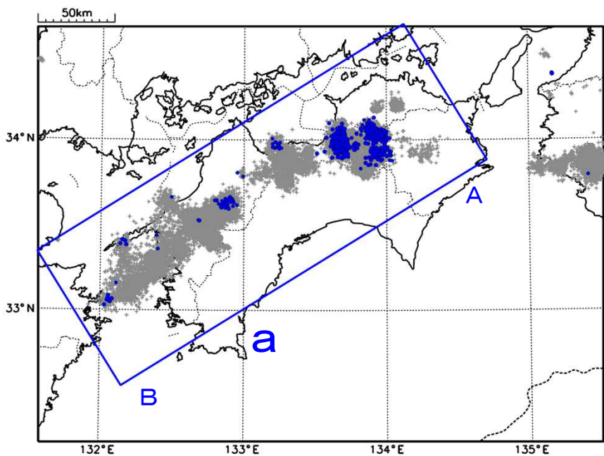
震央分布図（2019年3月1日～2025年4月1日、 深さ0～60km、Mすべて） 灰：2019年3月1日～2025年3月23日、 青：2025年3月24日以降
