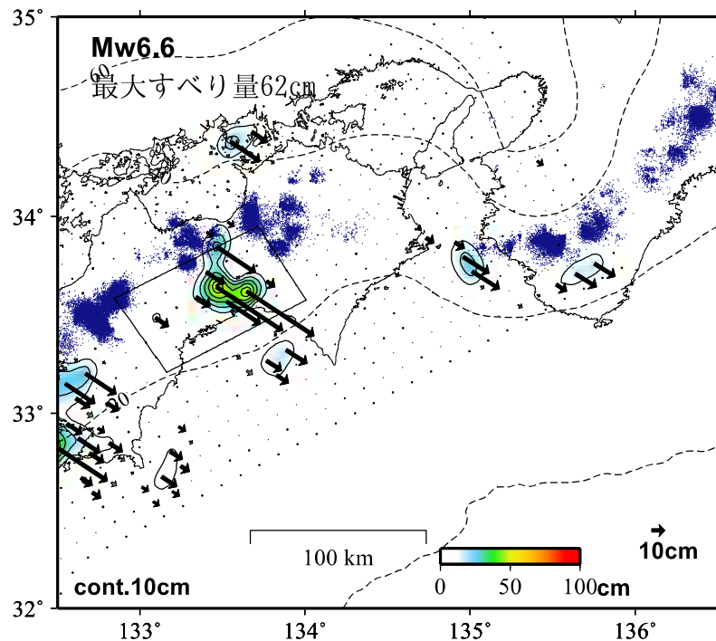
推定すべり分布 (2019-01-01/2025-03-07)
