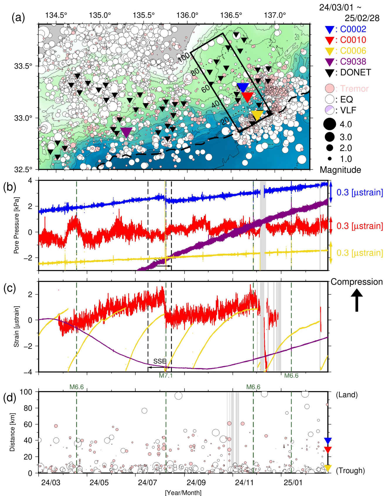
図4 直近1年間のSSE・低周波微動モニタリング（2024年3月1日～2025年2月28日）。（a）低周波微動・通常地震・超低周波地震の震央分布。（b）間隙水圧変化。（c）体積歪変化。（d）時空間分布。灰色は、エアガン発振期間あるいは停電期間のため、モニタリング対象外。緑点線は、豊後水道の地震（2024年4月17日 M6.6）、日向灘の地震（8月8日 M7.1、2025年1月13日 M6.6）、および能登地方の地震（11月26日 M6.6）。なお、過去資料の図3に緑点線で記した地震のうち、aの領域外かつ M6.5 未満のものは掲載していない。
