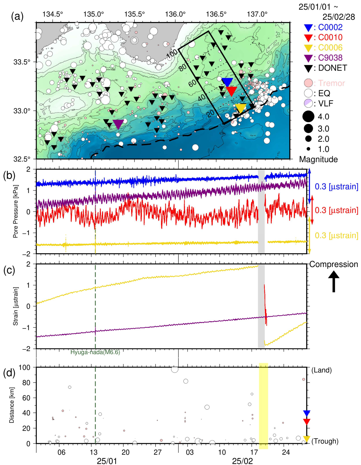
図3 直近2ヶ月間のSSE・低周波微動モニタリング(2025年1月1日~2025年2月28日)。(a) 震央分布図(●:低周波微動(深さ0~15km)、○:通常地震(深さ0~60km)、●:超低周波地震のメカニズム解)。▼▼▼▼▼は、それぞれC0002・C0010・C0006・C9038・DONET観測点。破線はトラフ軸。(b)長期孔内観測点における間隙水圧変化(—:C0002、—:C0010、—:C0006、—:C9038)。(c)長期孔内観測点における体積歪計(—:C0010、—:C0006)および光ファイバ歪計(—:C9038)の変化。(d)図3a中に実線で示した矩形領域内における、低周波微動・通常地震・超低周波地震の時空間分布。縦軸は、トラフ軸からの距離(km)。黄色背景は、DONET1休止期間(2025年2月18日~20日)のため、間隙圧の欠測・地震の検知能力低下が生じている。
