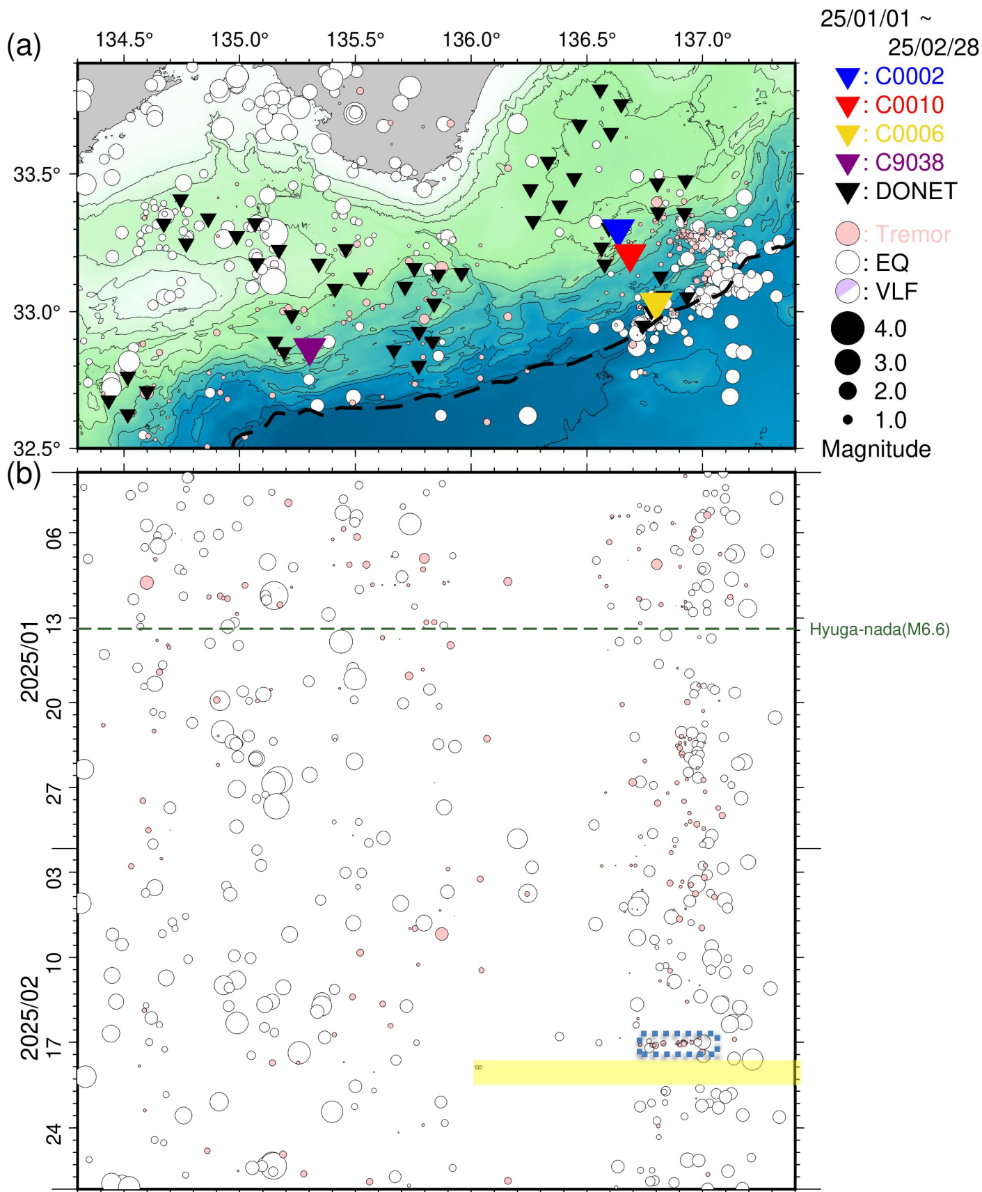
図5 直近2ヵ月間において熊野灘から室戸沖にて発生した低周波微動・通常地震・超低周波地震 (2025年1月1日～2025年2月28日)。図3と同様のシンボルにて表示。(a) 震央分布図。(b) aに示した震央を経度方向へ投影した時空間分布図。青点線の長方形領域は、2月16日～2月17日頃にかけて発生した微動活動を示す。
