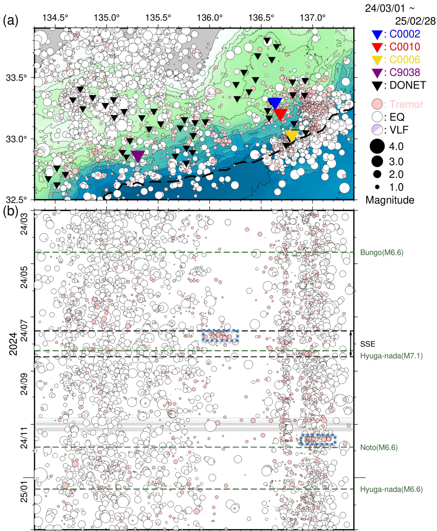
図 6 直近 1 年間に於いて熊野灘から室戸沖にて発生した低周波微動・通常地震・超低周波地震 (2024 年 3 月 1 日~2025 年 2 月 28 日)。図 4 と同様のシンボルにて表示。(a) 震央分布図。(b) a に示した震央を経度方向へ投影した時空間分布図。青点線の長方形領域は、これまでの評価文において言及した微動活動を示す。なお、過去資料の図 3 及び図 5 に緑点線で記した地震のうち、a の領域外かつ M6.5 未満のものは掲載していない。
