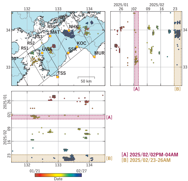
図1 四国地方における深部低周波地震の時空間分布図。 (2025/01/21 00:00 - 2025/02/27 00:00 (JST)) 気象庁カタログによる。
