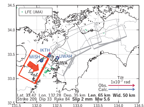
図4 2025/02/02PM - 04AM の歪・傾斜変化 (図2 [A]) を説明する断層モデル。
