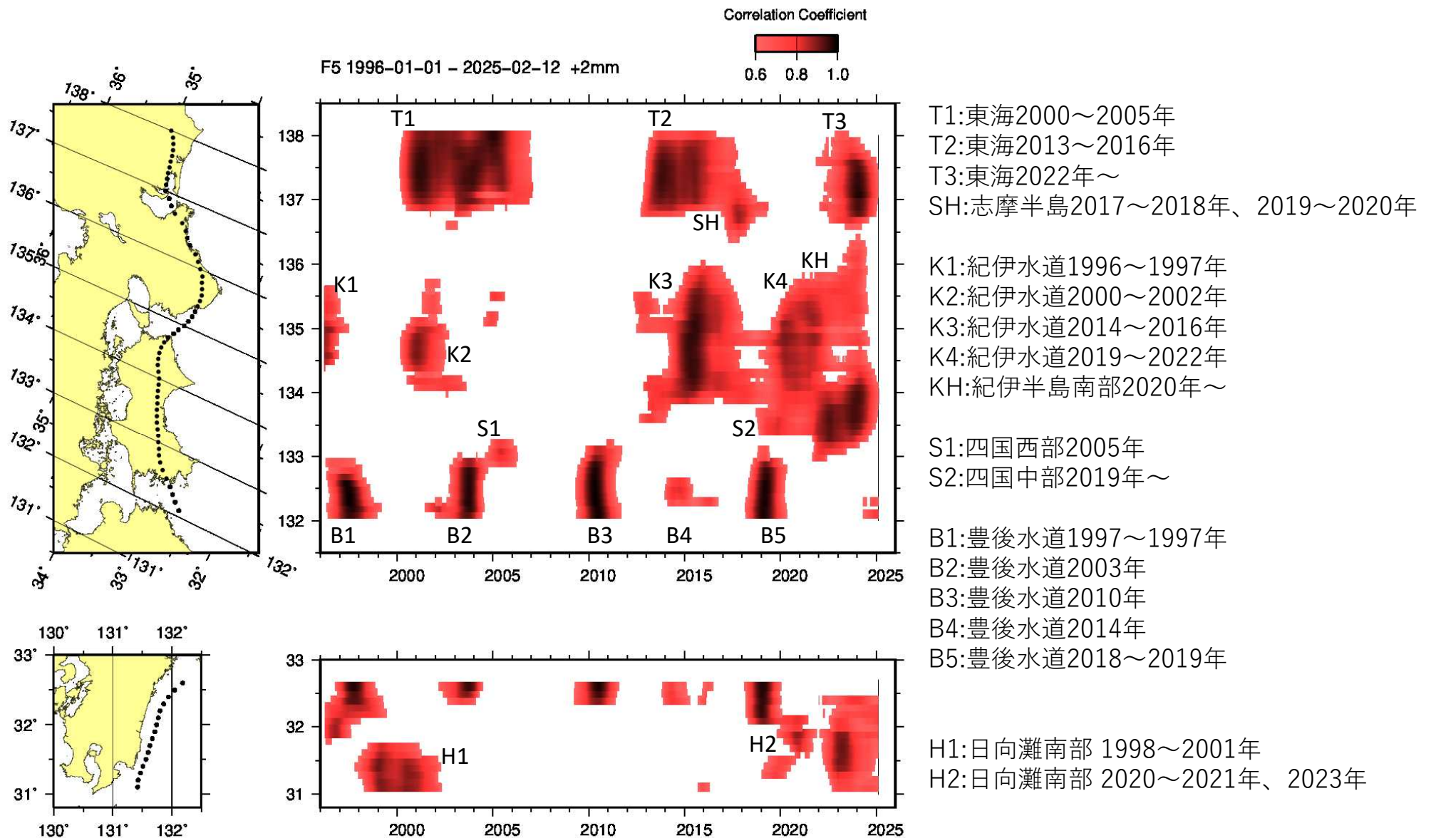
第1図 長期的スロースリップ客観検知図（1996年～2025年2月）
