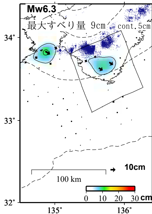
推定すべり分布 (2020-01-01/2025-02-13)
