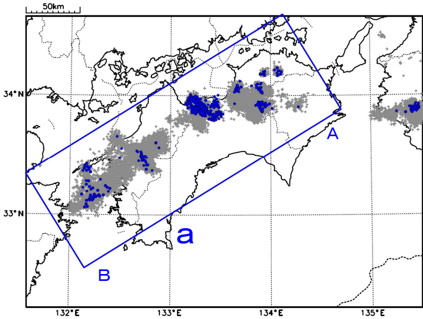
震央分布図（2019年2月1日～2025年2月25日、 深さ0～60km、Mすべて） 灰：2019年2月1日～2025年1月31日、 青：2025年2月1日以降
