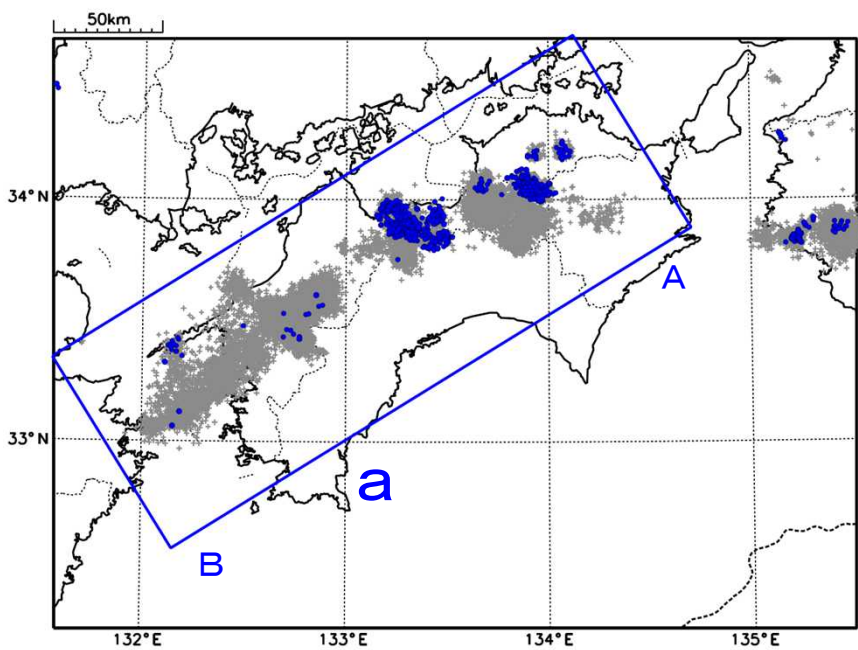
震央分布図（2019年2月1日～2025年3月3日、 深さ0～60km、Mすべて） 灰：2019年2月1日～2025年2月19日、 青：2025年2月20日以降
