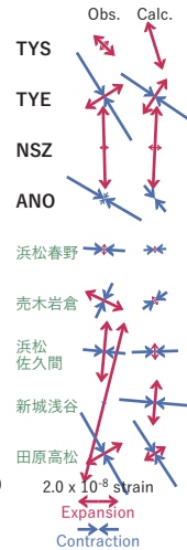
図7 2025/01/25PM-27AMの歪・傾斜・地下水位変化(図5[B])を説明する断層モデル。
