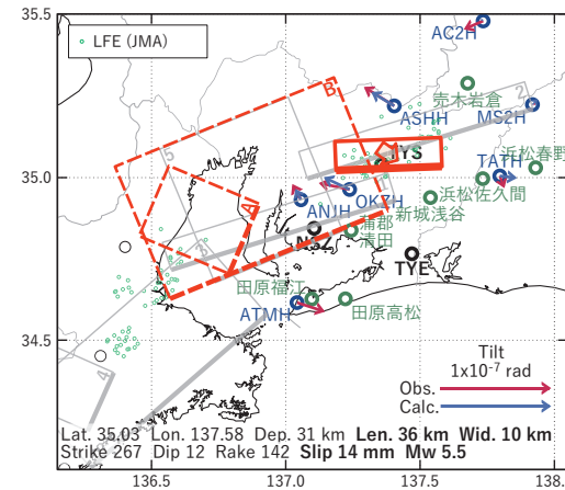
図8 2025/01/27PM-28の歪・傾斜変化(図5[C])を説明する断層モデル。
