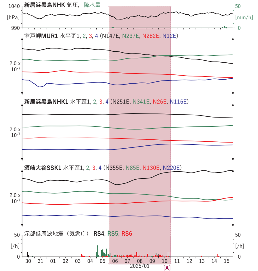
図10 歪・傾斜の時間変化(1)（2024/12/30 00:00-2025/01/16 00:00 (JST)）
