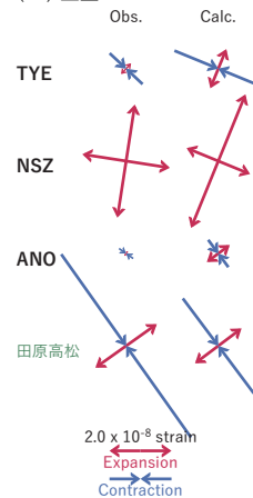
図3 2025/01/12-17の歪・傾斜変化(図2[A])を説明する断層モデル。
