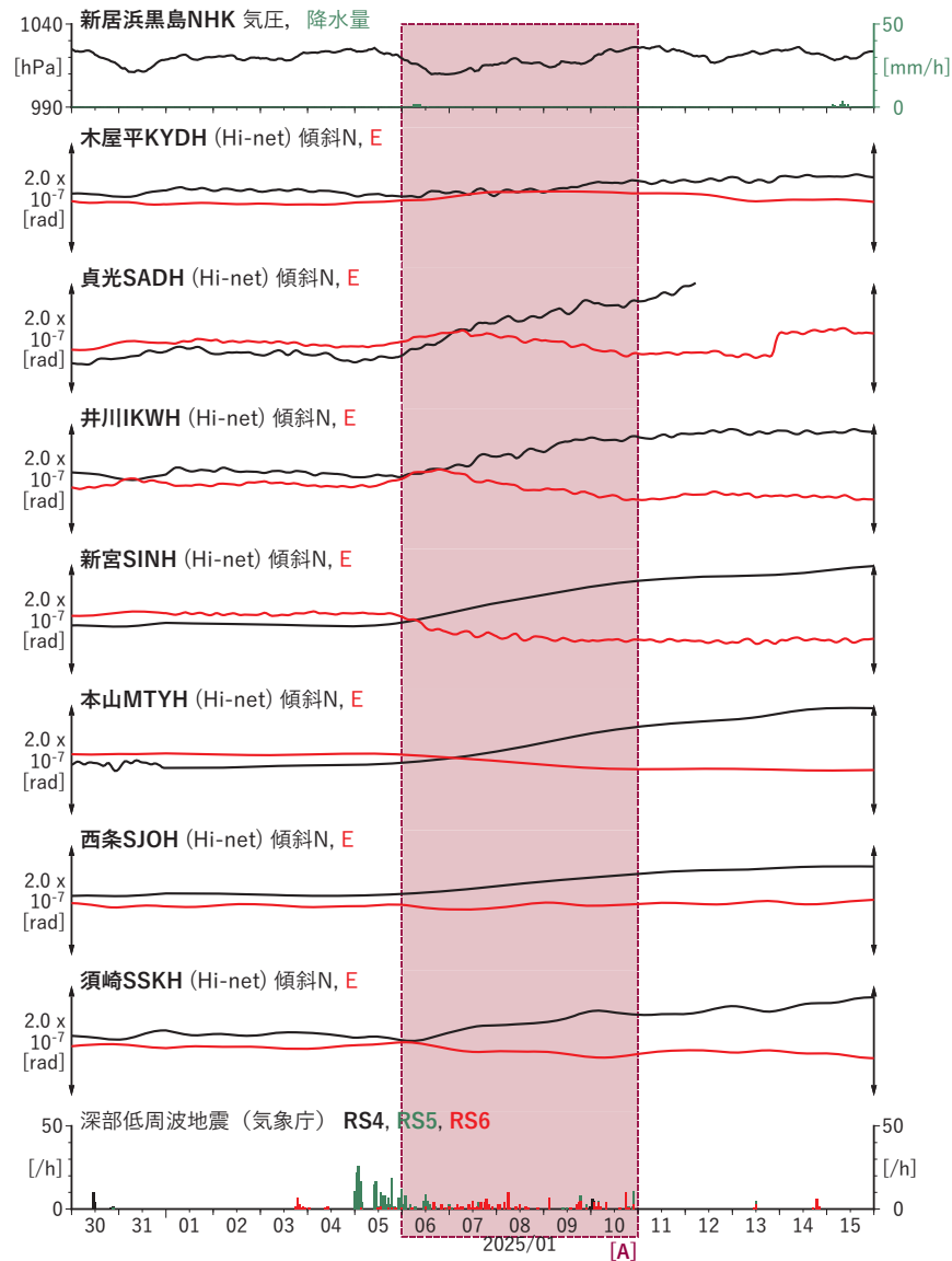
図10 歪・傾斜の時間変化(2) (2024/12/30 00:00-2025/01/16 00:00 (JST))
