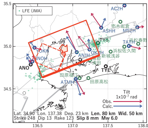
図7 2025/01/25PM-27AMの歪・傾斜・地下水位変化(図5[B])を説明する断層モデル。
