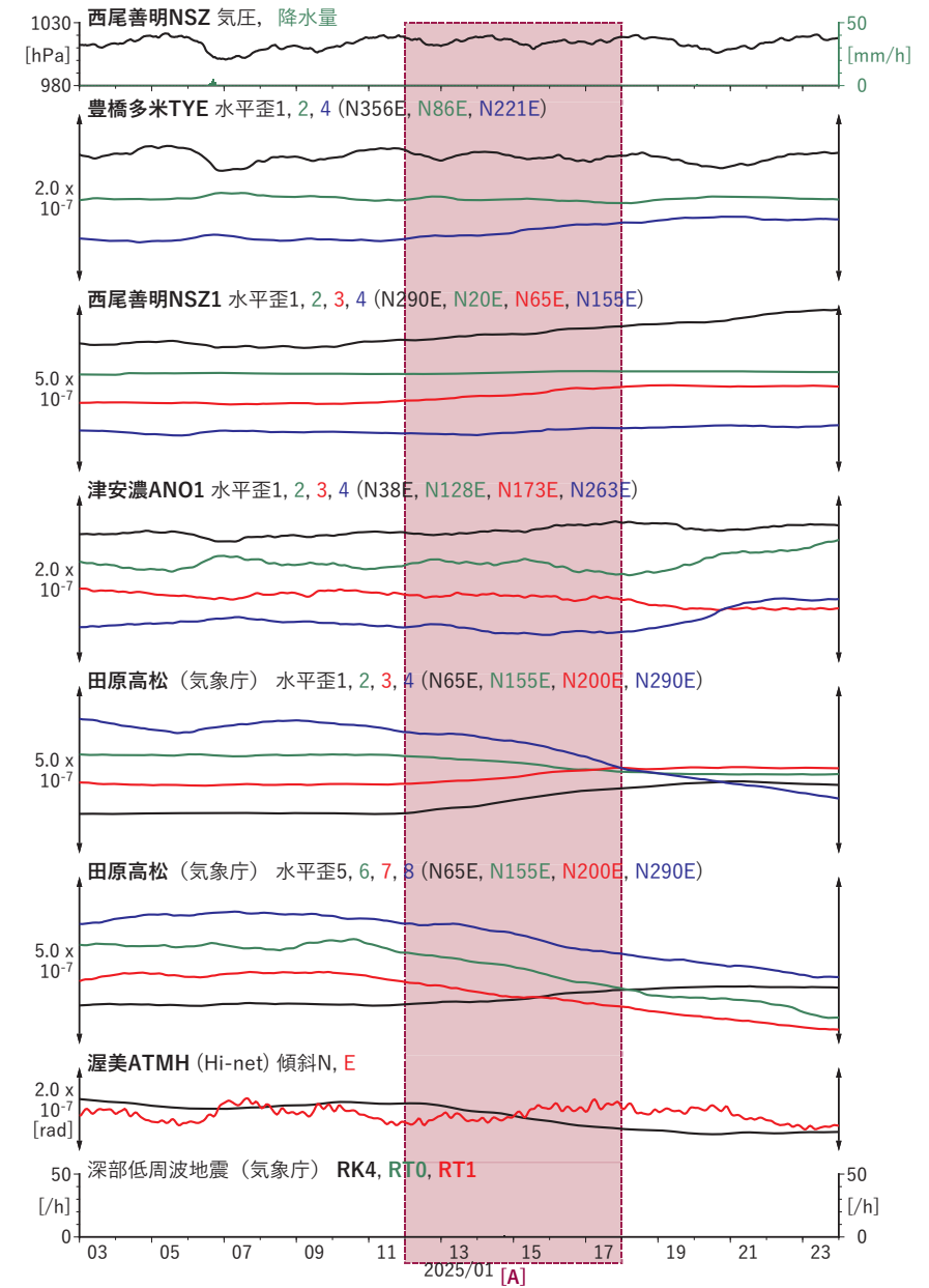
図2 歪・傾斜の時間変化（2025/01/03 00:00-2025/01/24 00:00 (JST)）
