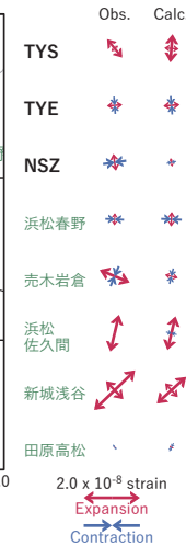
図8 2025/01/27PM-28の歪・傾斜変化(図5[C])を説明する断層モデル。
