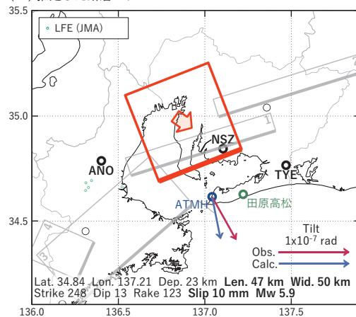
図3 2025/01/12-17の歪・傾斜変化(図2[A])を説明する断層モデル。
