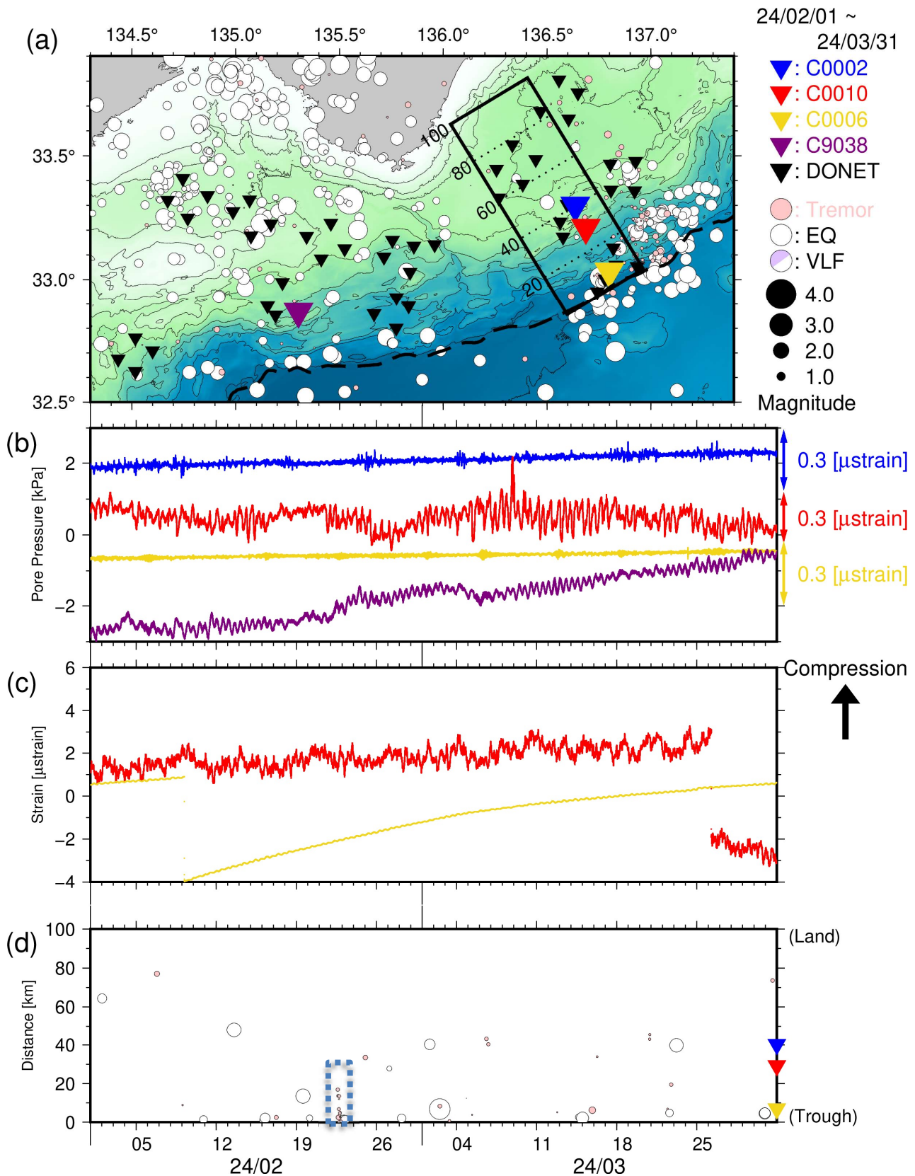
図3 直近2ヶ月間のSSE・低周波微動モニタリング(2024年2月1日~2024年3月31日)。(a)震央分布図(●:低周波微動(深さ0~15km)、○:通常地震(深さ0~60km)、●:超低周波地震のメカニズム解)。▼、▼、▼、▼、▼は、それぞれC0002・C0010・C0006・C9038・DONET観測点。破線はトラフ軸。(b)長期孔内観測点における間隙水圧変化(—:C0002、—:C0010、—:C0006、—:C9038)。(c)長期孔内観測点における体積歪変化(—:C0010、—:C0006)。(d)図3a中に実線で示した矩形領域内における、低周波微動・通常地震・超低周波地震の時空間分布。縦軸は、トラフ軸からの距離(km)。
