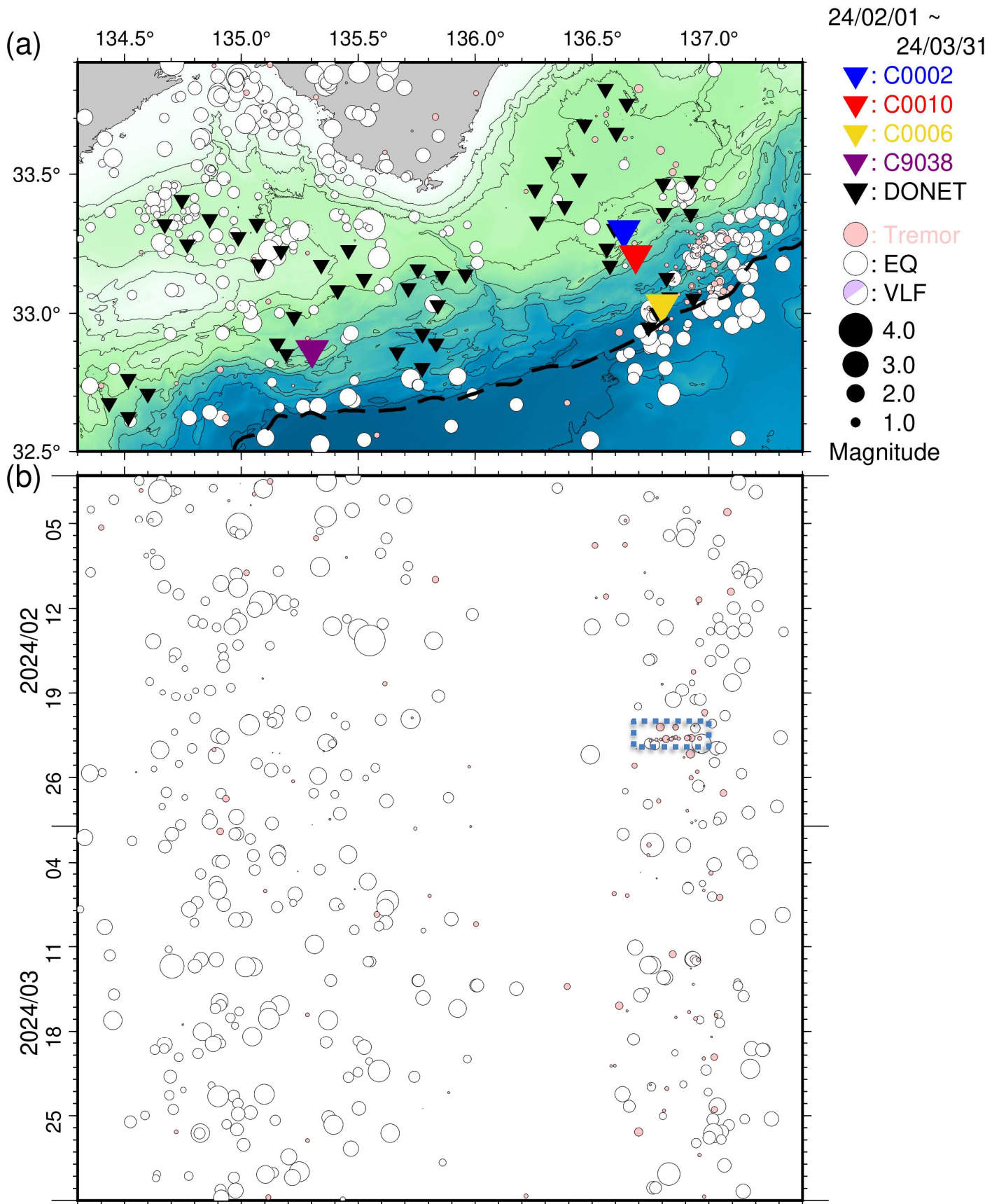
図5 直近2ヵ月間において熊野灘から室戸沖にて発生した低周波微動・通常地震・超低周波地震(2024年2月1日~2024年3月31日)。図3と同様のシンボルにて表示。(a)震央分布図。(b)aに示した震央を経度方向へ投影した時空間分布図。青点線枠内は、DONET1のCノード付近における低周波微動の群発的な小規模活動を示す(図3も同様)。
