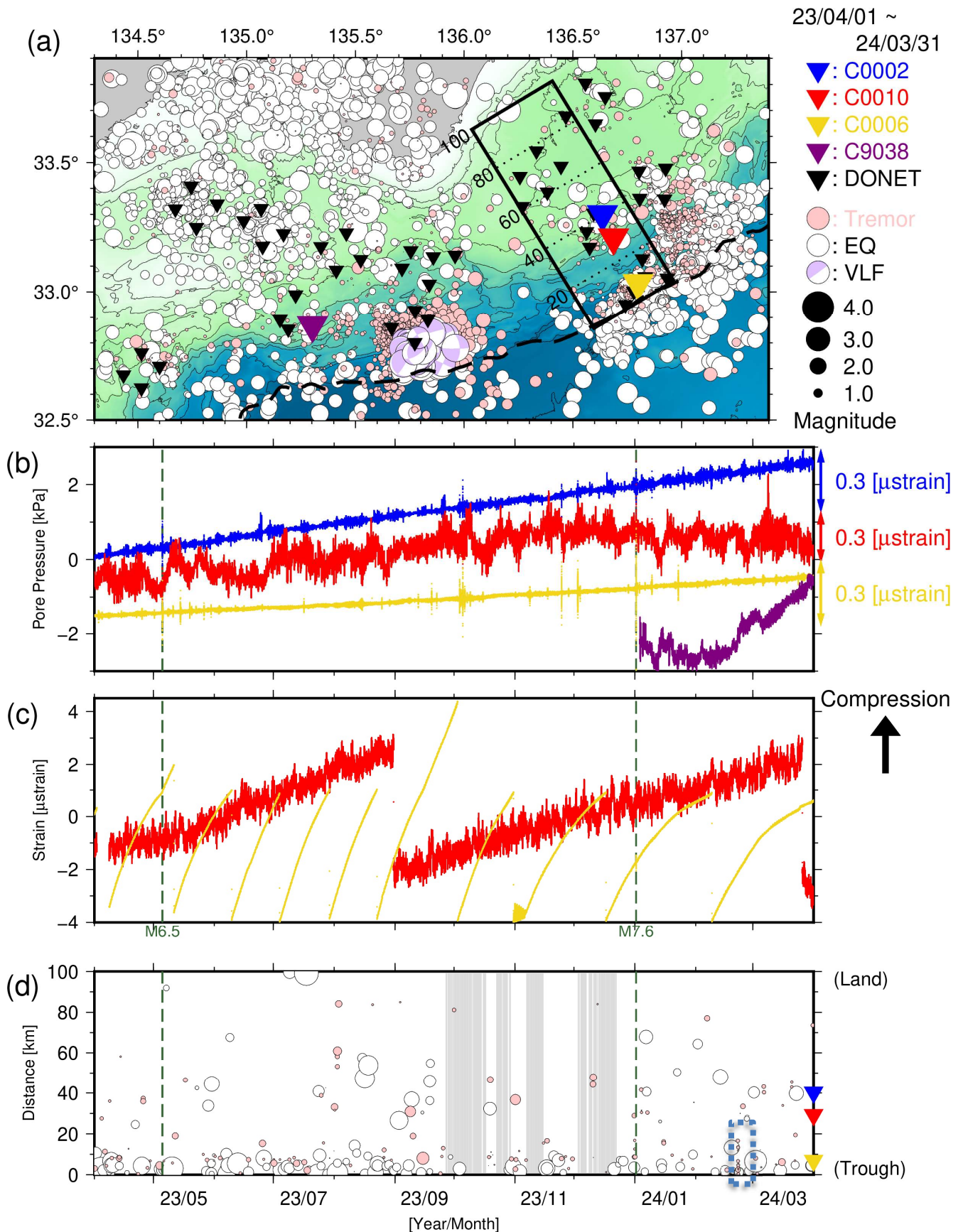
図4 直近1年間のSSE・低周波微動モニタリング(2023年4月1日~2024年3月31日)。(a)低周波微動・通常地震・超低周波地震の震央分布。(b)間隙水圧変化。(c)体積歪変化。(d)時空間分布。灰色はエアガン発振期間。緑点線は、能登地方の地震(2023年5月5日M6.5と2024年1月1日M7.6)。なお、過去資料の図3に緑点線で記した地震のうち、aの領域外かつM6.5未満のものは掲載していない。
