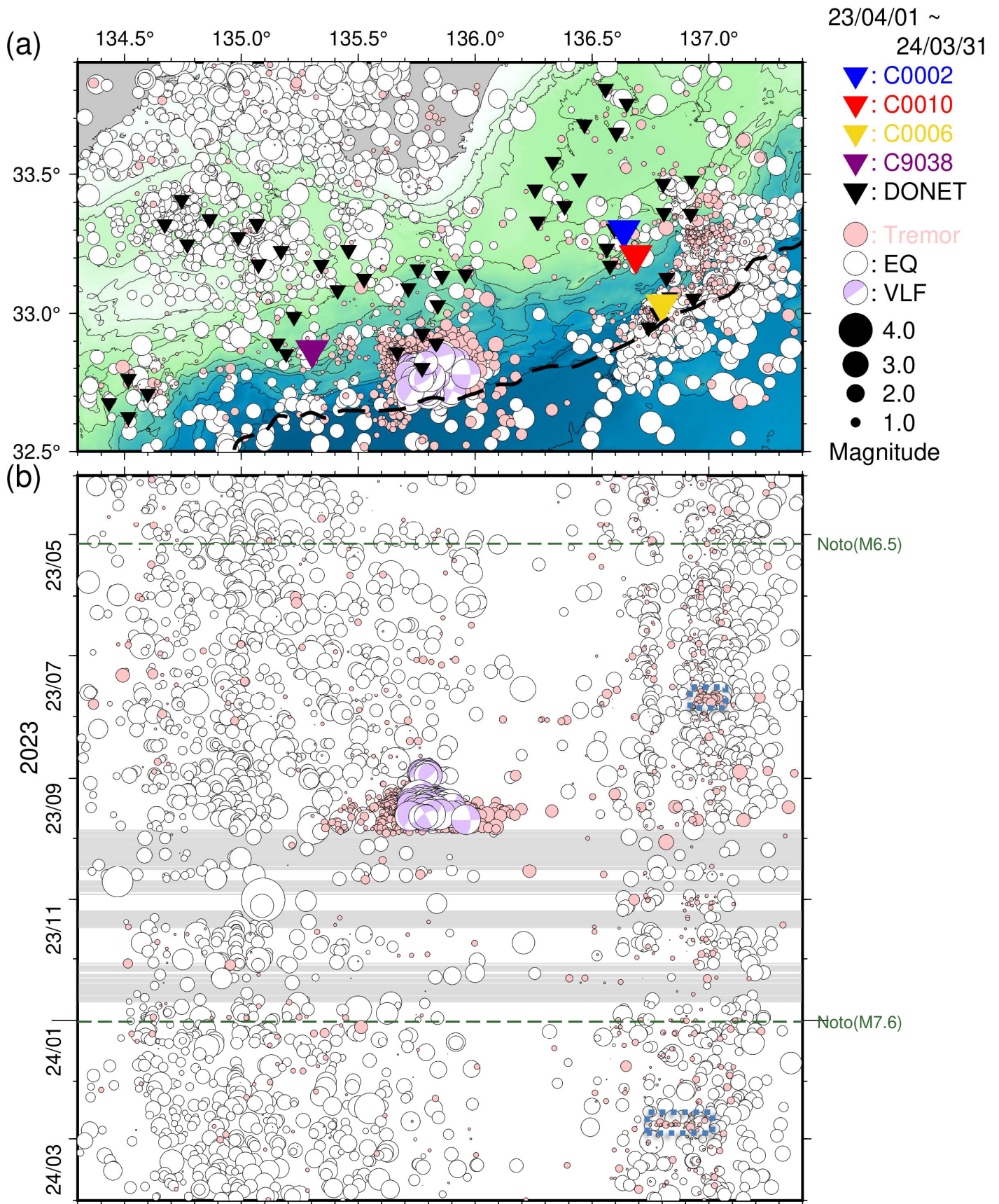
図 6 直近 1 年間に於いて熊野灘から室戸沖にて発生した低周波微動・通常地震・超低周波地震 (2023 年 4 月 1 日~2024 年 3 月 31 日)。図 4 と同様のシンボルにて表示。(a) 震央分布図。(b) a に示した震央を経度方向へ投影した時空間分布図。青点線の長方形領域は、DONET1 の B ノード及び C ノード付近における低周波微動の群発的な活動を示す。なお、過去資料の図 3 及び図 5 に緑点線で記した地震のうち、a の領域外かつ M6.5 未満のものは掲載していない。
