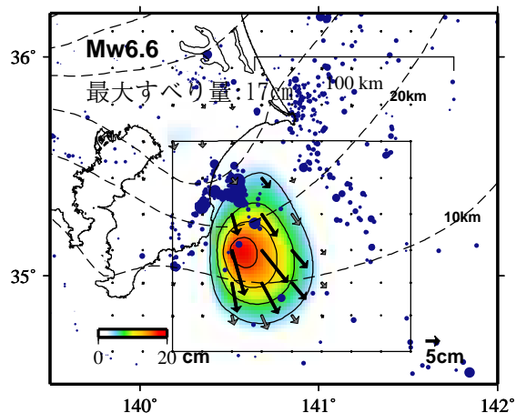
推定すべり分布 (2024-02-04/2024-03-30)
