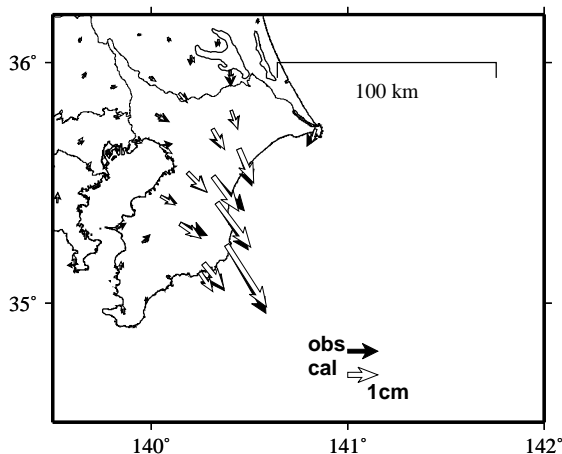
観測値（黒）と計算値（白）の比較 (2024-02-04/2024-03-30)
