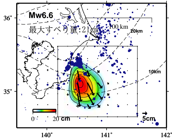
推定すべり分布 (2024-02-04/2024-03-17)
