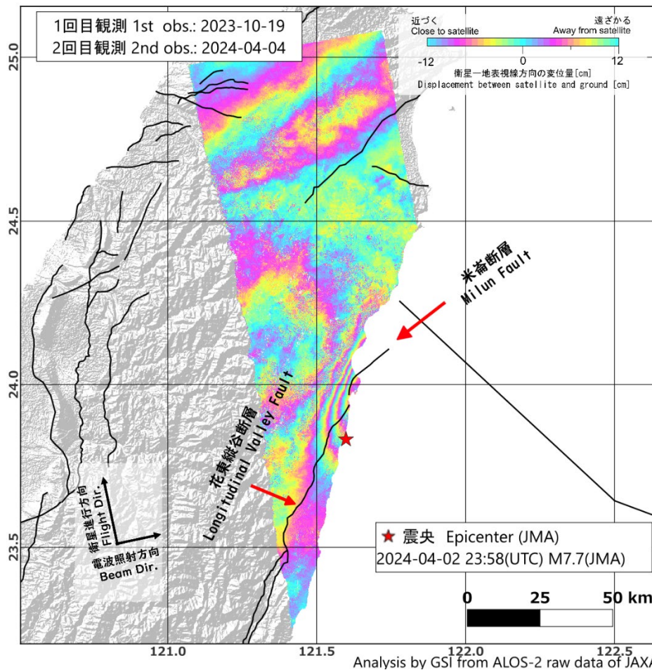
図1. SAR干渉解析結果。震央はJMAによる。断層線はStyron et al. (2020)より。
