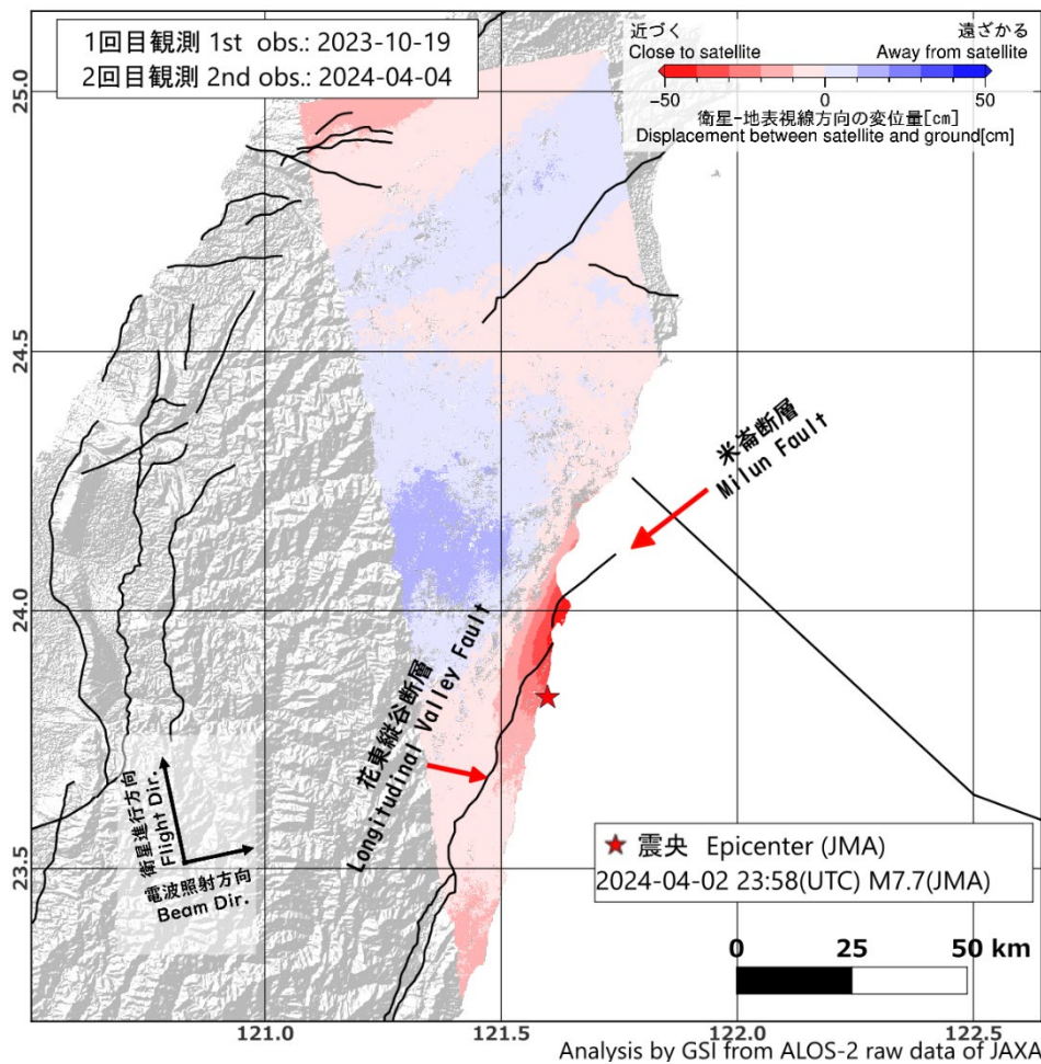
図2. SAR干渉解析結果(アンラップ済み)。震央はJMAによる。断層線はStyron et al. (2020)より。
