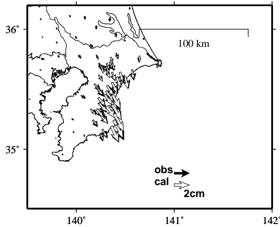
観測値（黒）と計算値（白）の比較 (2024-02-04/2024-03-17)
