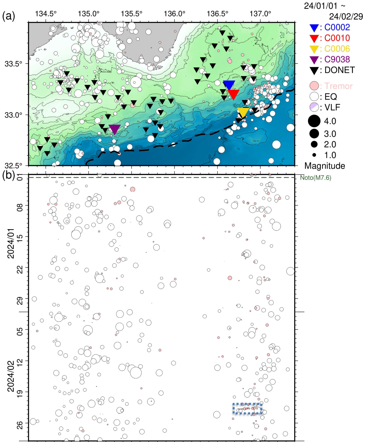
図5 直近2ヵ月間において熊野灘から室戸沖にて発生した低周波微動・通常地震・超低周波地震(2024年1月1日~2024年2月29日)。図3と同様のシンボルにて表示。(a)震央分布図。(b)aに示した震央を経度方向へ投影した時空間分布図。青点線枠内は、DONET1のCノード付近における低周波微動の群発的な小規模活動を示す(図3も同様)。
