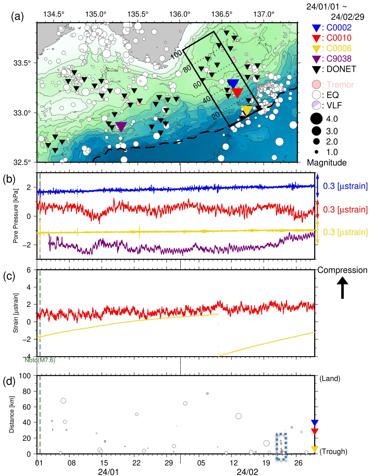
図3 直近2ヶ月間のSSE・低周波微動モニタリング(2024年1月1日~2024年2月29日)。(a)震央分布図(●:低周波微動(深さ0~15km)、○:通常地震(深さ0~60km)、●:超低周波地震のメカニズム解)。▼、▼、▼、▼、▼は、それぞれC0002・C0010・C0006・C9038・DONET観測点。破線はトラフ軸。(b)長期孔内観測点における間隙水圧変化(—:C0002、—:C0010、—:C0006、—:C9038)。(c)長期孔内観測点における体積歪変化(—:C0010、—:C0006)。(d)図3a中に実線で示した矩形領域内における、低周波微動・通常地震・超低周波地震の時空間分布。緑点線は、能登地方の地震(2024年1月1日M7.6)。縦軸は、トラフ軸からの距離(km)。
