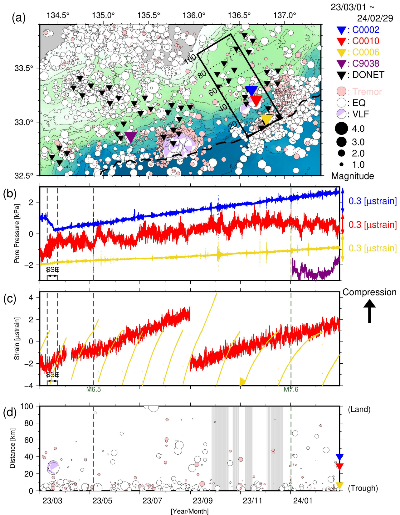
図4 直近1年間のSSE・低周波微動モニタリング(2023年3月1日~2024年2月29日)。(a)低周波微動・通常地震・超低周波地震の震央分布。(b)間隙水圧変化。(c)体積歪変化。(d)時空間分布。灰色はエアガン発振期間。緑点線は、能登地方の地震(2023年5月5日M6.5と2024年1月1日M7.6)。なお、過去資料の図3に緑点線で記した地震のうち、aの領域外かつM6.5未満のものは掲載していない。
