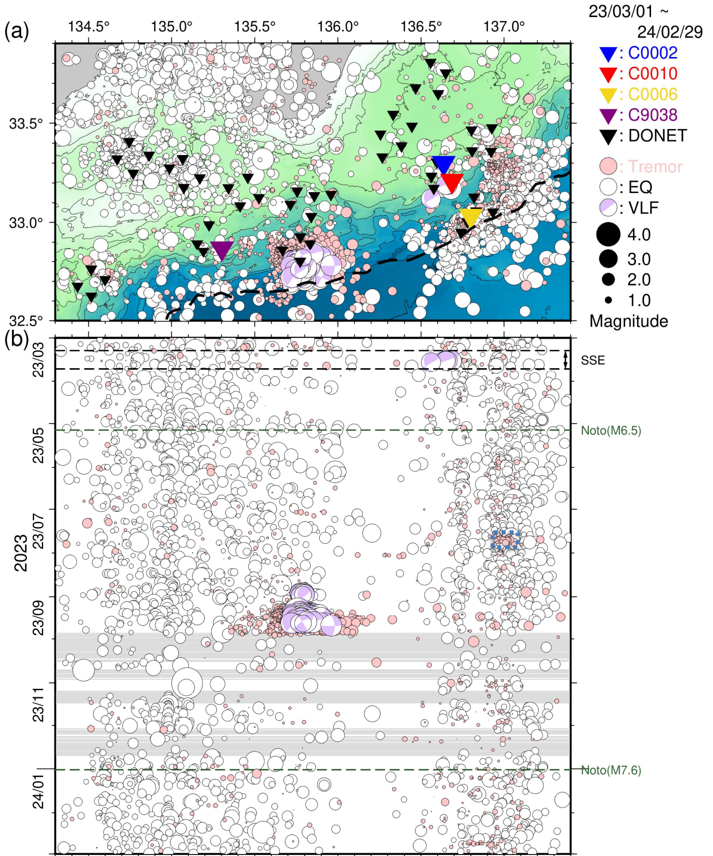
図 6 直近 1 年間に於いて熊野灘から室戸沖にて発生した低周波微動・通常地震・超低周波地震 (2023 年 3 月 1 日~2024 年 2 月 29 日)。図 4 と同様のシンボルにて表示。(a) 震央分布図。(b) a に示した震央を経度方向へ投影した時空間分布図。青点線の長方形領域は、DONET1 の B ノード付近における低周波微動の群発的な活動を示す。なお、過去資料の図 3 及び図 5 に緑点線で記した地震のうち、a の領域外かつ M6.5 未満のものは掲載していない。
