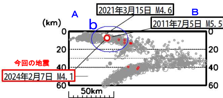
領域a内の断面図(A-B投影)
