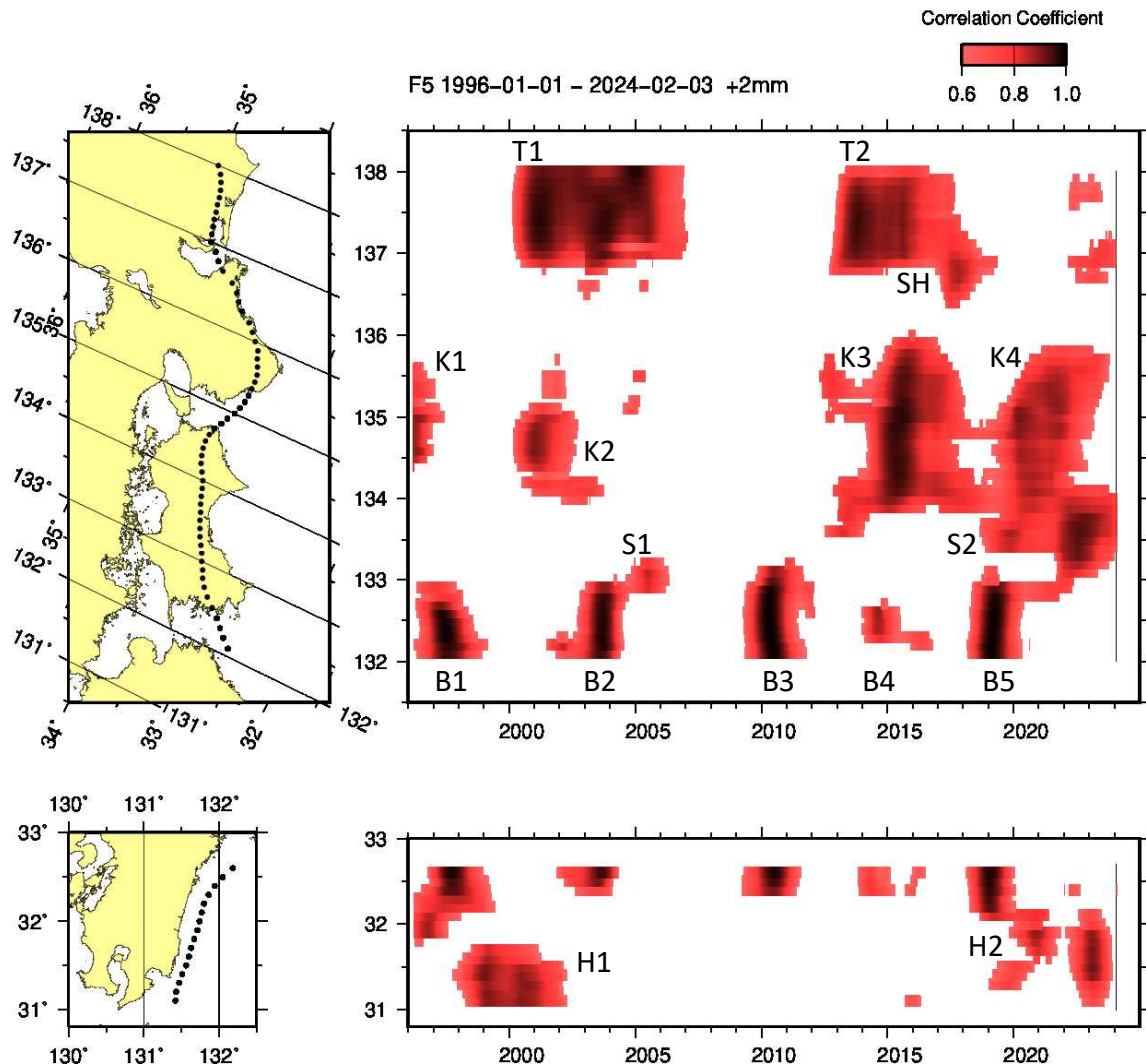
第1図 長期的スロースリップ客観検知図（1996年～2024年2月） スロースリップに伴う非定常変位の範囲（場所、時間）を赤～黒で示す。色が濃いほどスロースリップの発生可能性が高い。右端の縦線は最新データ日を示す。なお、これは変位が検出された範囲で、変動源自体の範囲ではない。
