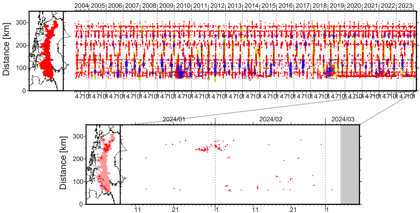
図1. 四国における2004年3月～2024年3月4日までの深部低周波微動の時空間分布(上図). 赤丸はエンベロップ相関・振幅ハイブリッド法 (Maeda and Obara, 2009) およびクラスタ処理 (Obara et al., 2010) によって1時間毎に自動処理された微動分布の重心である. 青菱形は周期20秒に卓越する超低周波地震 (Ito et al., 2007) である. 黄緑色太線は、これまでに検出された短期的スロースリップイベント (SSE) を示す. 下図は2024年2月を中心とした期間の拡大図である. 1月26日～2月5日頃には徳島県中部から愛媛県東部でやや活発な微動活動がみられた. 愛媛・香川・徳島県境付近で活動が開始した後、東方向への活動域の拡大がみられ、2月4日頃には愛媛県東部でも活動がみられた. これ以外の活動として、2月3日～5日頃および12日頃には、豊後水道において、それぞれ小規模およびごく小規模な活動がみられた. 2月17日頃および20～21日頃には愛媛県西部において、それぞれ小規模な活動がみられた.
