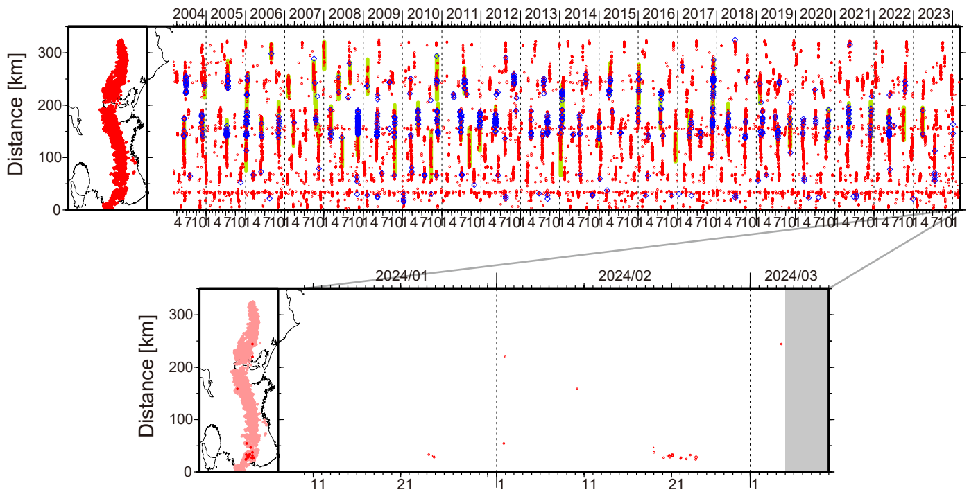
図1. 紀伊半島・東海地域における2004年3月～2024年3月4日までの深部低周波微動の時空間分布（上図）。赤丸はエンベロープ相関・振幅ハイブリッド法 (Maeda and Obara, 2009) およびクラスター処理 (Obara et al., 2010) によって1時間毎に自動処理された微動分布の重心である。青菱形は周期20秒に卓越する超低周波地震 (Ito et al., 2007) である。黄緑色の太線はこれまでに検出された短期的スロースリップイベント (SSE) を示す。下図は2024年2月を中心とした期間の拡大図である。2月以降の期間において、顕著な活動はみられなかったものの、2月20～23日頃に和歌山県中部において、小規模な微動活動がみられた。
