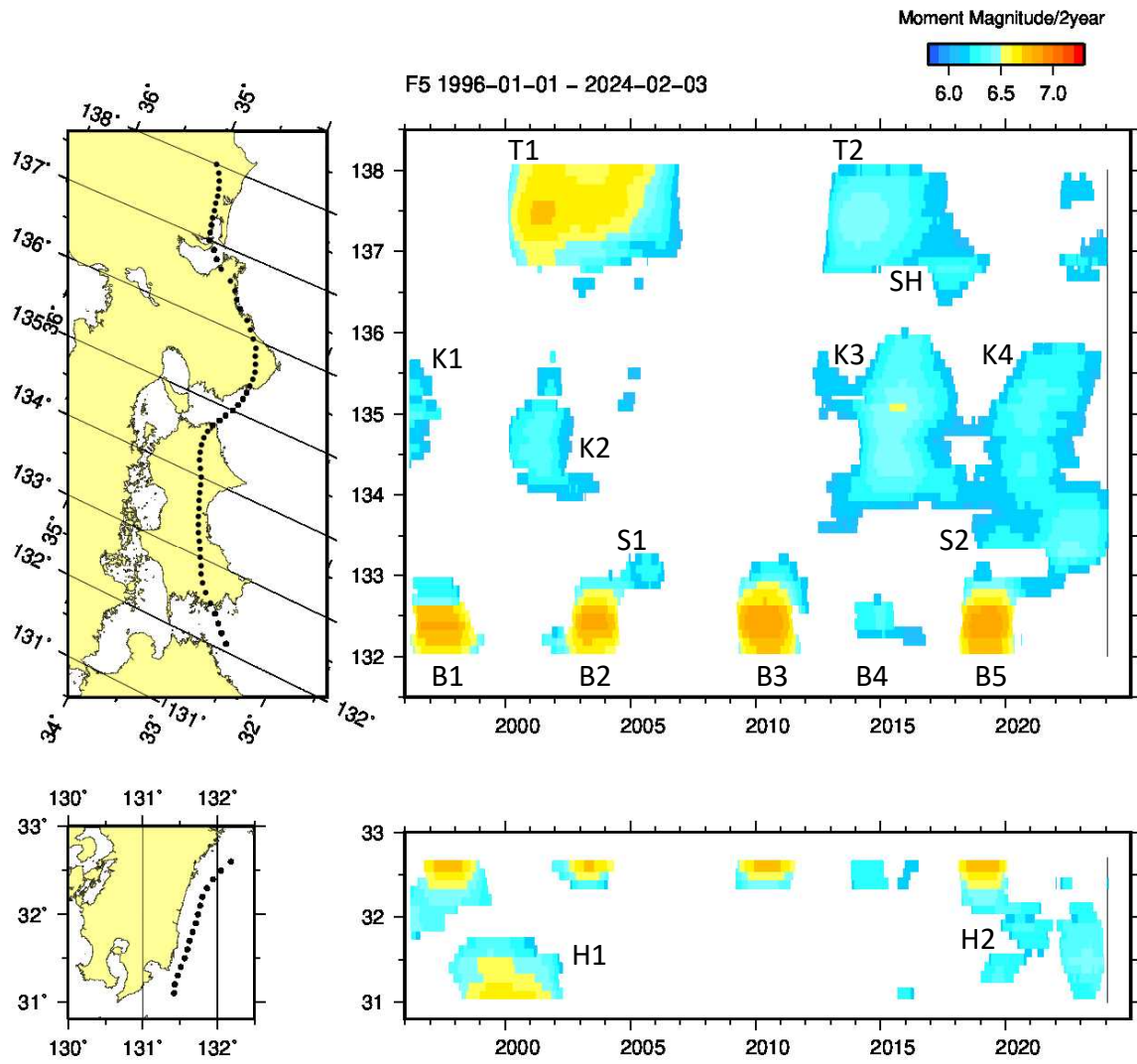
第2図 長期的スロースリップの規模分布 (1996年～2024年2月) 2年間あたりの変化量から推定したモーメントマグニチュード。
