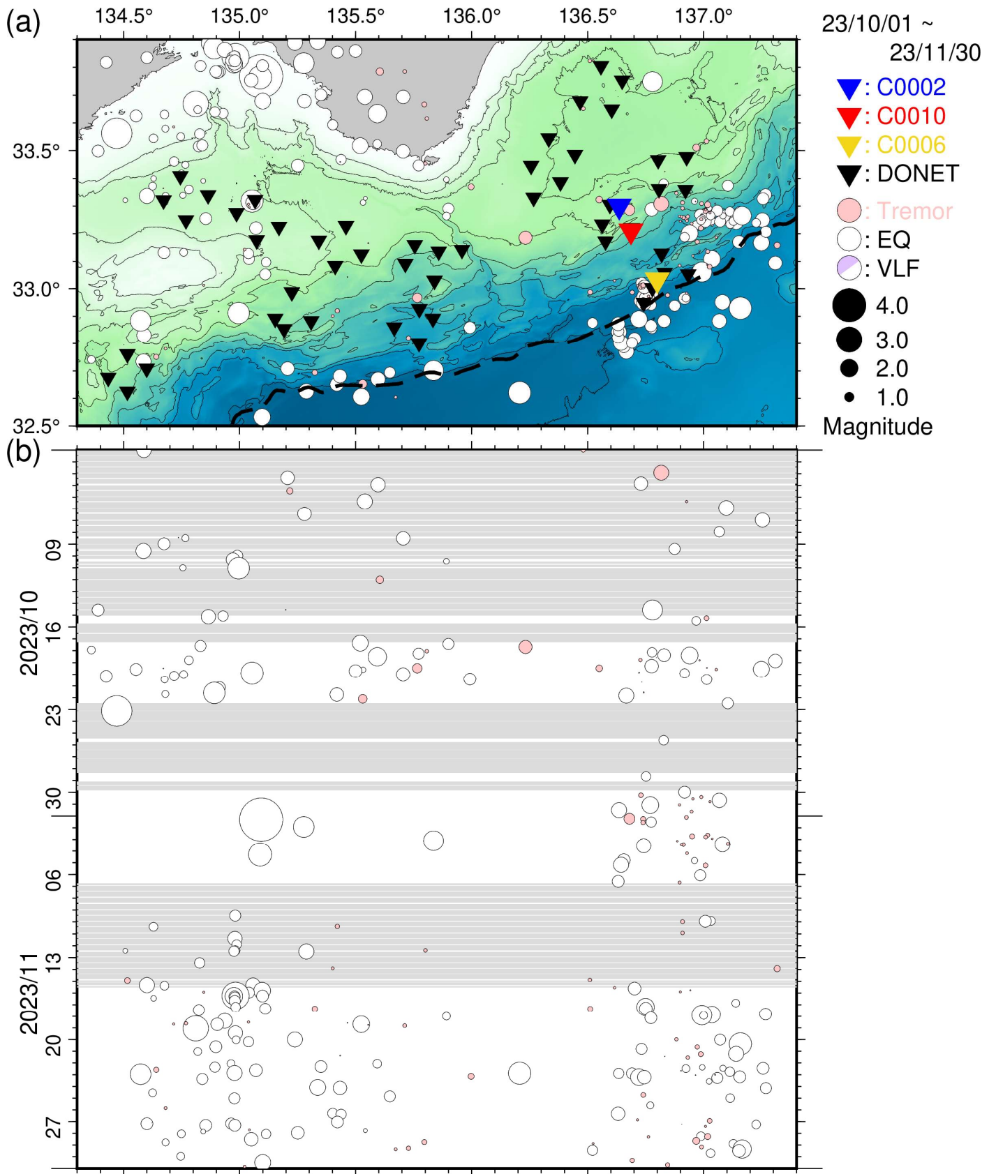
図5 直近2ヵ月間において熊野灘から室戸沖にて発生した低周波微動・通常地震・超低周波地震 (2023年10月1日~2023年11月30日)。図3と同様のシンボルにて表示。(a) 震央分布図。(b) aに示した震央を経度方向へ投影した時空間分布図。
