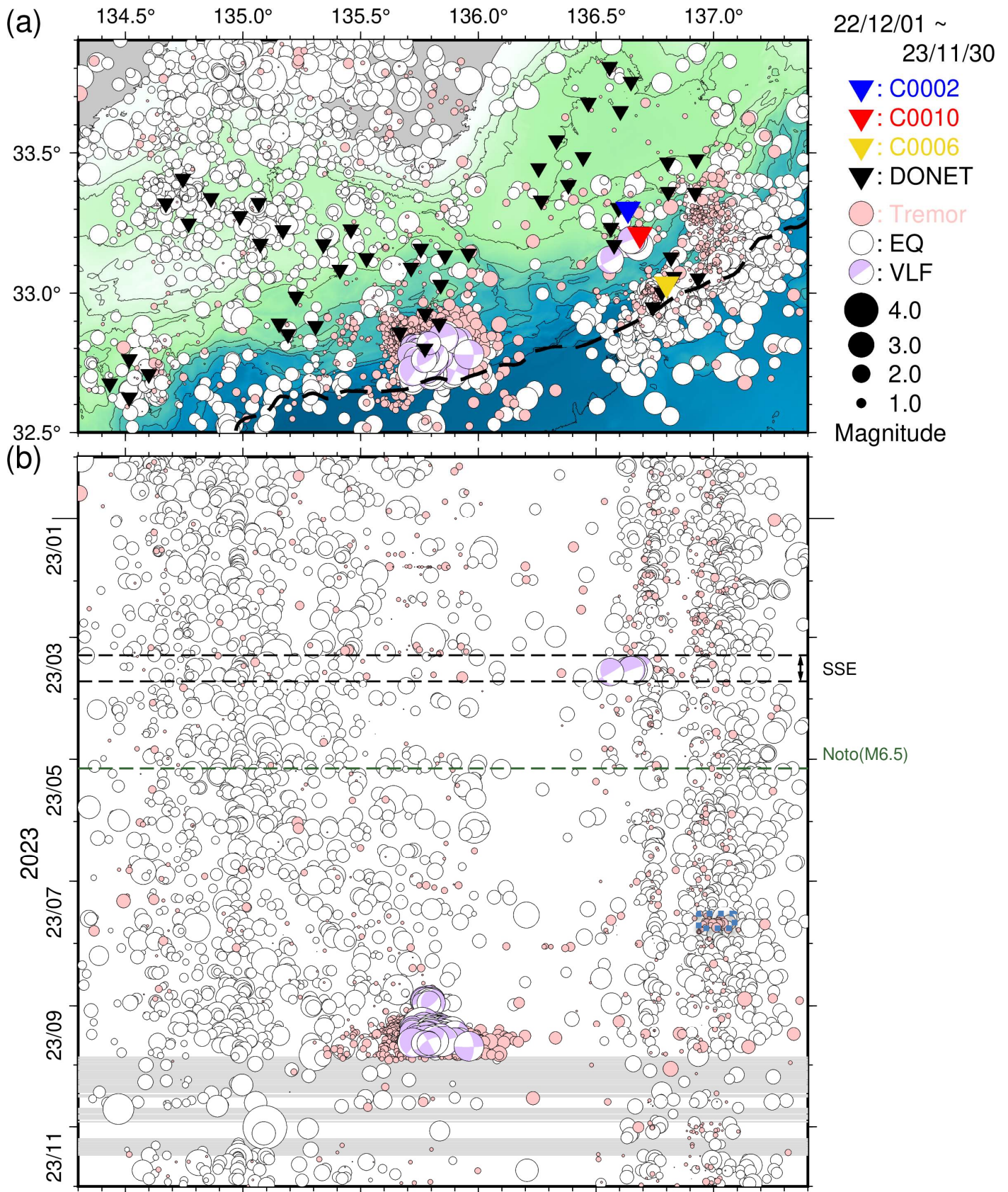
図 6 直近 1 年間に於いて熊野灘から室戸沖にて発生した低周波微動・通常地震・超低周波地震 (2022 年 12 月 1 日~2023 年 11 月 30 日)。図 4 と同様のシンボルにて表示。(a) 震央分布図。(b) a に示した震央を経度方向へ投影した時空間分布図。青点線の長方形領域は、DONET1 の B ノード付近における低周波微動の群発的な活動を示す。なお、図 3 および図 5 において過去資料に緑点線で記した地震のうち、a の領域外かつ M6.5 未満のものは掲載していない。
