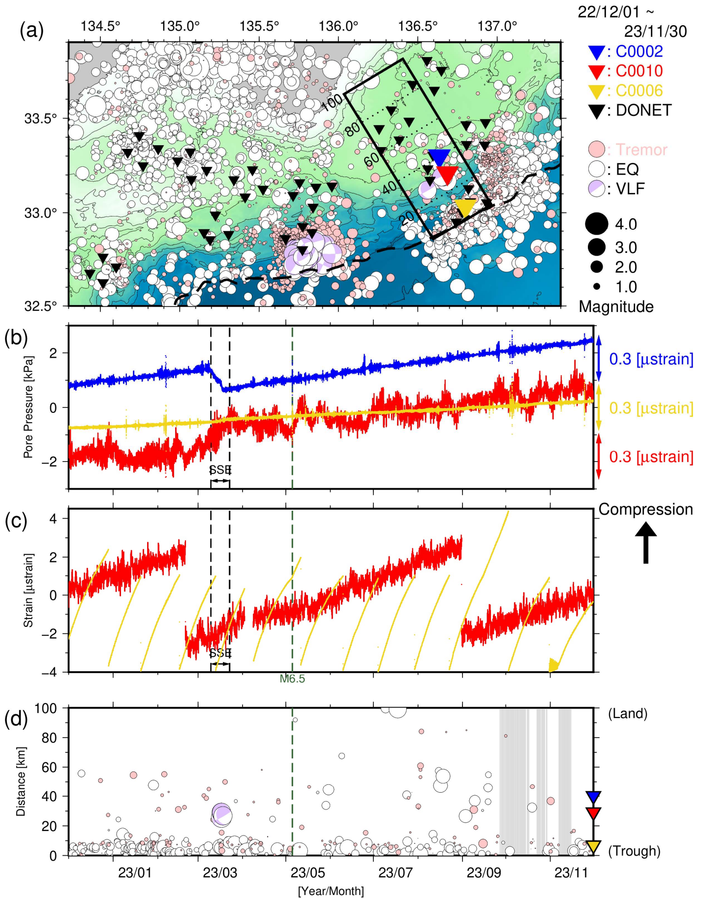
図4 直近1年間のSSE・低周波微動モニタリング(2022年12月1日~2023年11月30日)。(a)低周波微動・通常地震・超低周波地震の震央分布。(b)間隙水圧変化。(c)体積歪変化。(d)時空間分布。緑点線は、5月5日の能登地方地震を示す。なお、図3において過去資料に緑点線で記した地震のうち、aの領域外かつM6.5未満のものは掲載していない。
