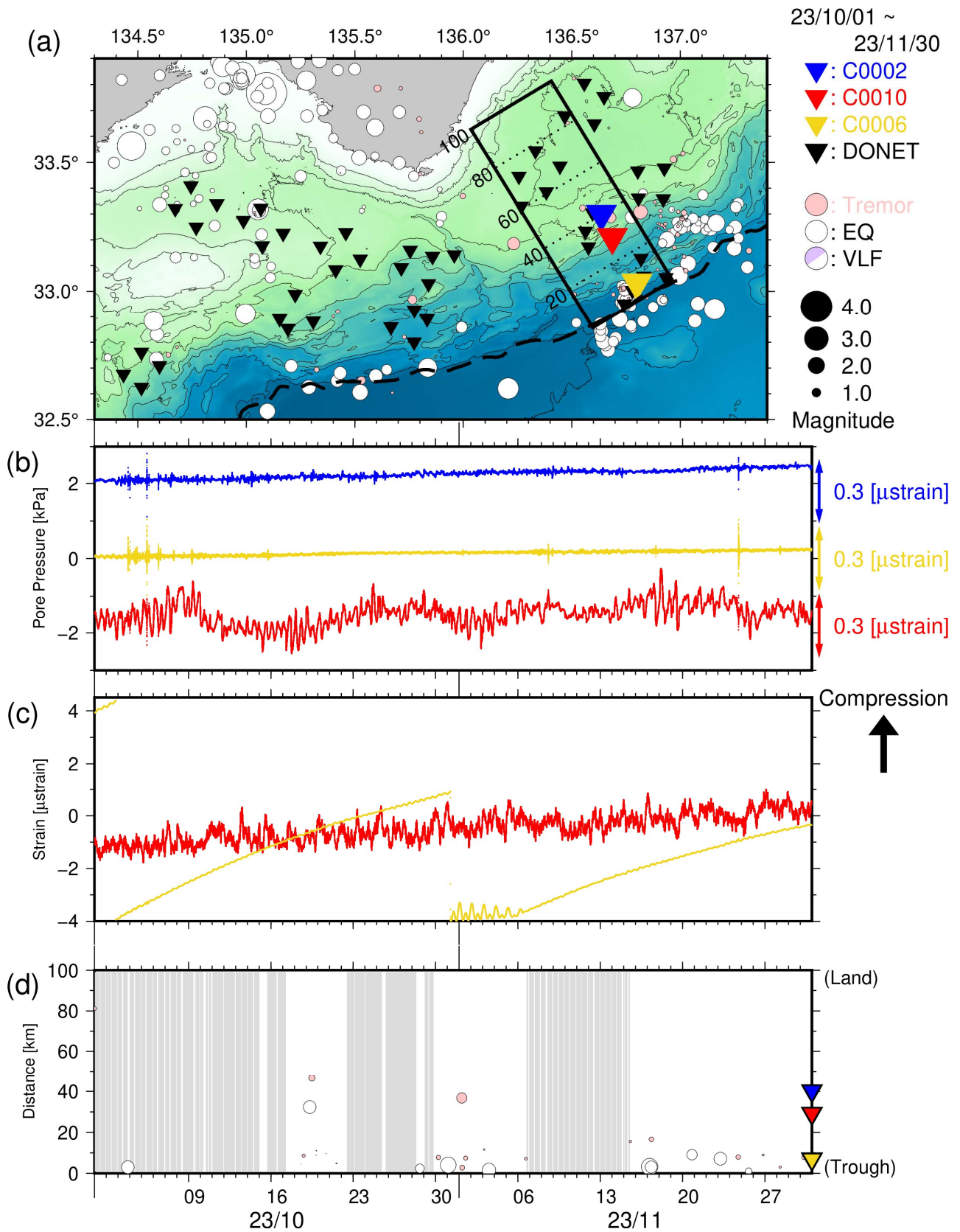
図3 直近2ヶ月間のSSE・低周波微動モニタリング（2023年10月1日～2023年11月30日）。 (a) 震央分布図（●：低周波微動（深さ0～15 km）、○：通常地震（深さ0～60 km）、●：超低周波地震のメカニズム解）。▼、▼、▼、▼は、それぞれC0002・C0010・C0006・DONET観測点。破線はトラフ軸。(b) 長期孔内観測点における間隙水圧変化（—：C0002、—：C0010、—：C0006）。 (c) 長期孔内観測点における体積歪変化（—：C0010、—：C0006）。(d) 図3a中に実線で示した矩形領域内における、低周波微動・通常地震・超低周波地震の時空間分布。縦軸は、トラフ軸からの距離（km）。灰色はエアガン発振期間を示す。
