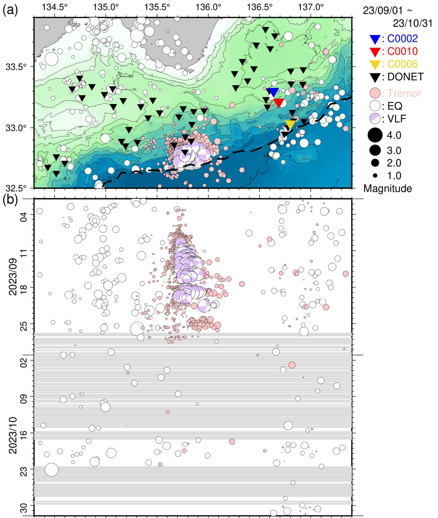
図5 直近2ヵ月間において熊野灘から室戸沖にて発生した低周波微動・通常地震・超低周波地震（2023年9月1日～2023年10月31日）。図3と同様のシンボルにて表示。(a) 震央分布図。(b) aに示した震央を経度方向へ投影した時空間分布図。
