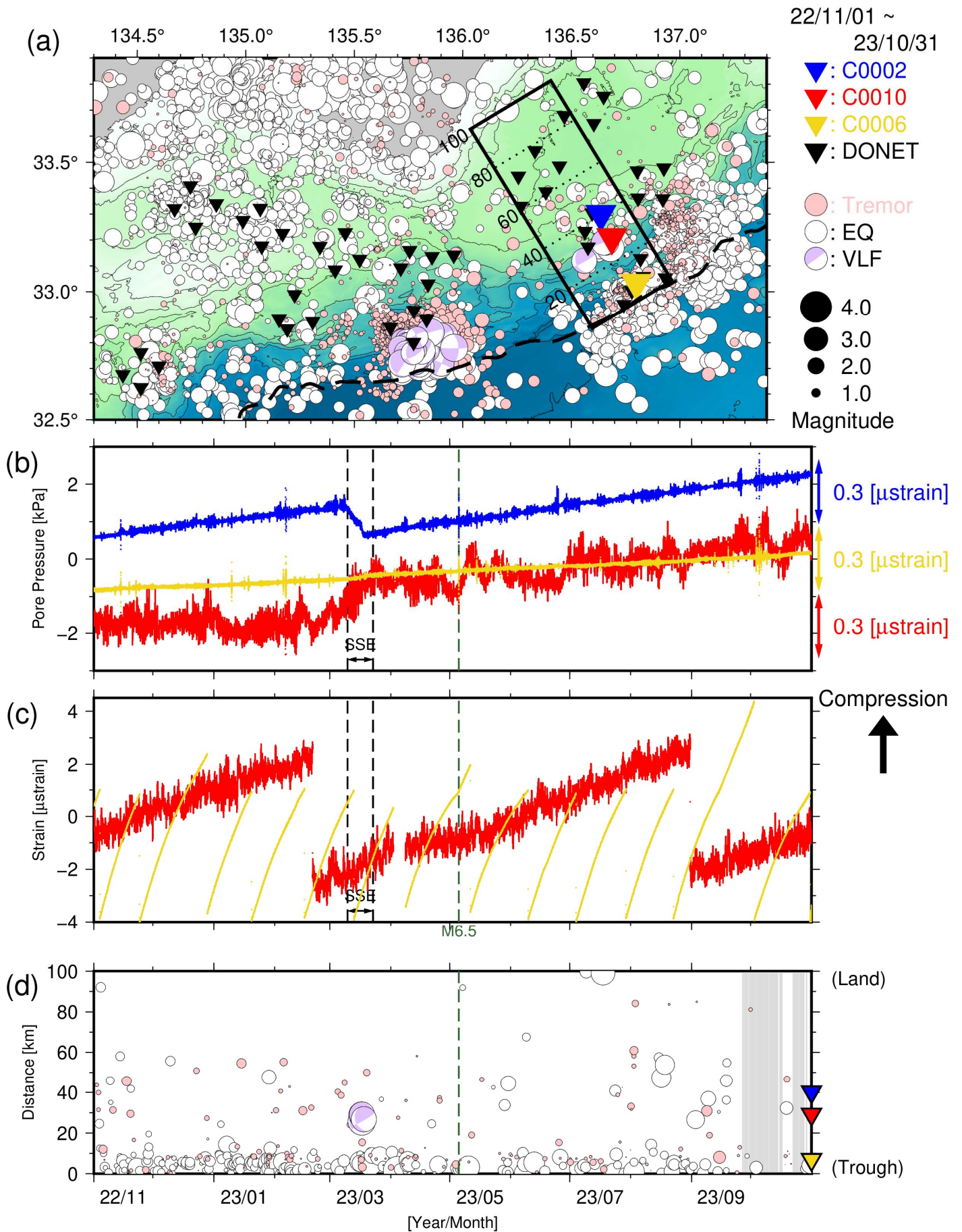
図4 直近1年間のSSE・低周波微動モニタリング(2022年11月1日~2023年10月31日)。(a)低周波微動・通常地震・超低周波地震の震央分布。(b)間隙水圧変化。(c)体積歪変化。(d)時空間分布。緑点線は、5月5日の能登地方地震を示す。なお、図3において過去資料に緑点線で記した地震のうち、aの領域外かつM6.5未満のものは掲載していない。
