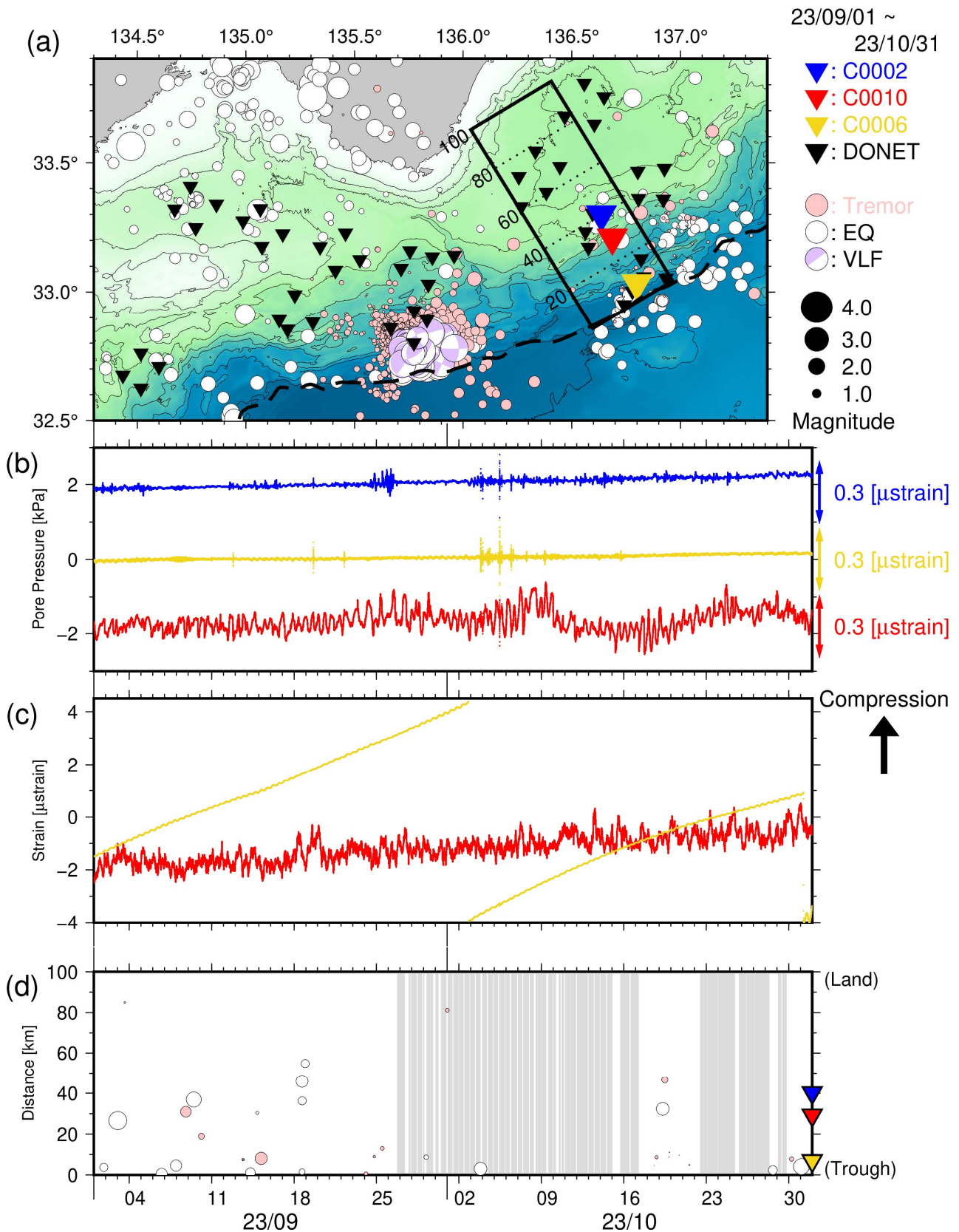
図3 直近2ヶ月間のSSE・低周波微動モニタリング(2023年9月1日~2023年10月31日)。 (a) 震央分布図(●:低周波微動(深さ0~15km)、○:通常地震(深さ0~60km)、●:超低周波地震のメカニズム解)。▼▼▼▼は、それぞれC0002・C0010・C0006・DONET観測点。破線はトラフ軸。(b) 長期孔内観測点における間隙水圧変化(—:C0002、—:C0010、—:C0006)。(c) 長期孔内観測点における体積歪変化(—:C0010、—:C0006)。(d) 図3a中に実線で示した矩形領域内における、低周波微動・通常地震・超低周波地震の時空間分布。縦軸は、トラフ軸からの距離(km)。灰色はエアガン発振期間を示す。
