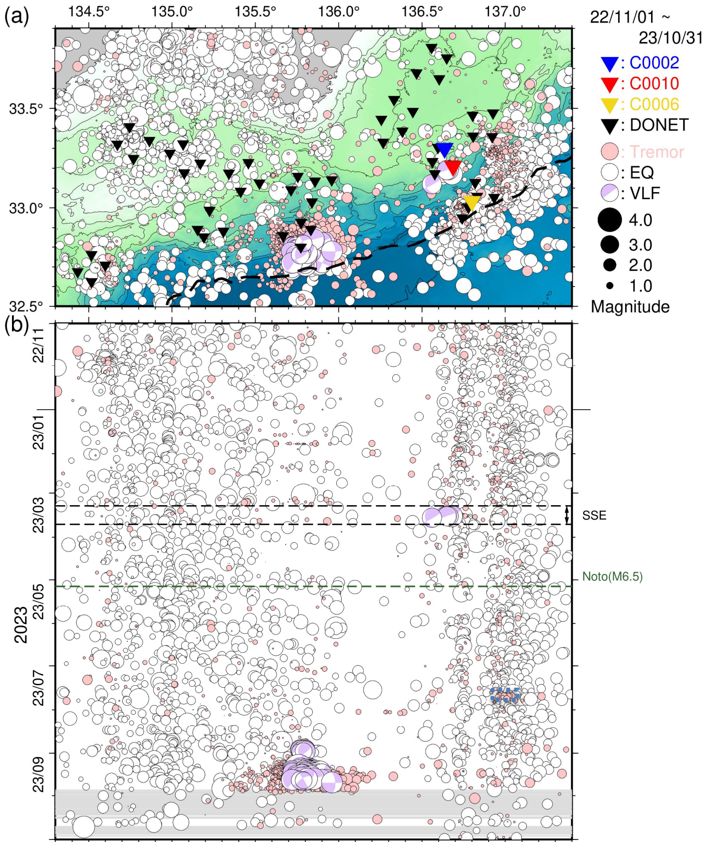
図 6 直近 1 年間に於いて熊野灘から室戸沖にて発生した低周波微動・通常地震・超低周波地震 (2022 年 11 月 1 日~2023 年 10 月 31 日)。図 4 と同様のシンボルにて表示。(a) 震央分布図。(b) a に示した震央を経度方向へ投影した時空間分布図。青点線の長方形領域は、DONET1 の B ノード付近における低周波微動の群発的な活動を示す。なお、図 3 および図 5 において過去資料に緑点線で記した地震のうち、a の領域外かつ M6.5 未満のものは掲載していない。
