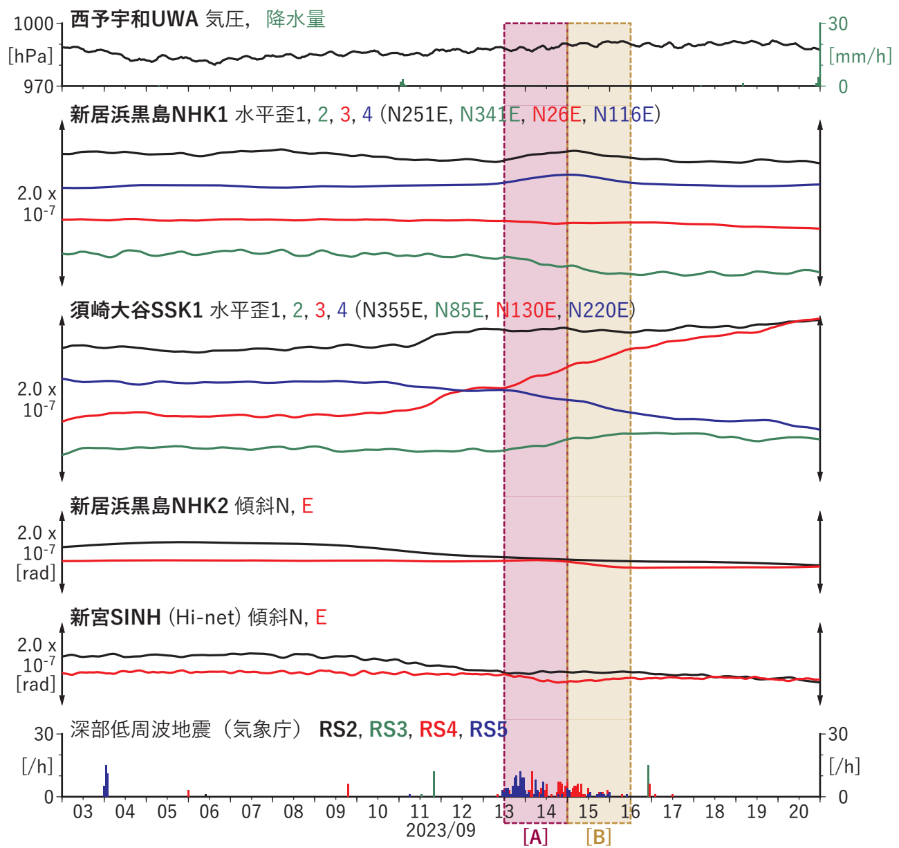
図5 四国地方における歪・傾斜の時間変化 (2023/09/03 00:00 - 2023/09/21 00:00 (JST))
