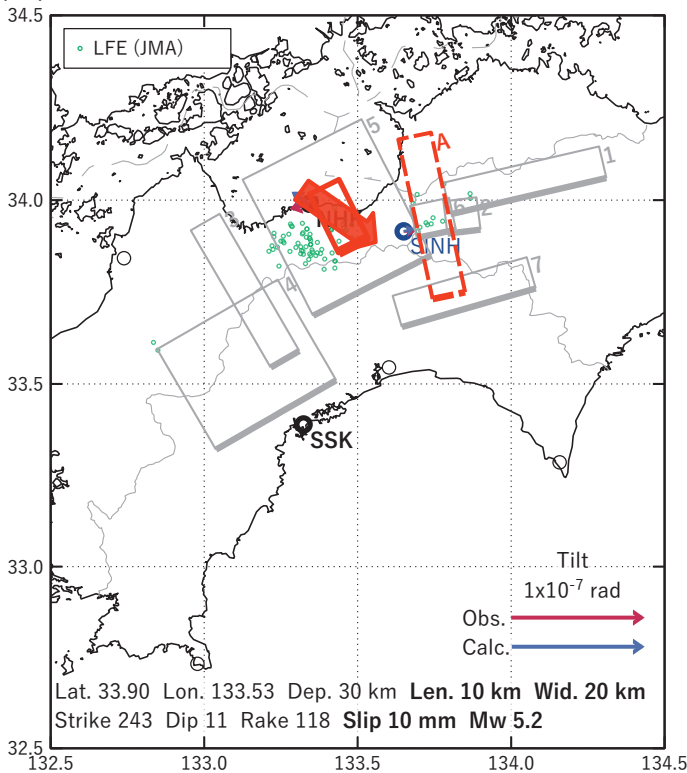
図7 2023/09/15 - 16AM の歪・傾斜変化 (図5 [B]) を説明する断層モデル。
