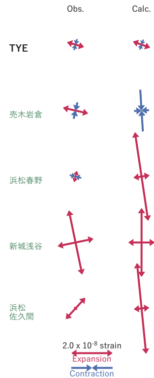
図3 2023/09/15 - 17 の歪・傾斜変化 (図2 [A]) を説明する断層モデル。
