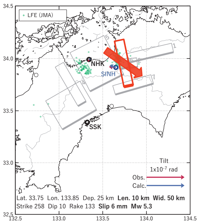
図6 2023/09/13PM - 14 の歪・傾斜変化 (図5 [A]) を説明する断層モデル。
