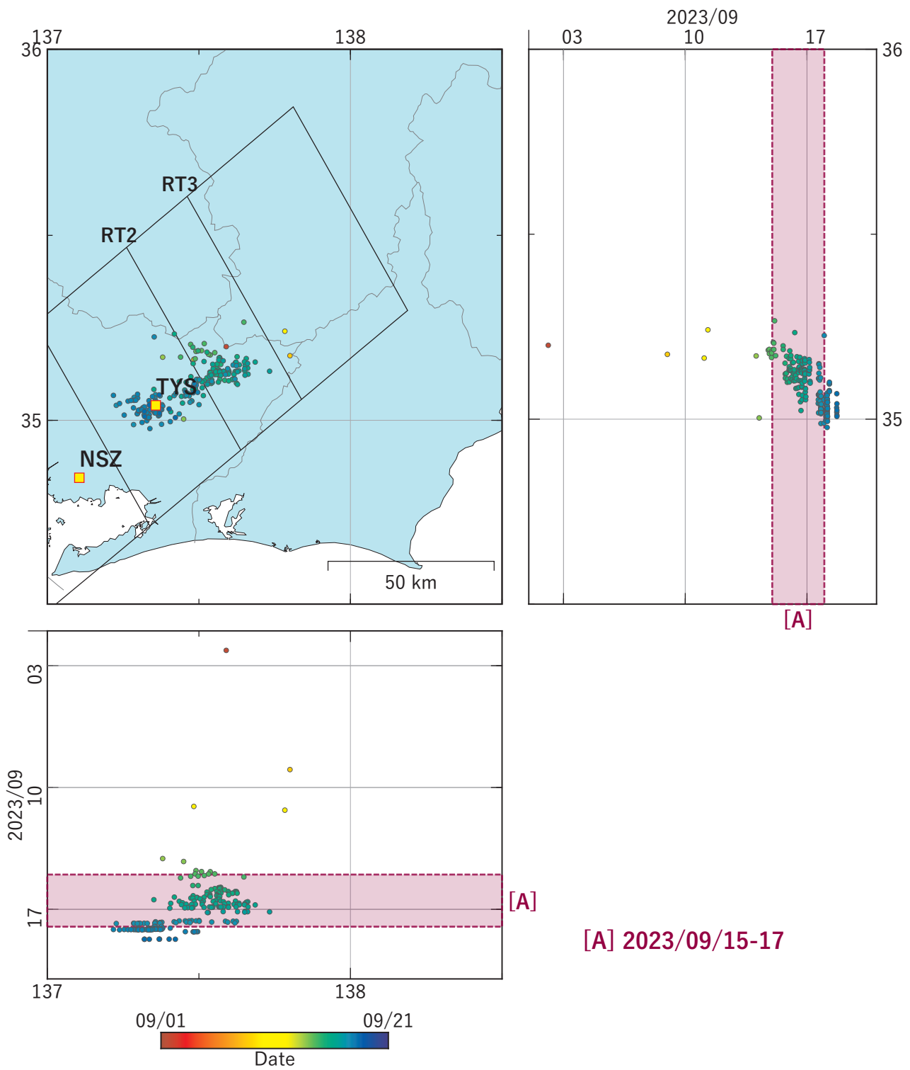
図1 東海地方における深部低周波地震の時空間分布図。 (2023/09/01 00:00 - 2023/09/21 00:00 (JST)) 気象庁カタログによる。
