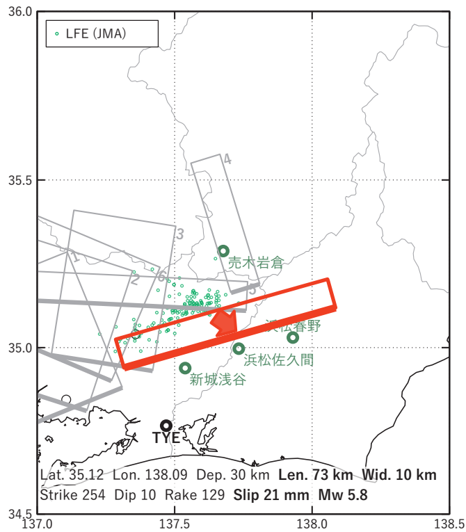
図3 2023/09/15 - 17 の歪・傾斜変化 (図2 [A]) を説明する断層モデル。
