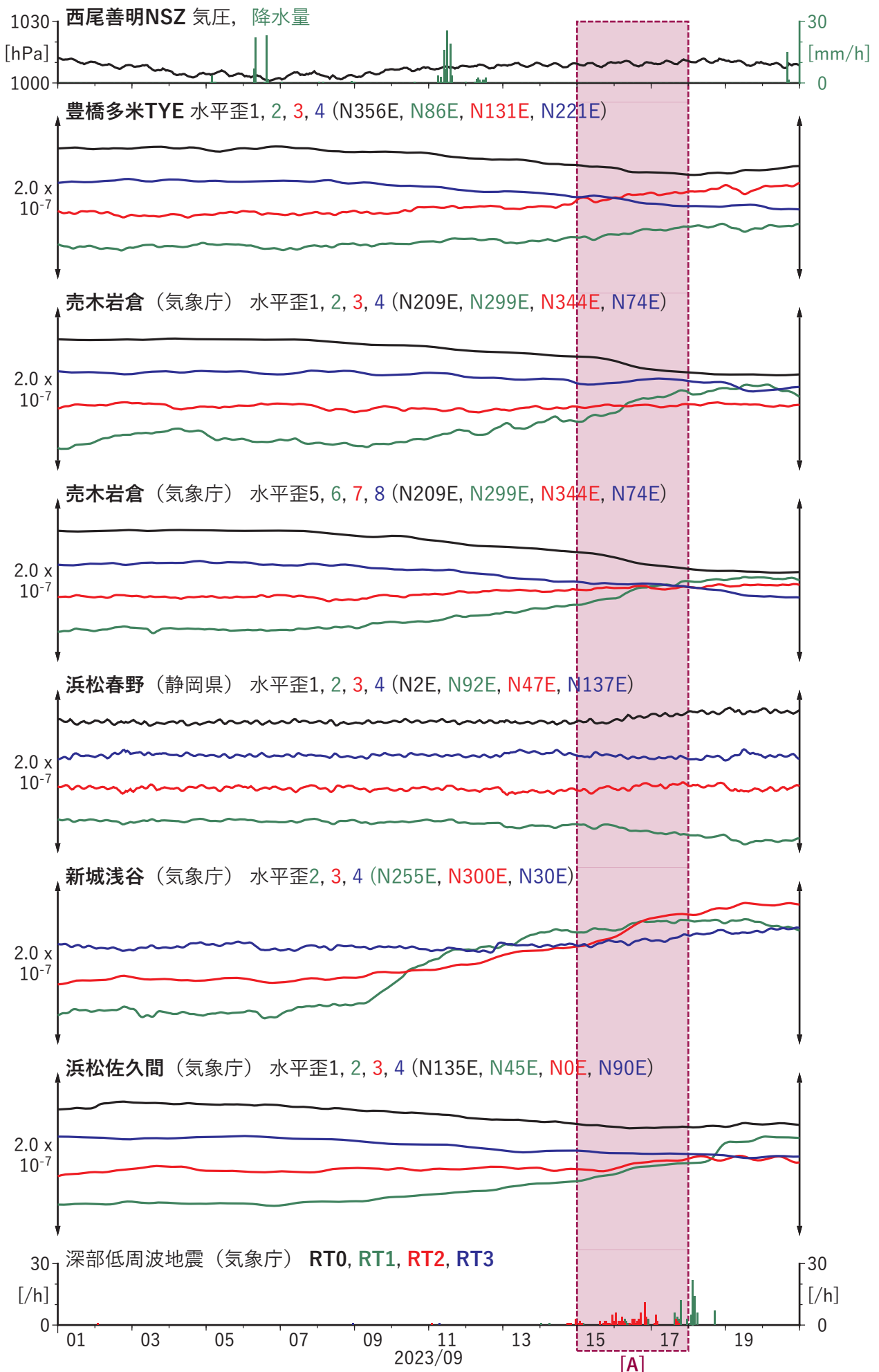
図2 東海地方における歪の時間変化 (2023/09/01 00:00 - 2023/09/21 00:00 (JST))
