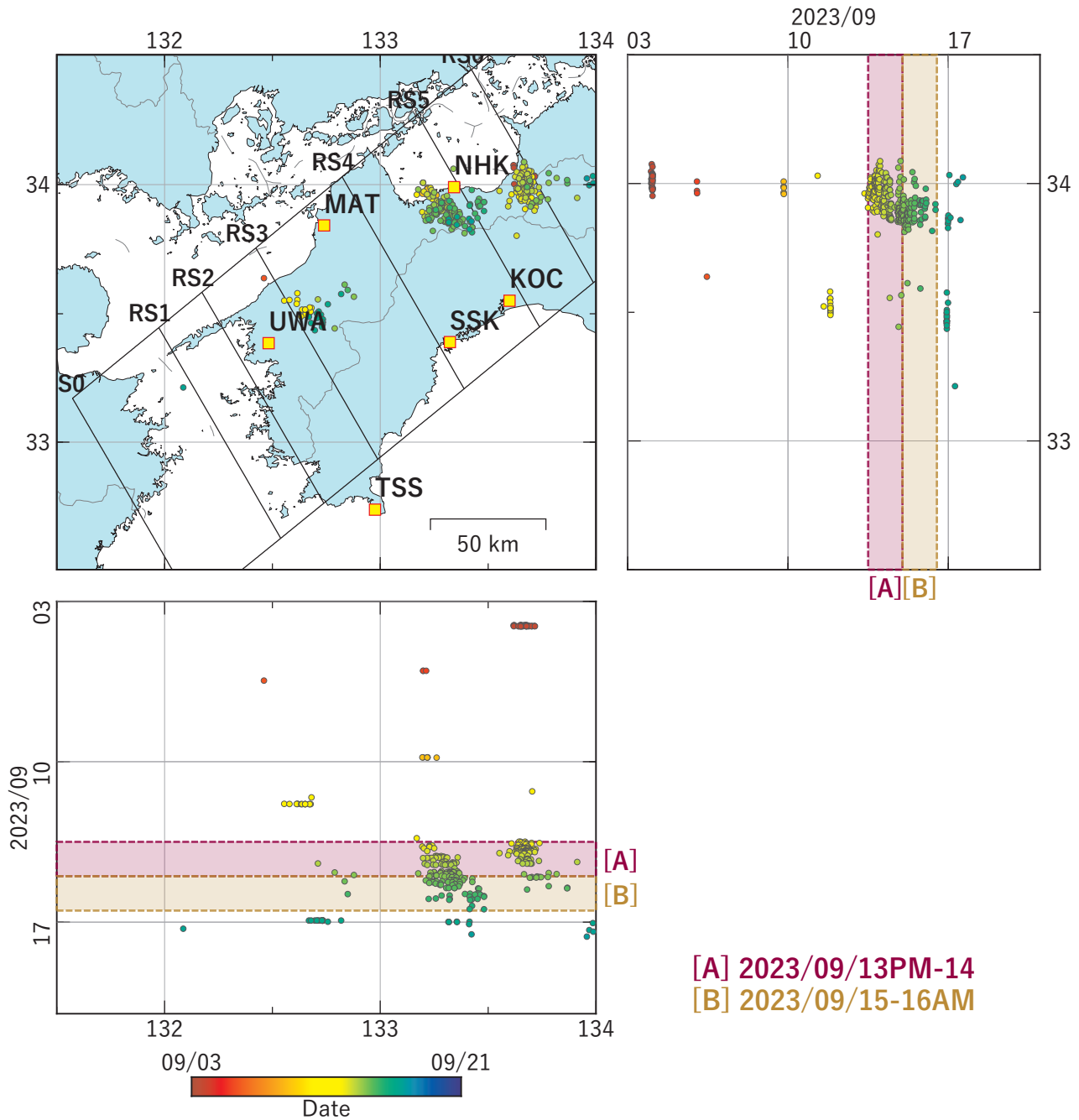
図4 四国地方における深部低周波地震の時空間分布図。 (2023/09/03 00:00 - 2023/09/21 00:00 (JST)) 気象庁カタログによる。
