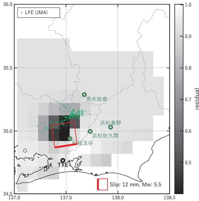
(b1) 推定した断層モデル
