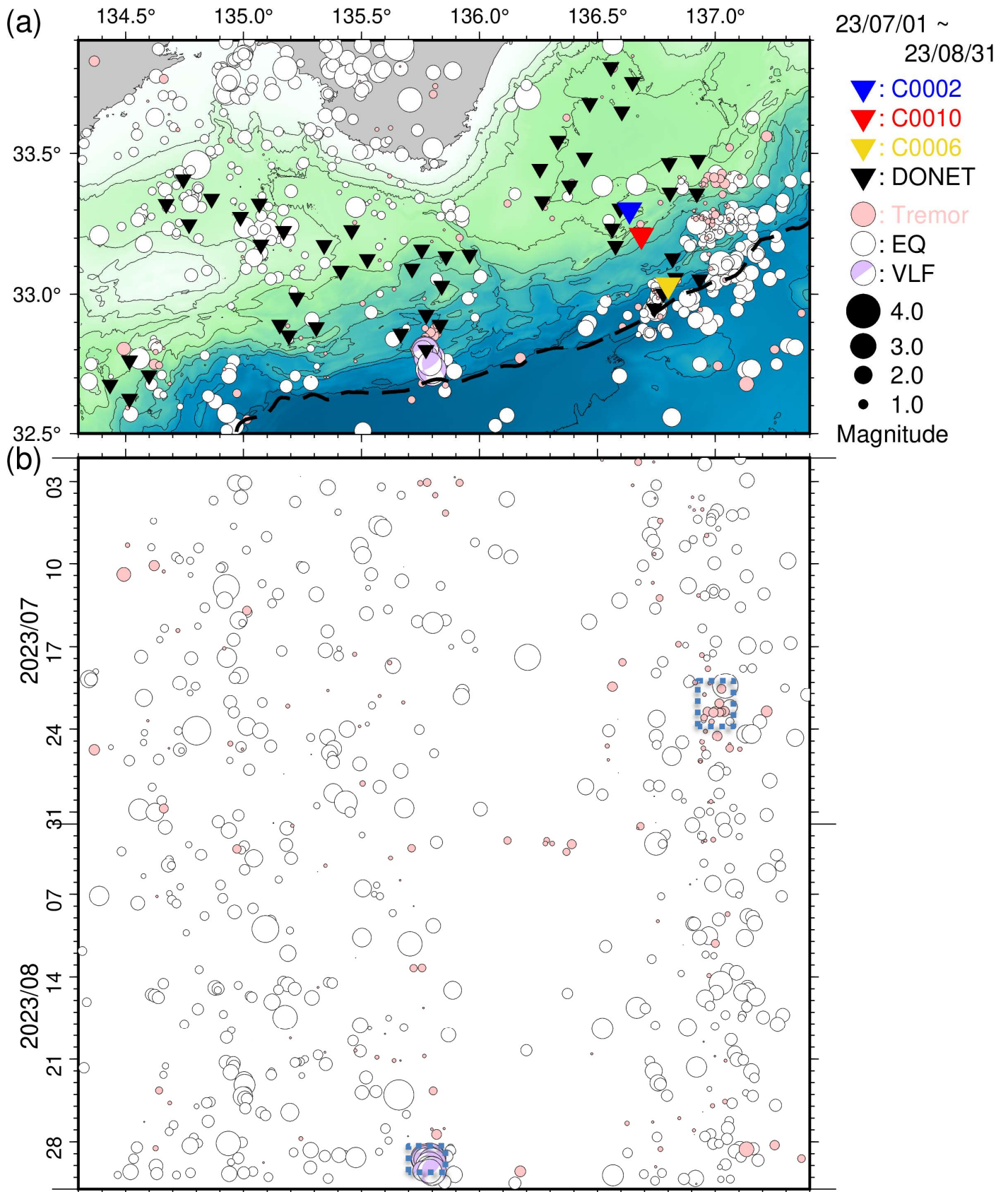
図5 直近2ヵ月間において熊野灘から室戸沖にて発生した低周波微動・通常地震・超低周波地震 (2023年7月1日~2023年8月31日)。図3と同様のシンボルにて表示。(a) 震央分布図。(b) aに示した震央を経度方向へ投影した時空間分布図。青点線の長方形領域は、DONET1のBノード付近及びDONET2のEノード付近における低周波微動の群発的な活動を示す。
