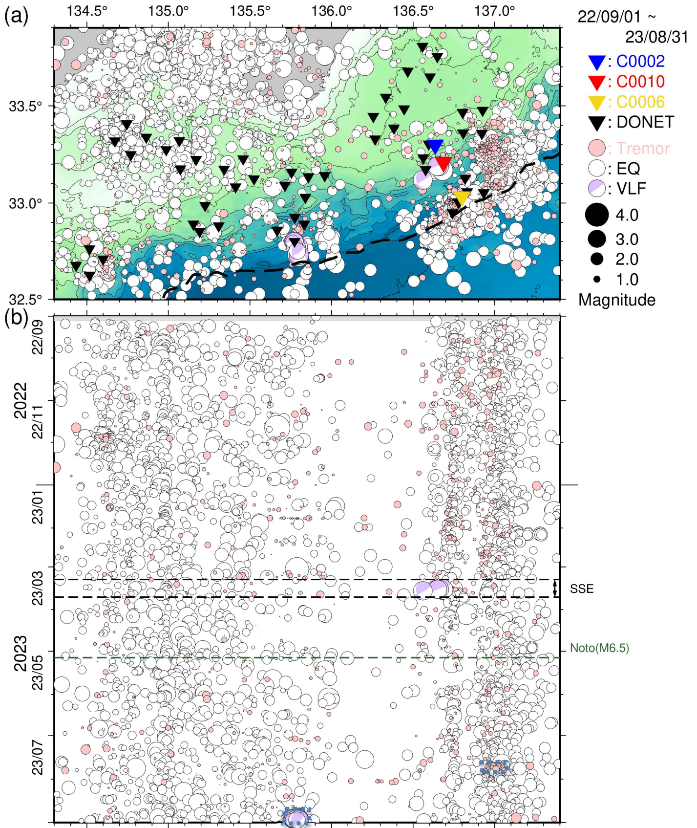
図 6 直近 1 年間に於いて熊野灘から室戸沖にて発生した低周波微動・通常地震・超低周波地震 (2022 年 9 月 1 日~2023 年 8 月 31 日)。図 4 と同様のシンボルにて表示。(a) 震央分布図。(b) a に示した震央を経度方向へ投影した時空間分布図。なお、図 3 および図 5 において過去資料に緑点線で記した地震のうち、a の領域外かつ M6.5 未満のものは掲載していない。
