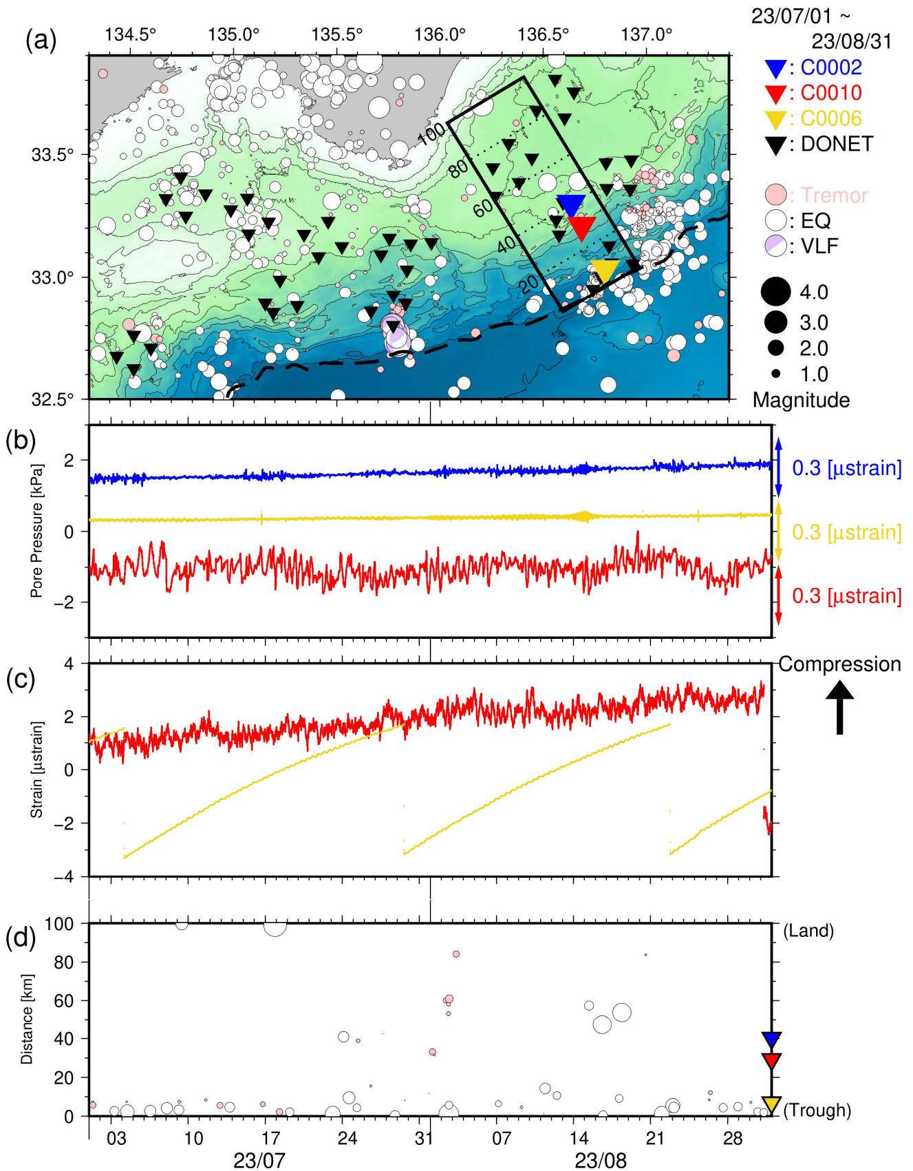
図3 直近2ヶ月間のSSE・低周波微動モニタリング(2023年7月1日~2023年8月31日)。(a)震央分布図(●:低周波微動(深さ0~15km)、○:通常地震(深さ0~60km)、●:超低周波地震のメカニズム解)。 ▼ ▼ ▼ ▼ は、それぞれC0002・C0010・C0006・DONET観測点。破線はトラフ軸。(b)長期孔内観測点における間隙水圧変化(—:C0002、—:C0010、—:C0006)。(c)長期孔内観測点における体積歪変化(—:C0010、—:C0006)。(d)図3a中に実線で示した矩形領域内における、低周波微動・通常地震・超低周波地震の時空間分布。縦軸は、トラフ軸からの距離(km)。
