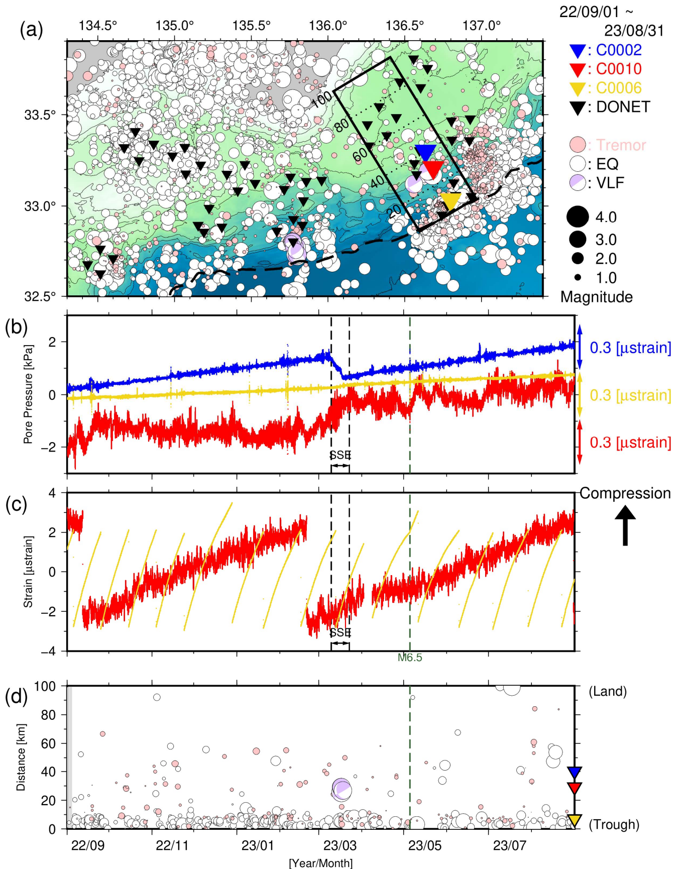
図4 直近1年間のSSE・低周波微動モニタリング(2022年9月1日~2023年8月31日)。(a)低周波微動・通常地震・超低周波地震の震央分布。(b)間隙水圧変化。(c)体積歪変化。(d)時空間分布。灰色はエアガン発振期間を示す。緑点線は、5月5日の能登地方地震を示す。なお、図3において過去資料に緑点線で記した地震のうち、aの領域外かつM6.5未満のものは掲載していない。
