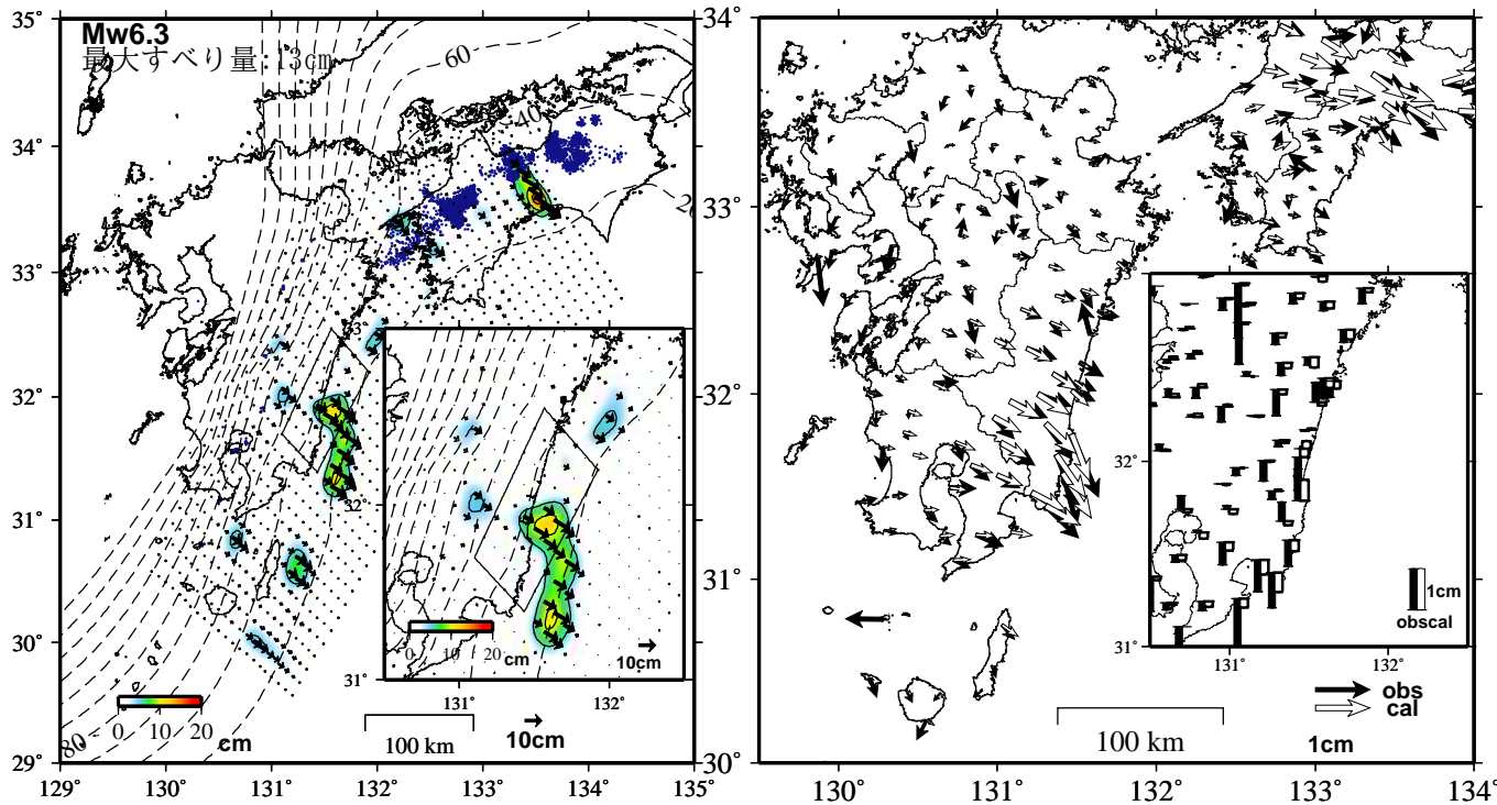
推定すべり分布 (2022-07-01/2023-08-10)
