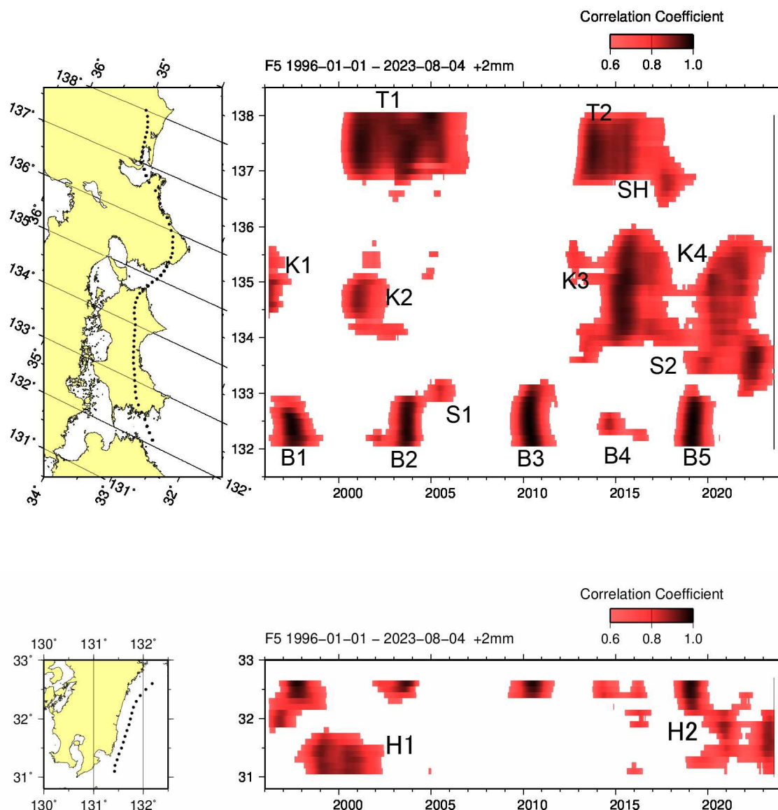
第1図 長期的スロースリップ客観検知図（1996年から2023年8月）
