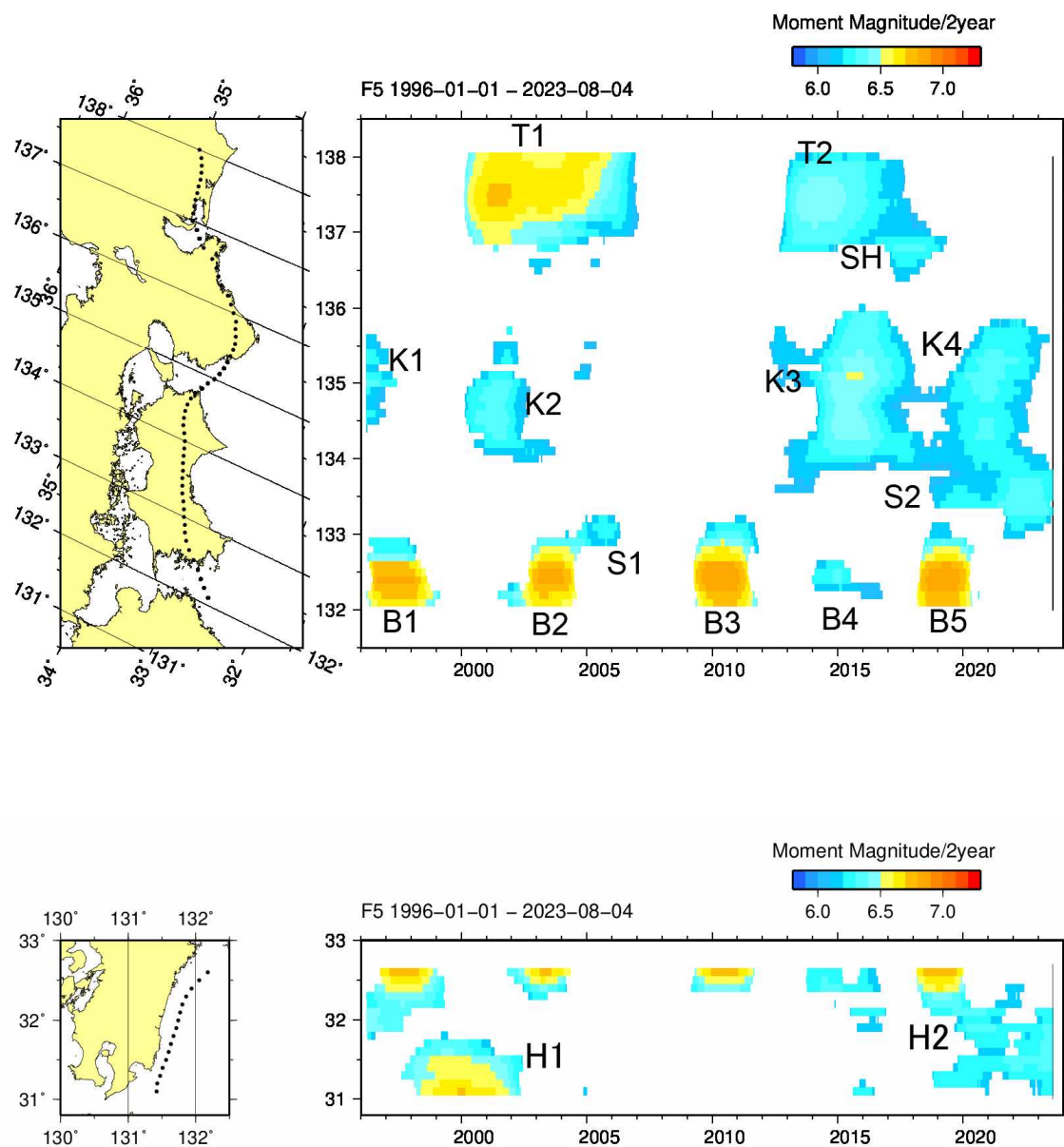
第2図 長期的スロースリップの規模分布（1996年から2023年8月） 2年間あたりの変化量から推定したモーメントマグニチュード。地域略号は第1図と同じ。
