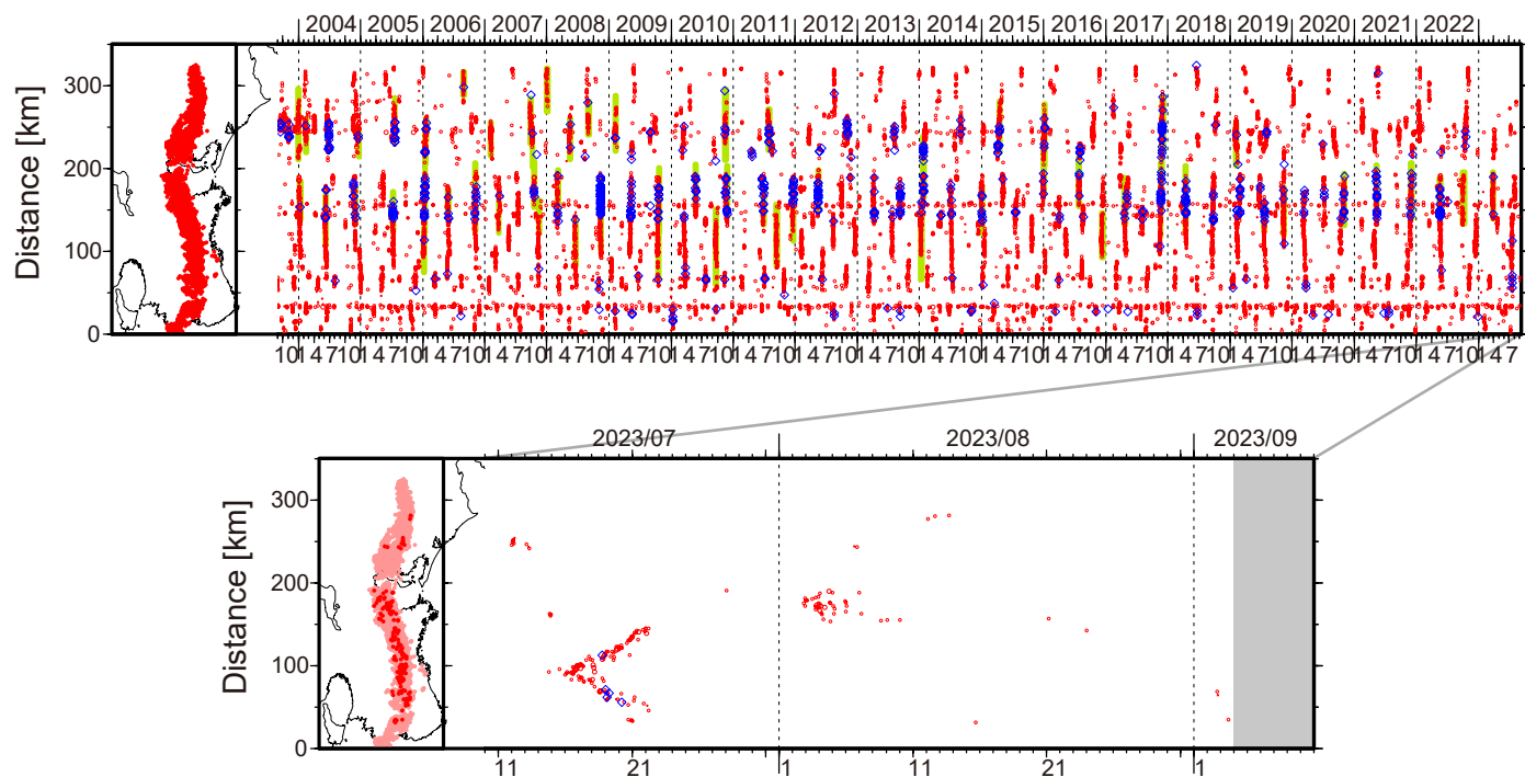
図 1. 紀伊半島・東海地域における 2003 年 9 月～2023 年 9 月 3 日までの深部低周波微動の時空間分布（上図）．赤丸はエンベロープ相関・振幅ハイブリッド法 (Maeda and Obara, 2009) およびクラスタ処理 (Obara et al., 2010) によって 1 時間毎に自動処理された微動分布の重心である．青菱形は周期 20 秒に卓越する超低周波地震 (Ito et al., 2007) である．黄緑色の太線はこれまでに検出された短期的スロースリップイベント (SSE) を示す．下図は 2023 年 8 月を中心とした期間の拡大図である．8 月 2 ～ 10 日頃には三重県北部において、やや活発な活動がみられた．この活動では北東・南西両方向への活動域の拡大がややみられ、その後 7 日頃から活動は低調となった．9 月 2 ～ 3 日頃には奈良県南部から和歌山県中部において、ごく小規模な微動活動がみられた．8 月 12 日 3:09 頃に三河湾付近の深さ約 39km で発生した M4.4 の地震 (Hi-net 暫定値) の後、3:15 頃から愛知県東部において微動活動が開始し、クラスタリング処理結果では 15 時台にも活動が推定されている．8 月 23 日 23:22 頃 (JST) にアルゼンチン付近の深さ約 570km で発生した M6.2 の地震 (USGS) の後、8 月 24 日の 0:15 ～ 0:25 頃に三重県中部において微動活動がみられた．
