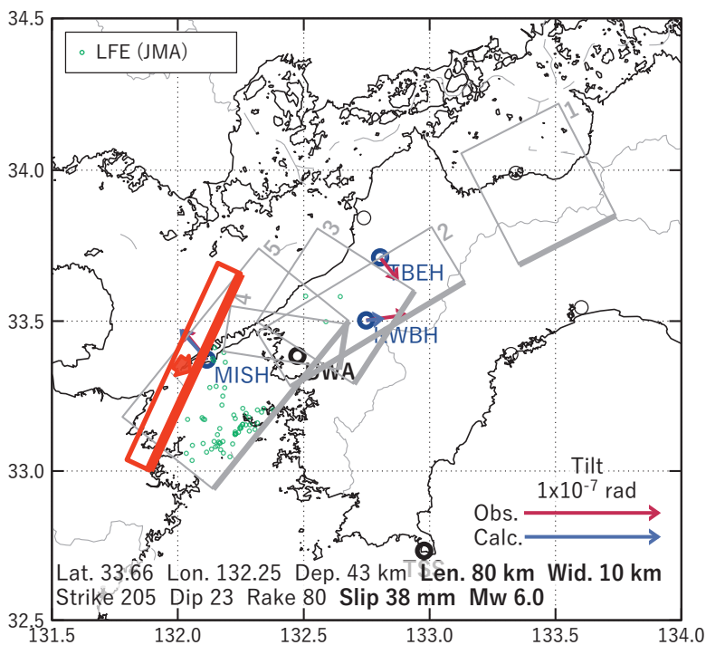
図6 2023/08/15 - 18AM の歪・傾斜変化 (図5 [A]) を説明する断層モデル。
