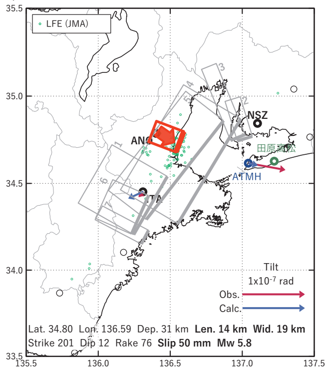
図3 2023/08/03 - 05 の歪・傾斜変化（図2 [A]）を説明する断層モデル。
