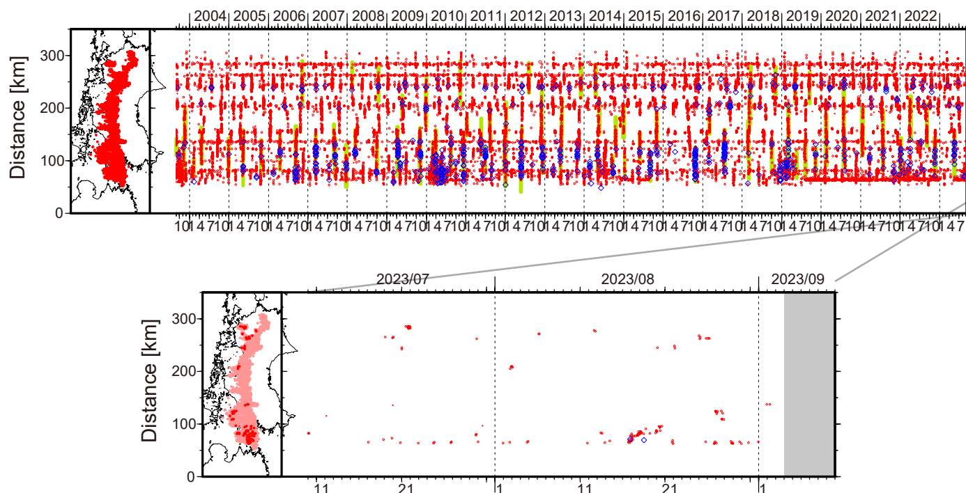
図 1. 四国における 2003 年 9 月 ~ 2023 年 9 月 3 日までの深部低周波微動の時空間分布 (上図). 赤丸はエンベロープ相関・振幅ハイブリッド法 (Maeda and Obara, 2009) およびクラスター処理 (Obara et al., 2010) によって 1 時間毎に自動処理された微動分布の重心である. 青菱形は周期 20 秒に卓越する超低周波地震 (Ito et al., 2007) である. 黄緑色太線は、これまでに検出された短期的スロースリップイベント (SSE) を示す. 下図は 2023 年 8 月を中心とした期間の拡大図である. 8 月 16 ~ 20 日頃には豊後水道においてやや活発な活動がみられた. この活動は豊後水道西部で開始し、やや東方向への活動域の移動がみられた. 8 月 2 ~ 3 日頃には愛媛県東部において、8 月 24 ~ 26 日頃には香川・徳島県境付近において、それぞれごく小規模な活動がみられた. 8 月 26 ~ 27 日頃に愛媛県西部において発生したごく小規模な活動は、8 月 26 日 22:29 頃に周防灘付近の深さ約 74km で発生した M5.4 (Hi-net 暫定値) の地震後、22:35 頃から開始した.
