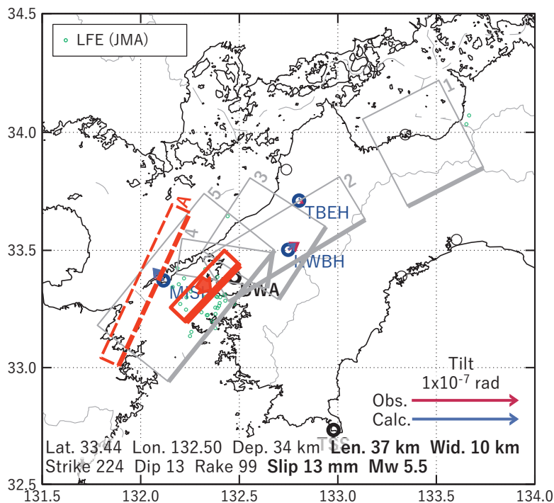
図7 2023/08/18PM-20 の歪・傾斜変化（図5[B]）を説明する断層モデル。
