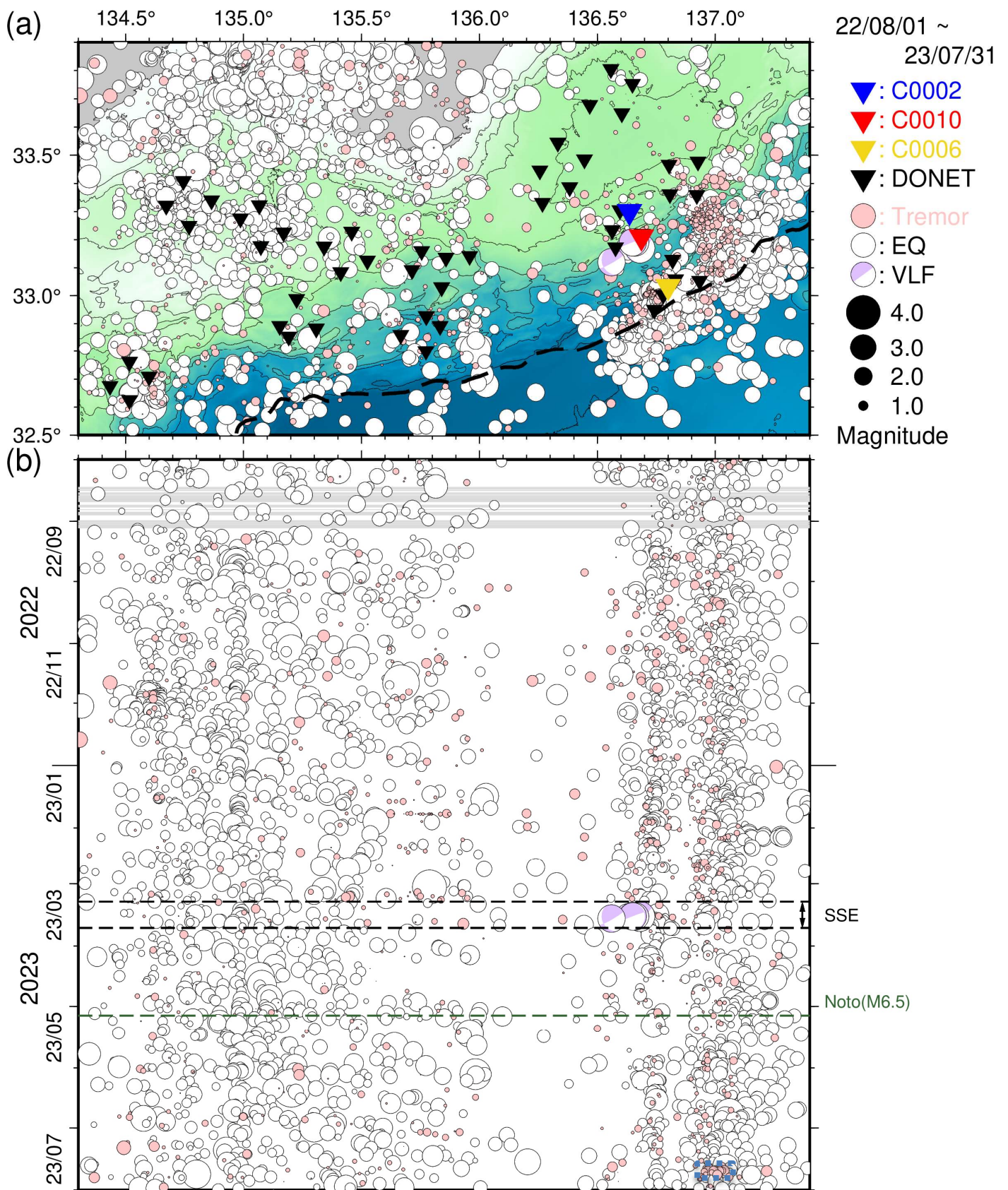
図 6 直近 1 年間に於いて熊野灘から室戸沖にて発生した低周波微動・通常地震・超低周波地震 (2022 年 8 月 1 日~2023 年 7 月 31 日)。図 4 と同様のシンボルにて表示。(a) 震央分布図。(b) a に示した震央を経度方向へ投影した時空間分布図。なお、図 3 および図 5 において過去資料に緑点線で記した地震のうち、a の領域外かつ M6.5 未満のものは掲載していない。
