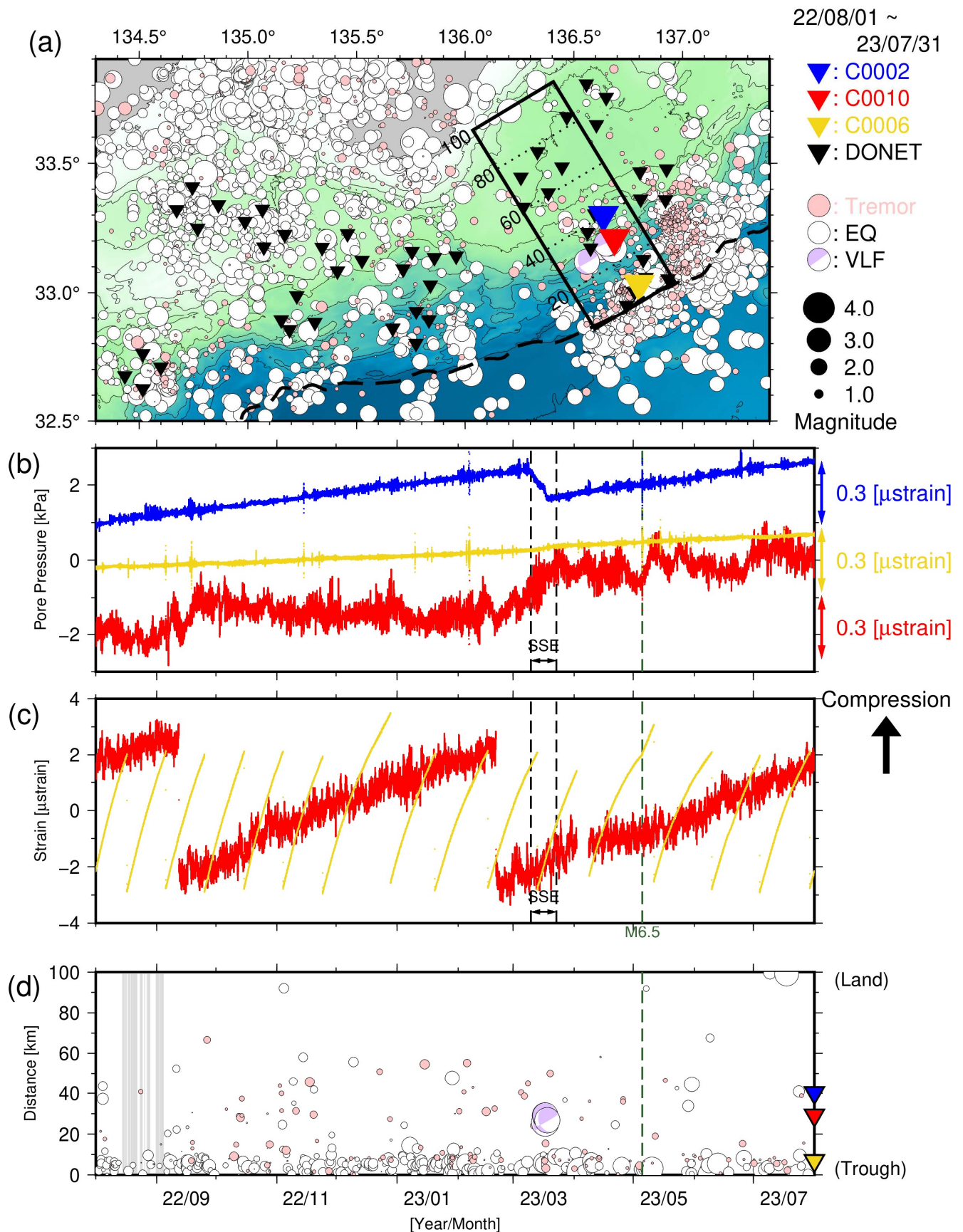
図4 直近1年間のSSE・低周波微動モニタリング(2022年8月1日~2023年7月31日)。(a)低周波微動・通常地震・超低周波地震の震央分布。(b)間隙水圧変化。(c)体積歪変化。(d)時空間分布。灰色はエアガン発振期間を示す。緑点線は、5月5日の能登地方地震を示す。なお、図3において過去資料に緑点線で記した地震のうち、aの領域外かつM6.5未満のものは掲載していない。
