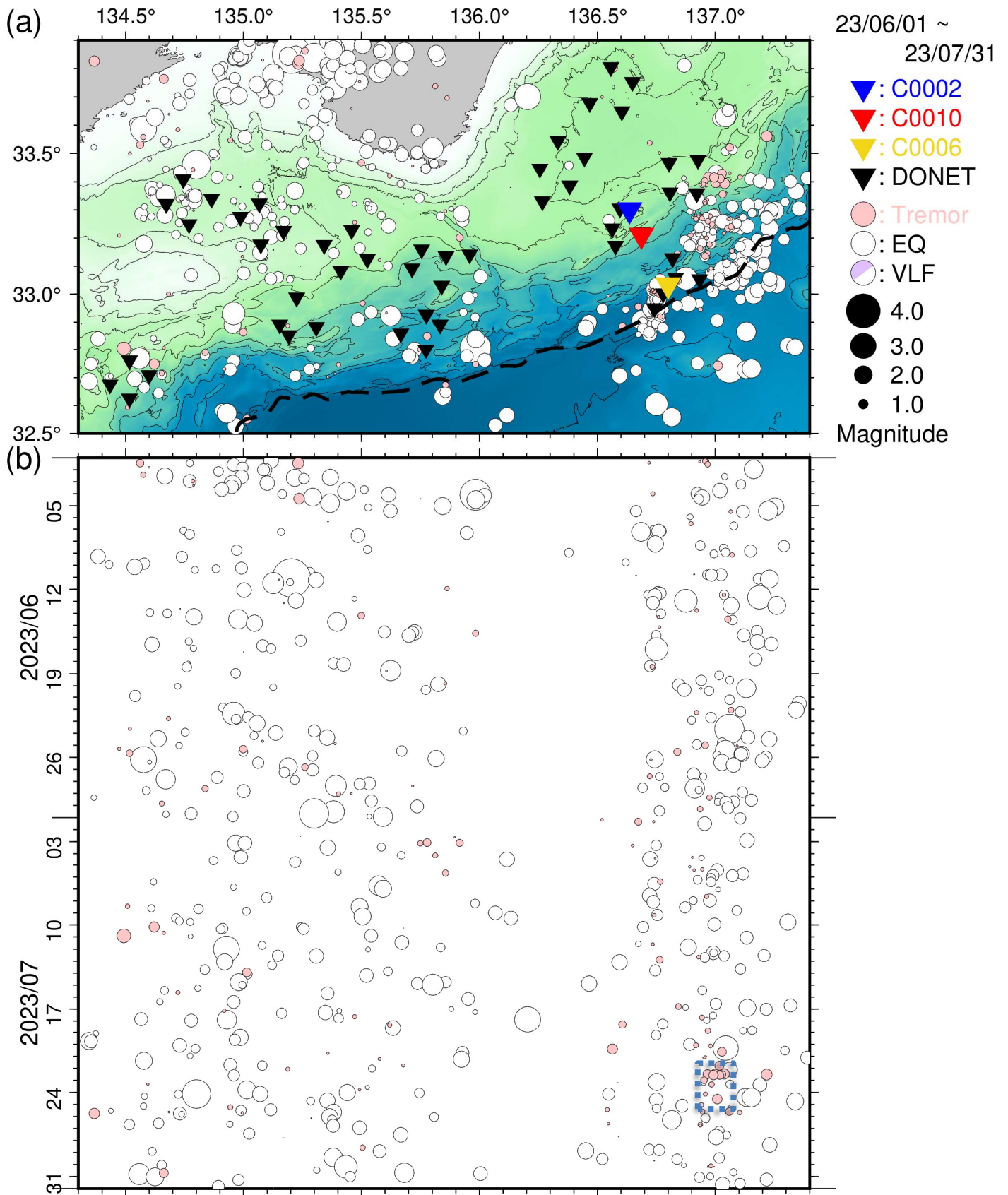
図5 直近2ヵ月間において熊野灘から室戸沖にて発生した低周波微動・通常地震・超低周波地震（2023年6月1日～2023年7月31日）。図3と同様のシンボルにて表示。(a) 震央分布図。(b) aに示した震央を経度方向へ投影した時空間分布図。青点線の長方形領域は、DONET1のBノード付近における低周波微動の群発的な活動を示す。
