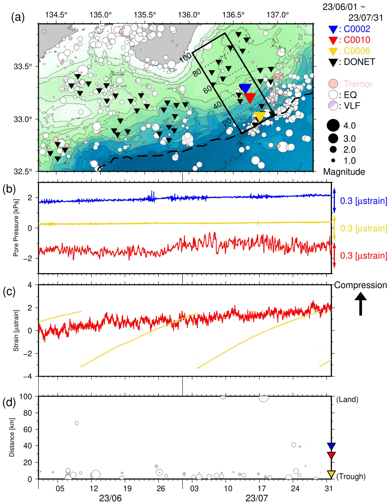
図3 直近2ヶ月間のSSE・低周波微動モニタリング(2023年6月1日~2023年7月31日)。(a)震央分布図(●:低周波微動(深さ0~15km)、○:通常地震(深さ0~60km)、●:超低周波地震のメカニズム解)。 ▼ ▼ ▼ ▼ は、それぞれC0002・C0010・C0006・DONET観測点。破線はトラフ軸。(b)長期孔内観測点における間隙水圧変化(—:C0002、—:C0010、—:C0006)。(c)長期孔内観測点における体積歪変化(—:C0010、—:C0006)。(d)図3a中に実線で示した矩形領域内における、低周波微動・通常地震・超低周波地震の時空間分布。縦軸は、トラフ軸からの距離(km)。
