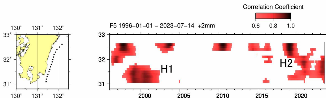
第1図 長期的スロースリップ客観検知図（1996年から2023年7月）
