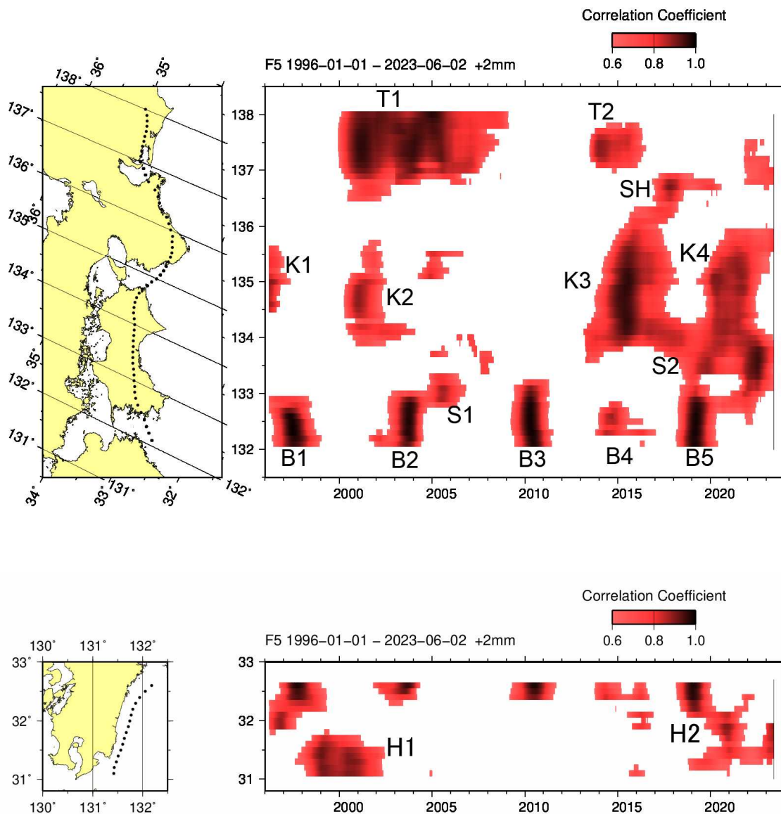
第1図 長期的スロースリップ客観検知図（1996年から2023年6月）
