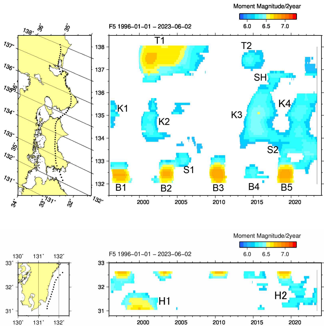
第2図 長期的スロースリップの規模分布（1996年から2023年6月） 2年間あたりの変化量から推定したモーメントマグニチュード。地域略号は第1図と同じ。
