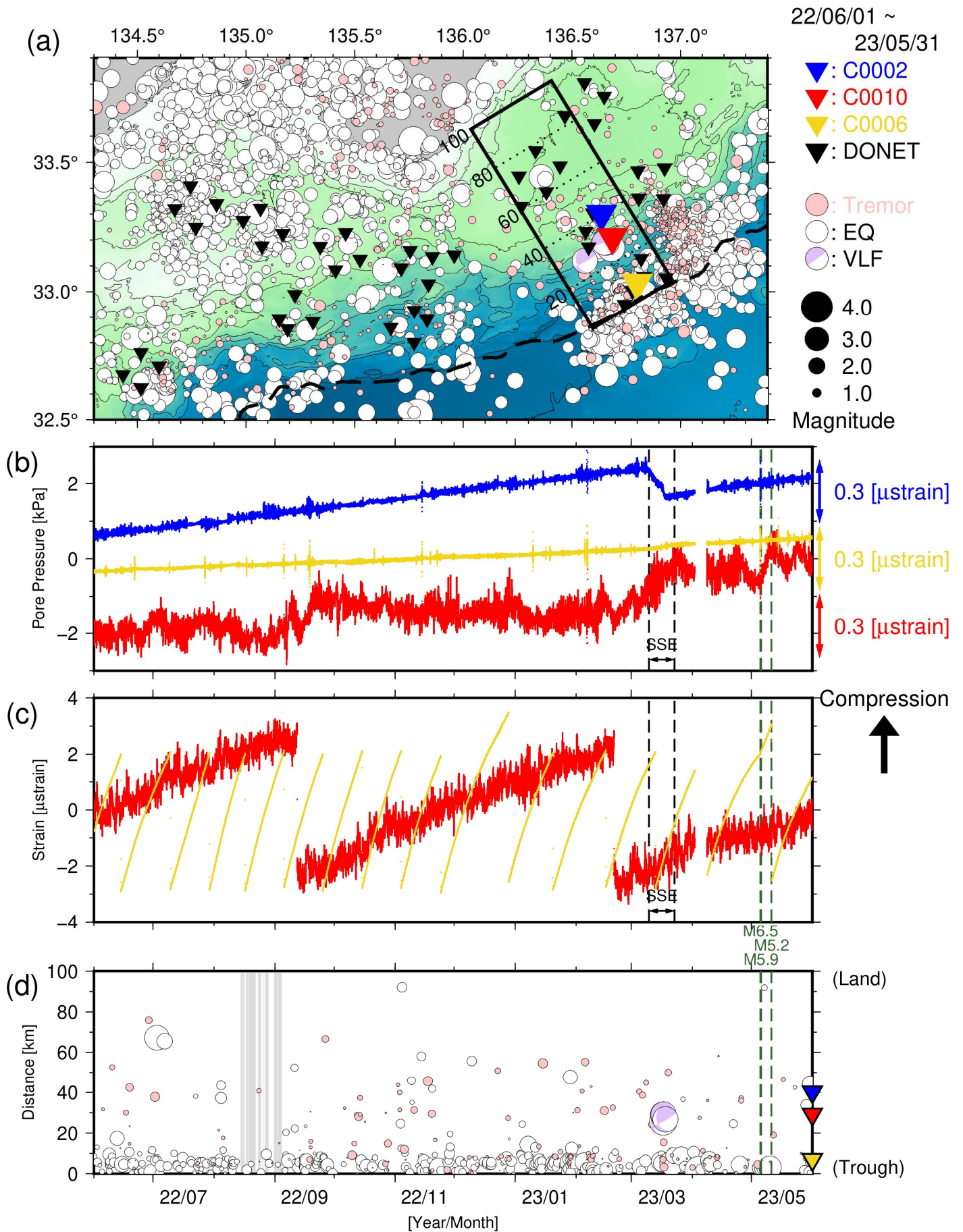
図4 直近1年間のSSE・低周波微動モニタリング(2022年6月1日~2023年5月31日)。(a)低周波微動・通常地震・超低周波地震の震央分布。(b)間隙水圧変化。(c)体積歪変化。(d)時空間分布。灰色はエアガン発振期間を示す。なお、図3において過去資料に緑点線で記した地震のうち、aの領域外かつM6.5未満のものは掲載していない。
