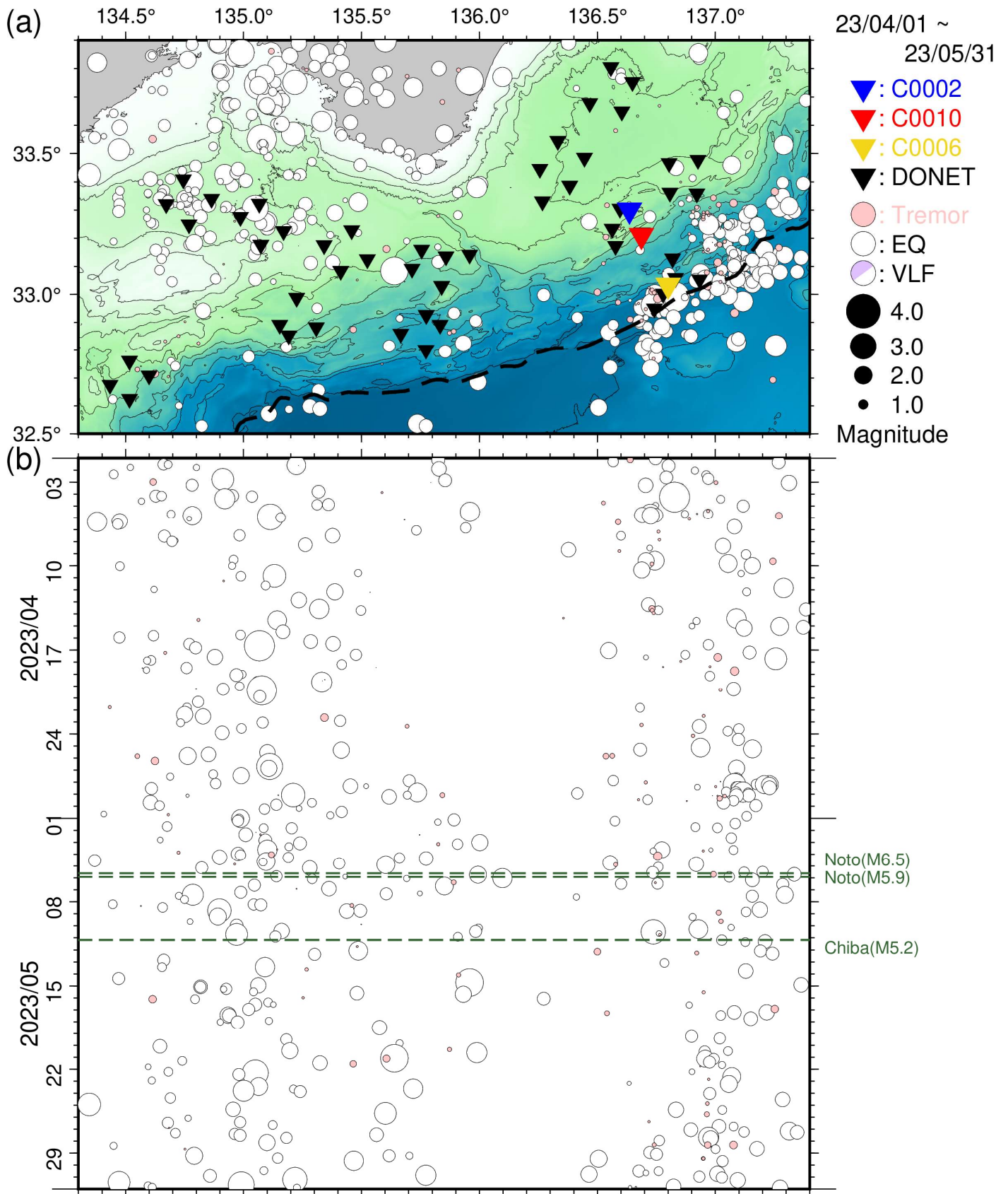
図5 直近2ヵ月間において熊野灘から室戸沖にて発生した低周波微動・通常地震・超低周波地震（2023年4月1日～2023年5月31日）。図3と同様のシンボルにて表示。(a) 震央分布図。(b) aに示した震央を経度方向へ投影した時空間分布図。
