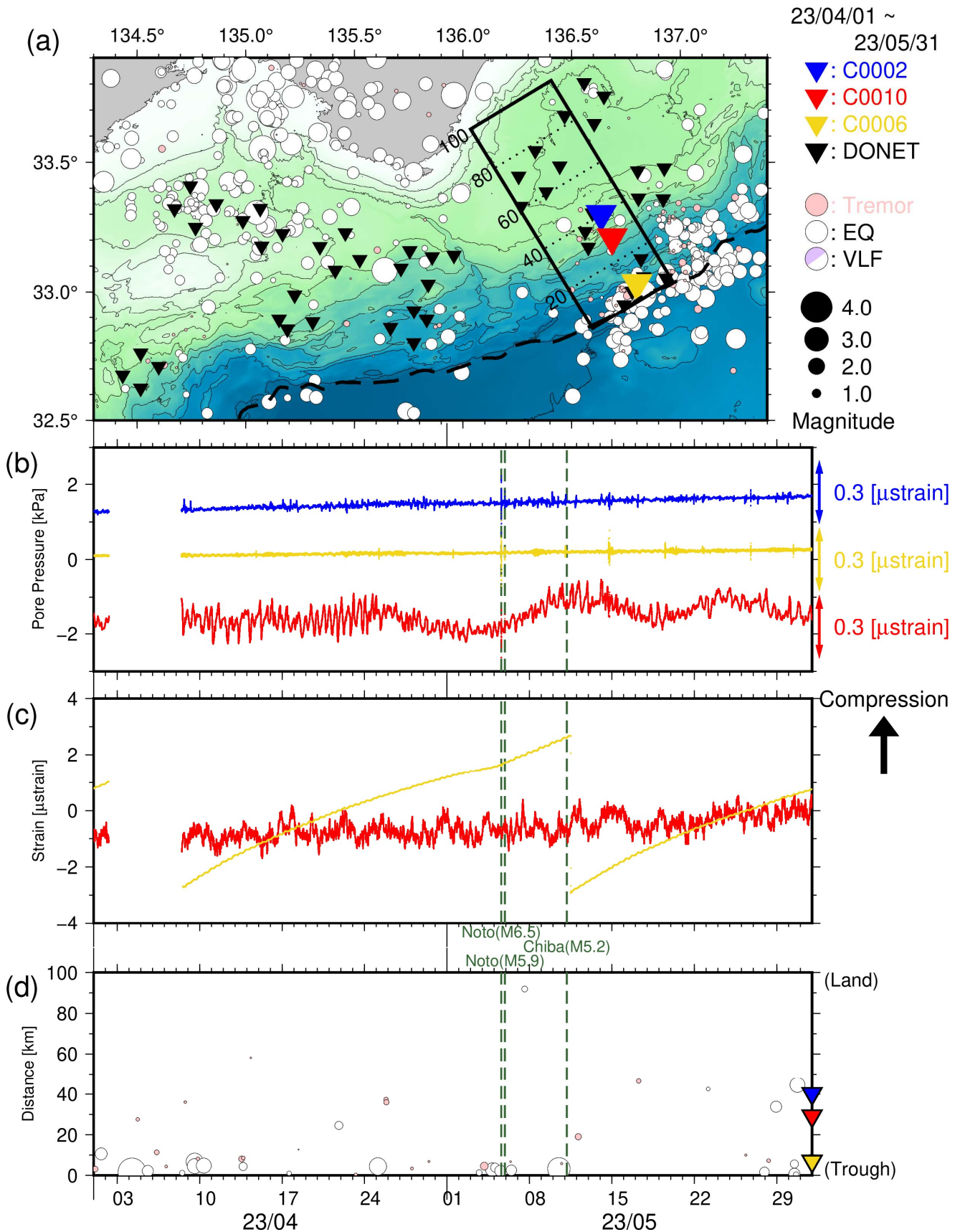
図3 直近2ヶ月間のSSE・低周波微動モニタリング(2023年4月1日~2023年5月31日)。(a)震央分布図(●:低周波微動(深さ0~15km)、○:通常地震(深さ0~60km)、●:超低周波地震のメカニズム解)。(b)長期孔内観測点における間隙水圧変化(—:C0002、—:C0010、—:C0006)。(c)長期孔内観測点における体積歪変化(—:C0010、—:C0006)。(d)図3a中に実線で示した矩形領域内における、低周波微動・通常地震・超低周波地震の時空間分布。縦軸は、トラフ軸からの距離(km)。
