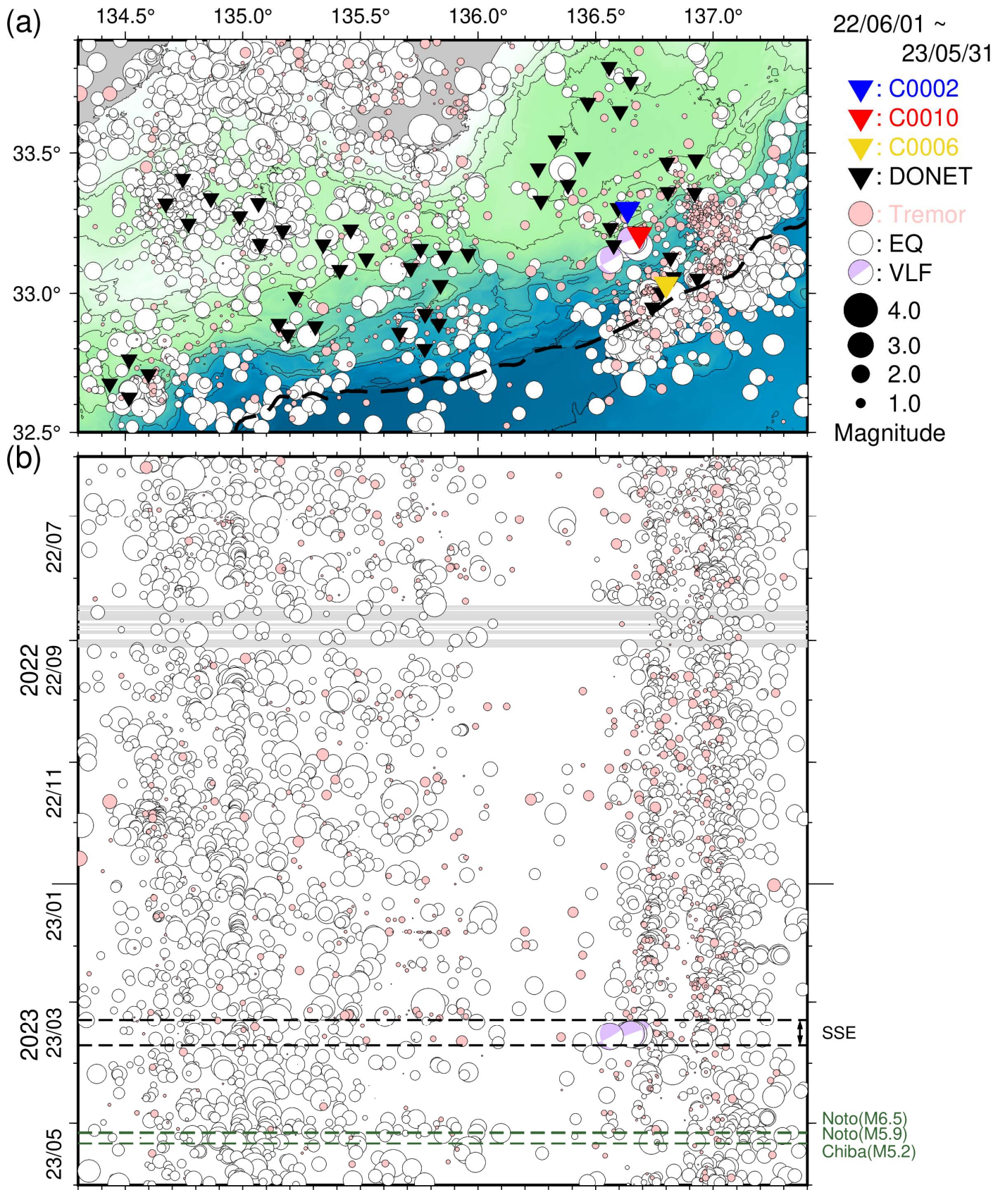
図 6 直近 1 年間に於いて熊野灘から室戸沖にて発生した低周波微動・通常地震・超低周波地震 (2022 年 6 月 1 日~2023 年 5 月 31 日)。図 4 と同様のシンボルにて表示。(a) 震央分布図。(b) a に示した震央を経度方向へ投影した時空間分布図。なお、図 3 および図 5 において過去資料に緑点線で記した地震のうち、a の領域外かつ M6.5 未満のものは掲載していない。
