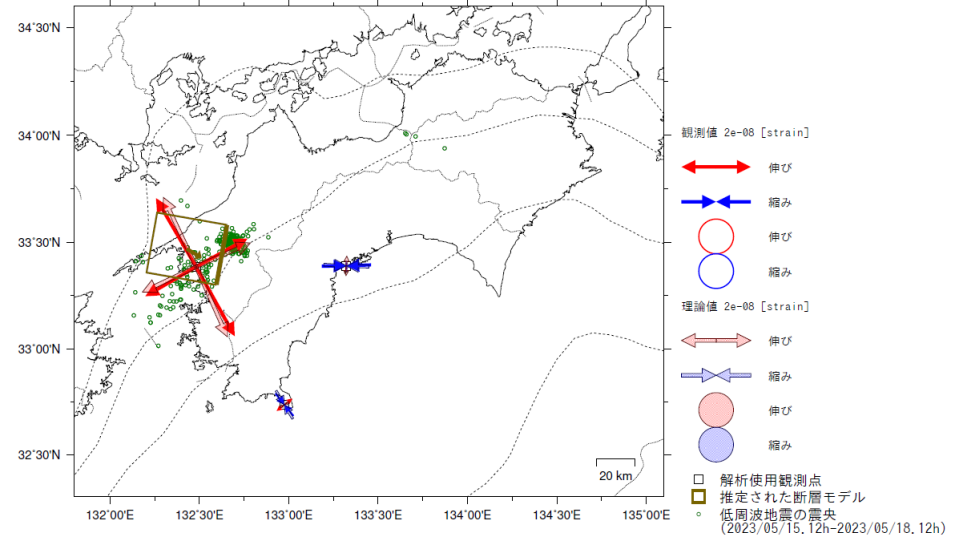
土佐清水松尾、西予宇和及び須崎大谷は産業技術総合研究所のひずみ・傾斜計である。
