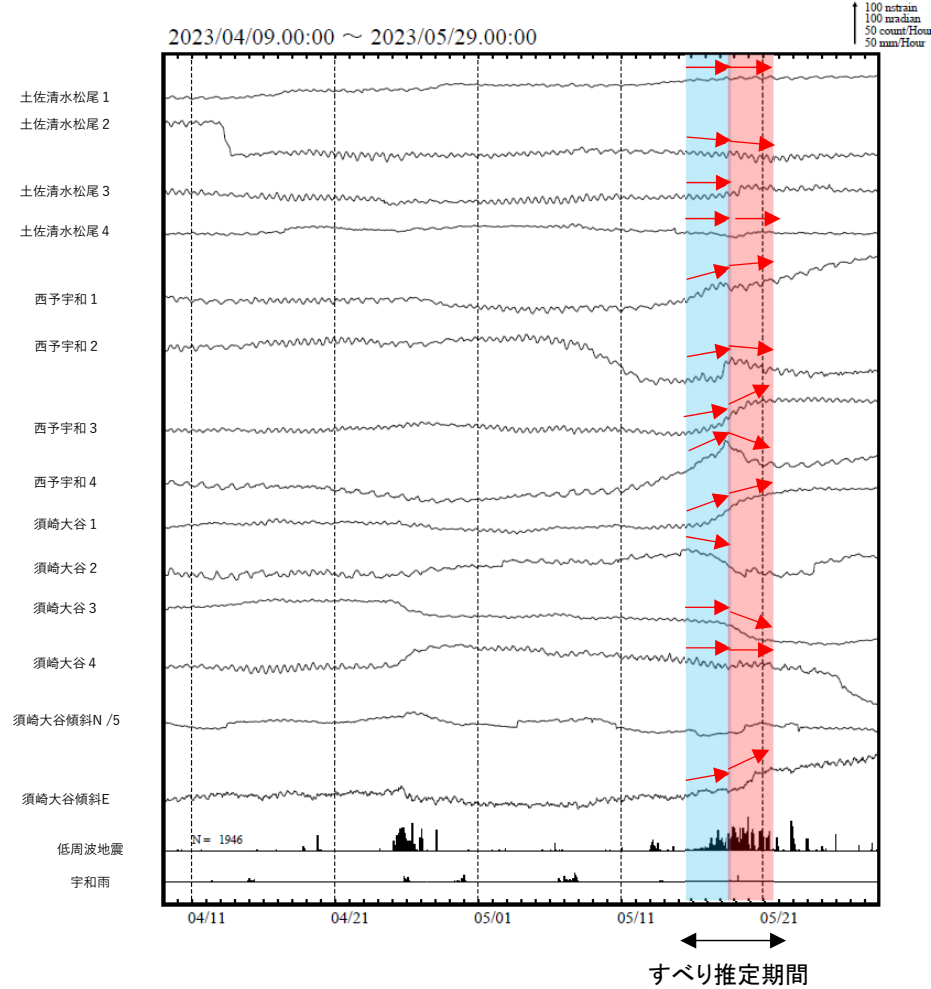
土佐清水松尾、西予宇和及び須崎大谷は産業技術総合研究所のひずみ・傾斜計である。
