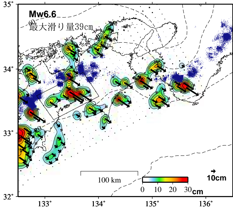
推定すべり分布 (2019/1/1-2023/5/10)
