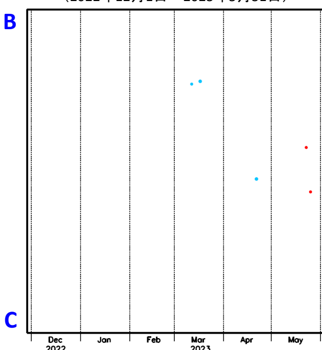
領域a内の時空間分布図(B-C投影) (2022年12月1日～2023年5月31日)
