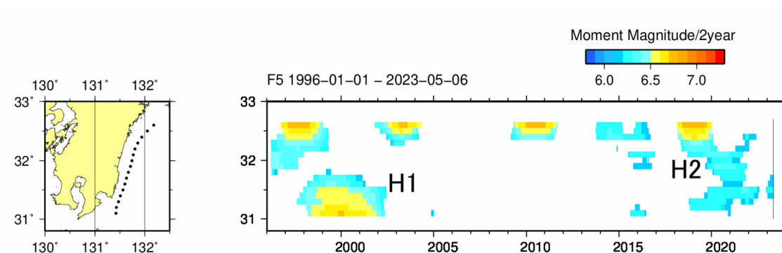
第2図 長期的スロースリップの規模分布（1996年から2023年5月） 2年間あたりの変化量から推定したモーメントマグニチュード。地域略号は第1図と同じ。
