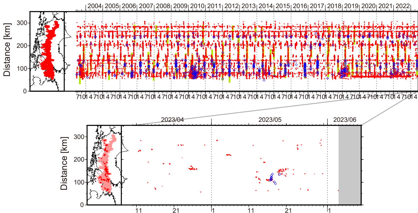
図1. 四国における2003年6月～2023年6月3日までの深部低周波微動の時空間分布(上図). 赤丸はエンベロープ相関・振幅ハイブリッド法 (Maeda and Obara, 2009) およびクラスタ処理 (Obara et al., 2010) によって1時間毎に自動処理された微動分布の重心である. 青菱形は周期20秒に卓越する超低周波地震 (Ito et al., 2007) である. 黄緑色太線は、これまでに検出された短期的スロースリップイベント (SSE) を示す. 下図は2023年5月を中心とした期間の拡大図である. 5月18～22日頃には愛媛県西部において、やや活発な活動がみられ、東西方向への活動域の拡大が若干みられた. この活動に際し、傾斜変動から短期的SSEの断層モデルも推定されている. 5月5～6日頃には愛媛県東部において、5月12～14日頃および5月15～17日頃には愛媛県西部において、5月23～25日頃には愛媛・香川・徳島県境付近において、それぞれ小規模な活動がみられた. 5月14～15日頃には愛媛県東部において、5月30日頃には香川県付近において、それぞれごく小規模な活動がみられた.
