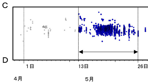
震央分布図の領域a内の時空間分布図 (C-D投影、2023年4月29日~5月27日)
