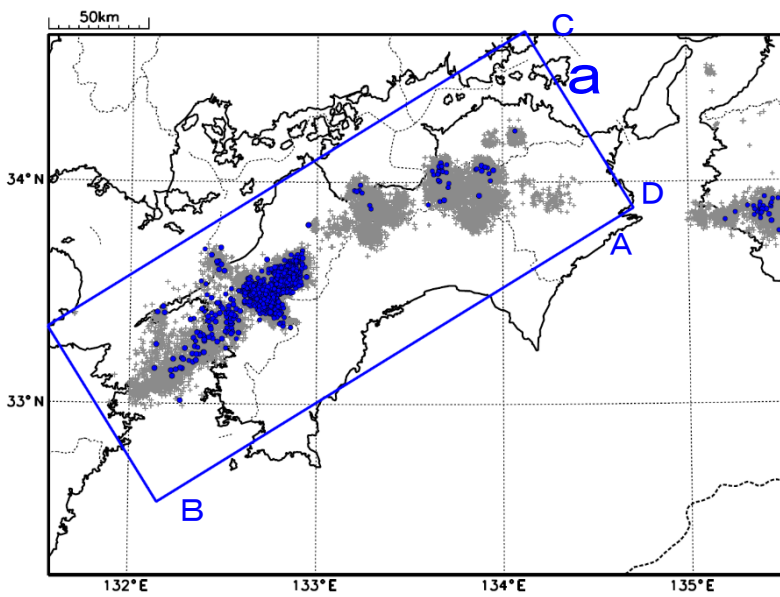
震央分布図(2018年4月1日~2023年5月27日、 深さ0~60km、Mすべて) 灰:2018年4月1日~2023年5月12日、 青:2023年5月13日以降
