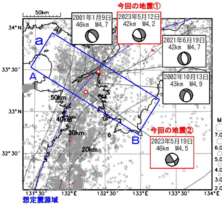
震央分布図 (1997年10月1日～2023年5月31日、 深さ0～80km、 M \geq 2.0 ) 2023年5月12日以降の地震を赤色で表示
