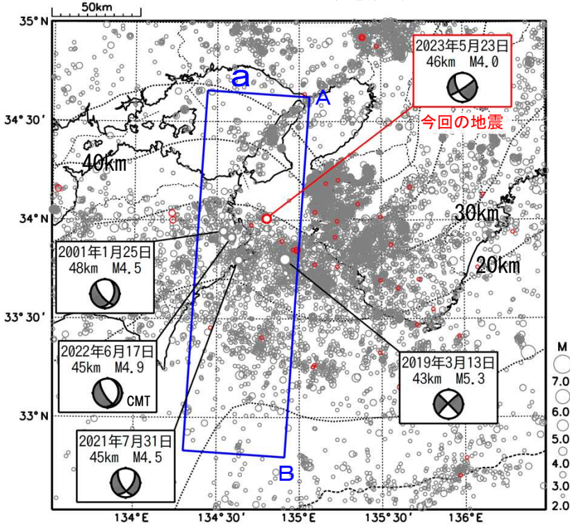
震央分布図 (1997年10月1日～2023年5月31日、 深さ0～60km、 M \geq 2.0 ) 2023年5月1日以降の地震を赤く表示
