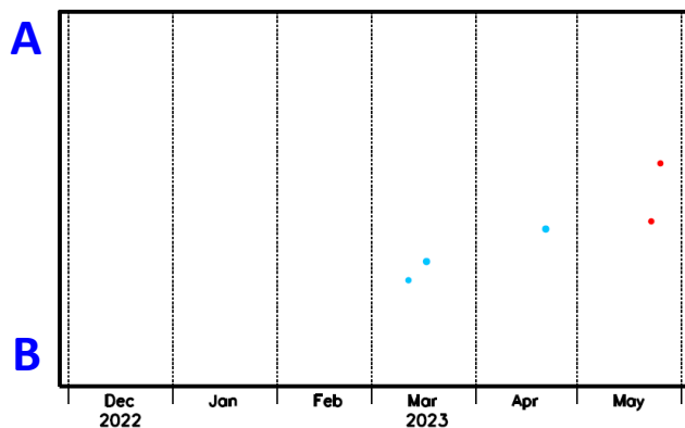
領域a内の時空間分布図(A-B投影) (2022年12月1日～2023年5月31日)
