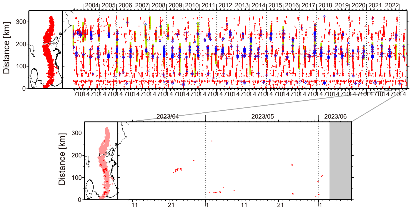
図1. 紀伊半島・東海地域における2003年6月～2023年6月3日までの深部低周波微動の時空間分布(上図). 赤丸はエンベロープ相関・振幅ハイブリッド法 (Maeda and Obara, 2009) およびクラスタ処理 (Obara et al., 2010) によって1時間毎に自動処理された微動分布の重心である. 青菱形は周期20秒に卓越する超低周波地震 (Ito et al., 2007) である. 黄緑色の太線はこれまでに検出された短期的スロースリップイベント (SSE) を示す. 下図は2023年5月を中心とした期間の拡大図である. この期間に顕著な活動はとくにみられなかったものの, 5月3～5日頃および5月24～25日頃には和歌山県中部において, 5月31日～6月2日頃には, 奈良県南部から奈良・三重県境付近において, それぞれごく小規模な活動がみられた.
