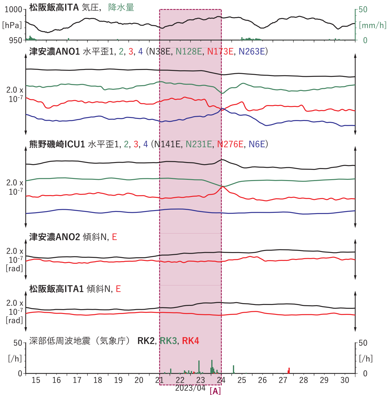
図8 歪・傾斜の時間変化(1) (2023/04/15 00:00-2023/05/01 00:00 (JST))
