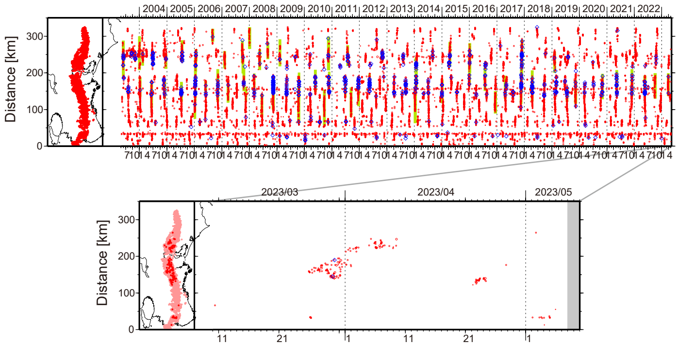
図1. 紀伊半島・東海地域における2003年5月～2023年5月7日までの深部低周波微動の時空間分布(上図). 赤丸はエンベロップ相関・振幅ハイブリッド法(Maeda and Obara, 2009)およびクラスタ処理(Obara et al., 2010)によって1時間毎に自動処理された微動分布の重心である. 青菱形は周期20秒に卓越する超低周波地震(Ito et al., 2007)である. 黄緑色の太線はこれまでに検出された短期的スロースリップイベント(SSE)を示す. 下図は2023年4月を中心とした期間の拡大図である. 3月25日～4月9日頃には三重県北部から愛知県西部で活発な微動活動がみられた. この活動は三重県北部で開始したのち, プレート境界の浅部側への活動域の移動がみられた. さらに北東方向への活動域の拡大がみられ, 4月1日頃からは, 愛知県西部において活動が開始した. この活動に際し, 傾斜変動から短期的SSEの断層モデルも推定されている. 4月22～24日頃には三重・奈良県境付近において, 小規模な活動がみられた. 5月3～5日頃には和歌山県中部において, ごく小規模な活動がみられた.
