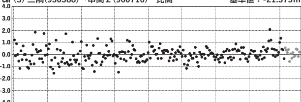
cm (3) 三隅(950388)→串間2(960716) 比高 基準値: -21.375m
