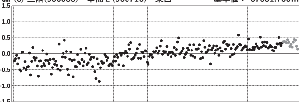
cm (3) 三隅(950388)→串間2(960716) 南北 基準値: -373521.185m
