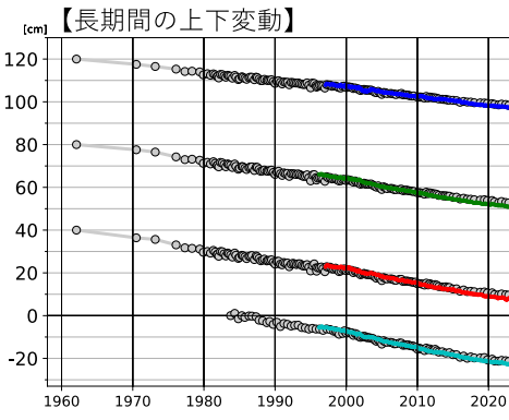
【長期間の上下変動】
