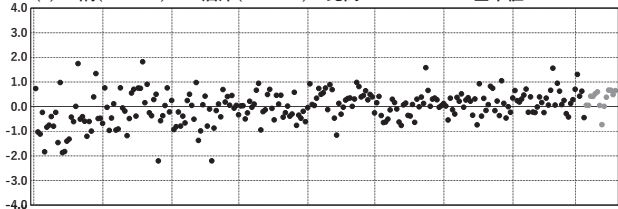
cm (4) 三隅(950388)→P油津(02P211) 比高 基準値: -28.852m
