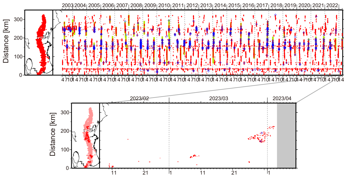
図1. 紀伊半島・東海地域における2003年4月～2023年4月3日までの深部低周波微動の時空間分布(上図). 赤丸はエンベロップ相関・振幅ハイブリッド法(Maeda and Obara, 2009)およびクラスタ処理(Obara et al., 2010)によって1時間毎に自動処理された微動分布の重心である. 青菱形は周期20秒に卓越する超低周波地震(Ito et al., 2007)である. 黄緑色の太線はこれまでに検出された短期的スロースリップイベント(SSE)を示す. 下図は2023年3月を中心とした期間の拡大図である. 3月25日頃から三重県北部で微動活動が開始したのち、プレート境界の浅部側への活動域の移動がみられた. さらに北東方向への活動域の拡大がみられ、4月1日頃からは、愛知県西部において活動がみられている. この活動に際し、傾斜変動から短期的SSEの断層モデルも推定されている. 3月7～10日頃には、奈良県南部において小規模な活動が、3月26日頃には、和歌山県中部においてごく小規模な活動がみられた. 3月9日17:17頃に紀伊水道南部(深さ45km)で発生したM3.8(Hi-net暫定値)の後、17:20台に和歌山県中部で微動活動がみられ、クラスタリング処理結果でも微動源が推定されている.
