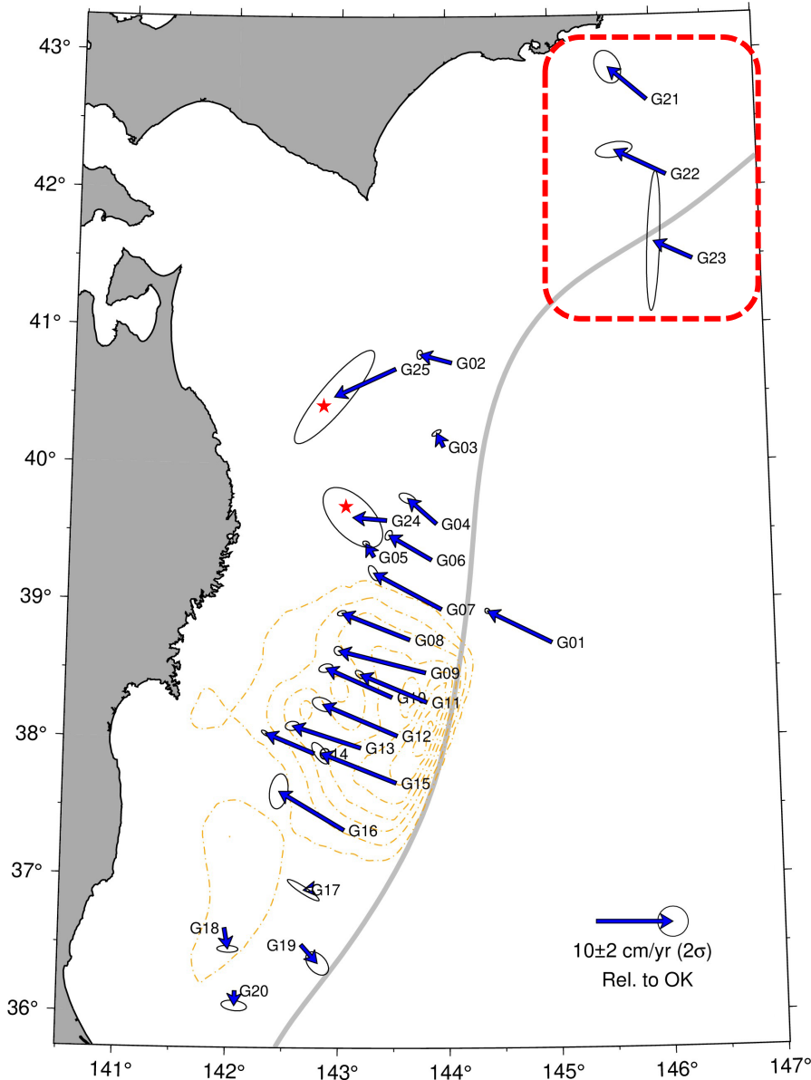
2012/09–2022/10 でのGNSS-A変位速度 (2σ誤差楕円) 橙色コンター：Iinuma et al. (2012)による2011年東北沖地震時すべりモデル
