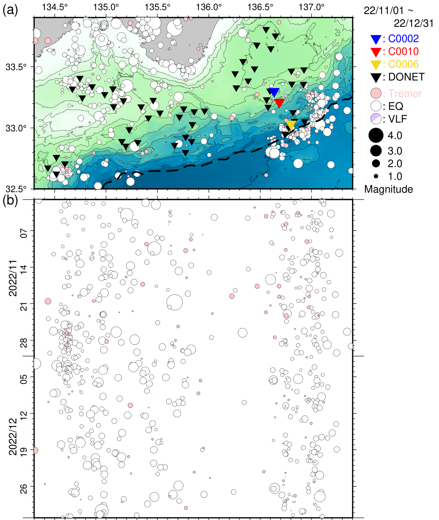
図5 直近2ヵ月間において熊野灘から室戸沖にて発生した低周波微動・通常地震・超低周波地震 (2022年11月1日~2022年12月31日)。図3と同様のシンボルにて表示。(a) 震央分布図。(b) aに示した震央を経度方向へ投影した時空間分布図。
