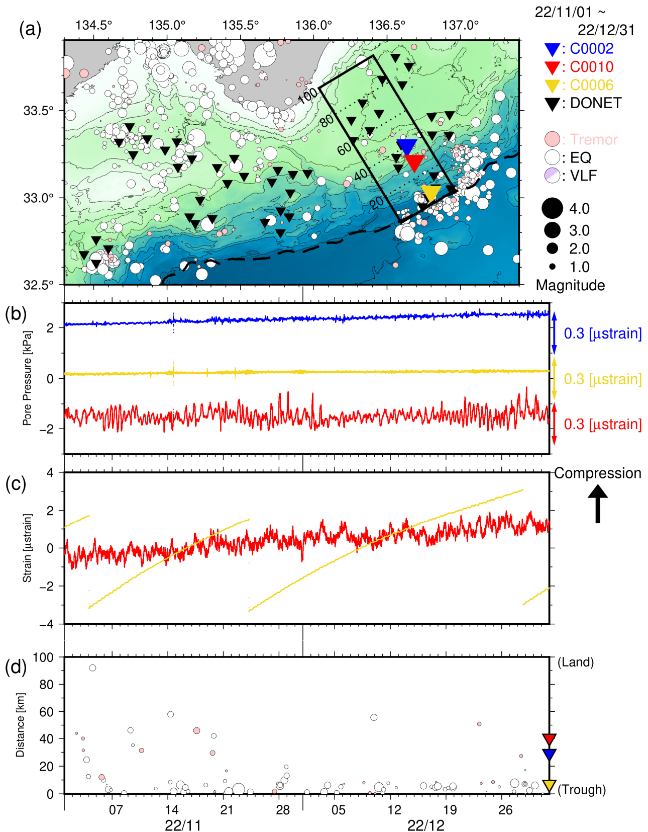
図3 直近2ヶ月間のSSE・低周波微動モニタリング(2022年11月1日~2022年12月31日)。 (a) 震央分布図(●:低周波微動(深さ0~15km)、○:通常地震(深さ0~60km)、●:超低周波地震のメカニズム解)。▼▼▼は、それぞれC0002・C0010・C0006・DONET観測点。破線はトラフ軸。(b) 長期孔内観測点における間隙水圧変化(—:C0002、—:C0010、—:C0006)。(c) 長期孔内観測点における体積歪変化(—:C0010、—:C0006)。(d) 図3a中に実線で示した矩形領域内における、低周波微動・通常地震・超低周波地震の時空間分布。灰色はエアガン発振期間。縦軸は、トラフ軸からの距離(km)。
