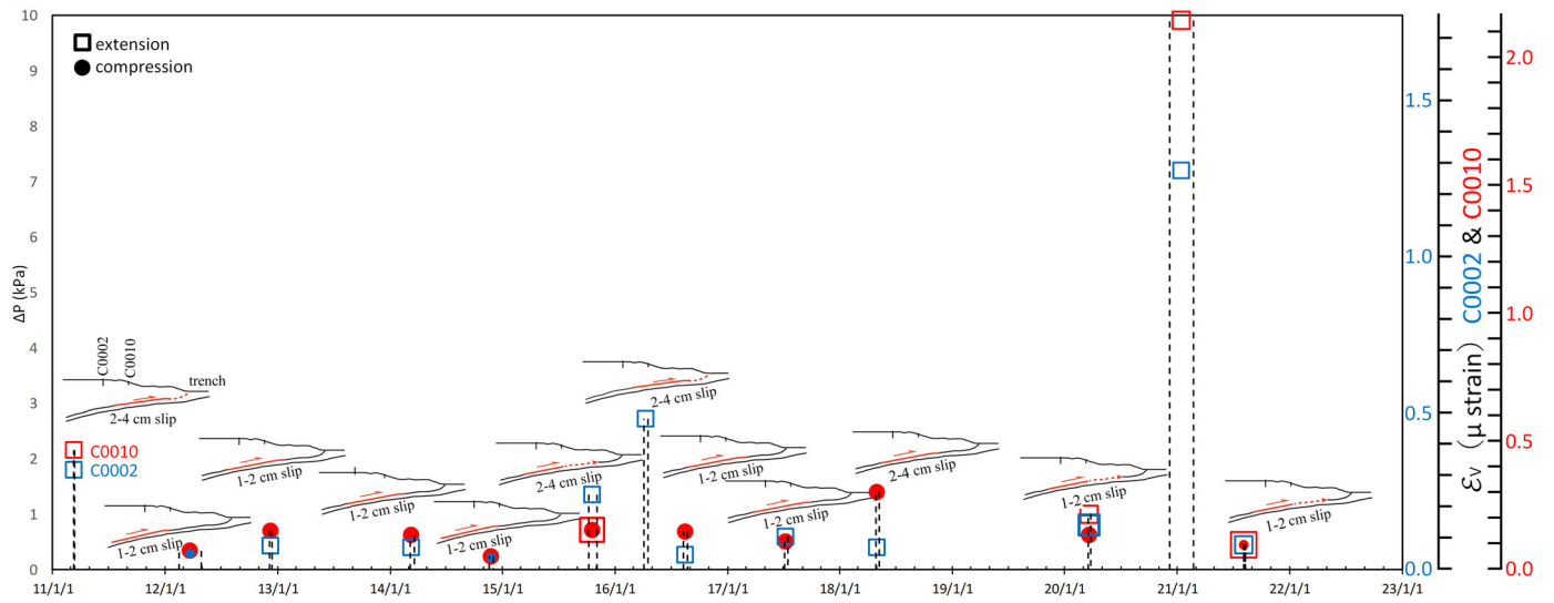
図7 孔内観測点において観測された SSE 発生時の間隙水圧変化 (Araki et al., 2017; Ariyoshi et al. 2021a を加筆・修正)。間隙水圧変化 ( \Delta P ) とそれらを体積歪 ( \epsilon_v ) に換算したスケールを縦軸に示している。●・□は、それぞれ圧縮・伸長方向の間隙水圧変化を示す。青・赤のシンボルは、それぞれ C0002・C0010 の間隙水圧変化を示す。
