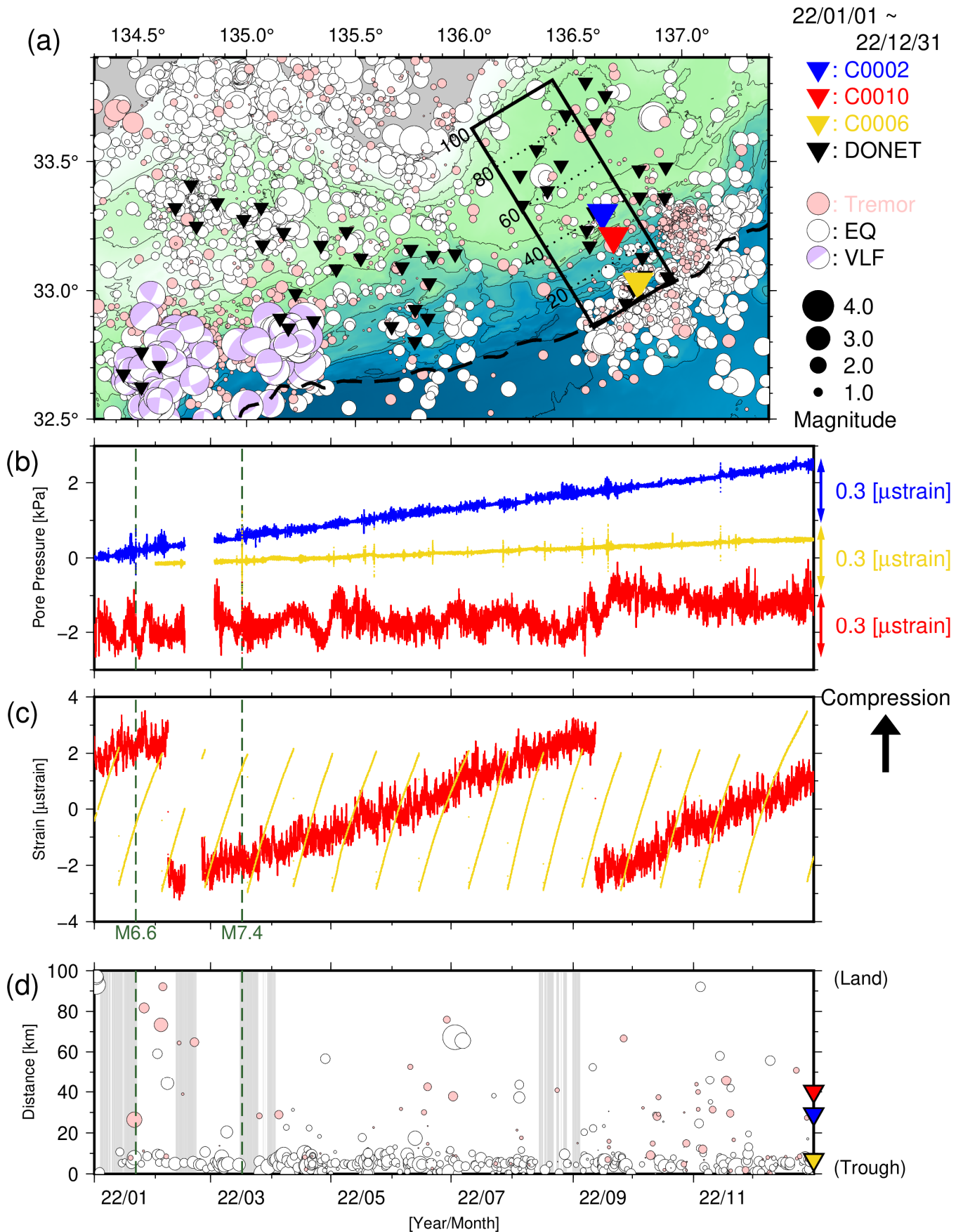
図4 直近1年間のSSE・低周波微動モニタリング(2022年1月1日~2022年12月31日)。(a)低周波微動・通常地震・超低周波地震の震央分布。(b)間隙水圧変化。(c)体積歪変化。(d)時空間分布。灰色はエアガン発振期間を示す。(b-d)の緑点線は、1月22日日向灘地震、及び3月16日福島県沖地震。なお、図3において過去資料に緑点線で記した地震のうち、aの領域外かつM6.5未満のものは掲載していない。
