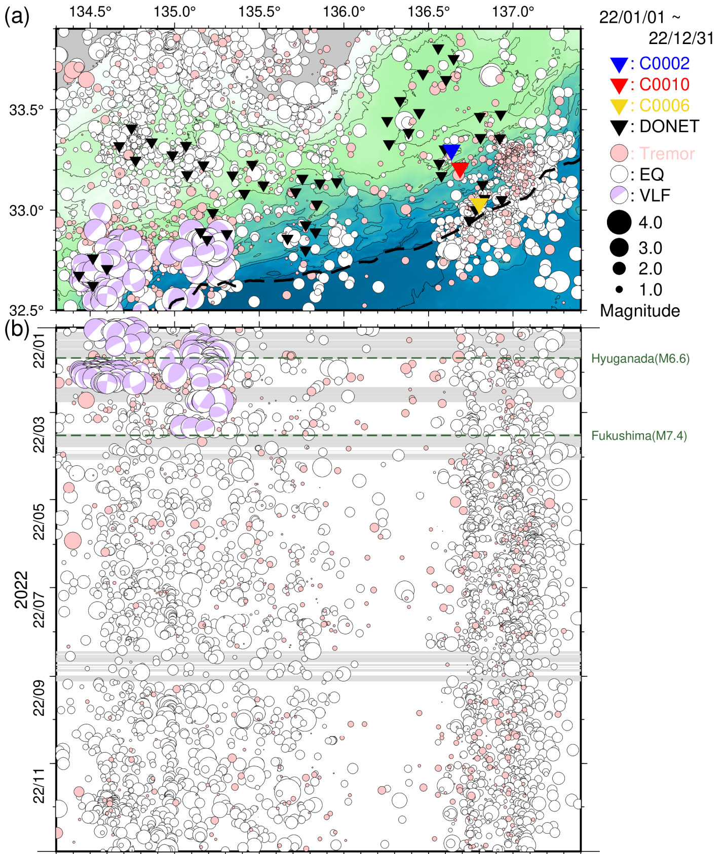
図 6 直近 1 年間に於いて熊野灘から室戸沖にて発生した低周波微動・通常地震・超低周波地震 (2022 年 1 月 1 日~ 2022 年 12 月 31 日)。図 4 と同様のシンボルにて表示。(a) 震央分布図。(b) a に示した震央を経度方向へ投影した時空間分布図。なお、図 3 および図 5 において過去資料に緑点線で記した地震のうち、a の領域外かつ M6.5 未満のものは掲載していない。
