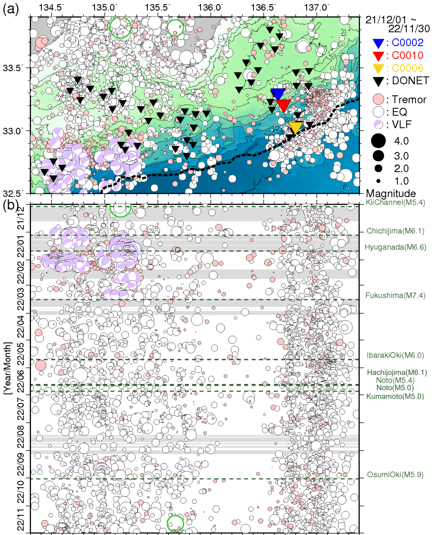
図 6 直近 1 年間に於いて熊野灘から室戸沖にて発生した低周波微動・通常地震・超低周波地震 (2021 年 12 月 1 日~2022 年 11 月 30 日)。図 4 と同様のシンボルにて表示。(a) 震央分布図。(b) a に示した震央を経度方向へ投影した時空間分布図。
