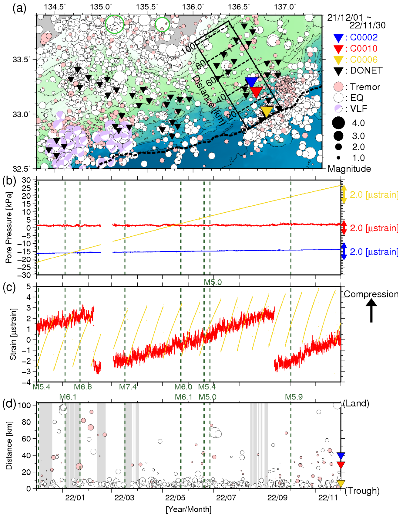
図4 直近1年間のSSE・低周波微動モニタリング(2021年12月1日~2022年11月30日)。(a)低周波微動・通常地震・超低周波地震の震央分布。(b)間隙水圧変化。(c)体積歪変化。(d)時空間分布。灰色はエアガン発振期間を示す。(b-d)の緑点線は、12月3日紀伊水道地震、1月4日父島近海地震、1月22日日向灘地震、3月16日福島県沖地震、5月22日茨城県沖地震、5月23日八丈島東方沖地震、6月19日・20日能登地方地震、6月26日熊本地方地震、及び10月2日大隅半島東方沖地震。
