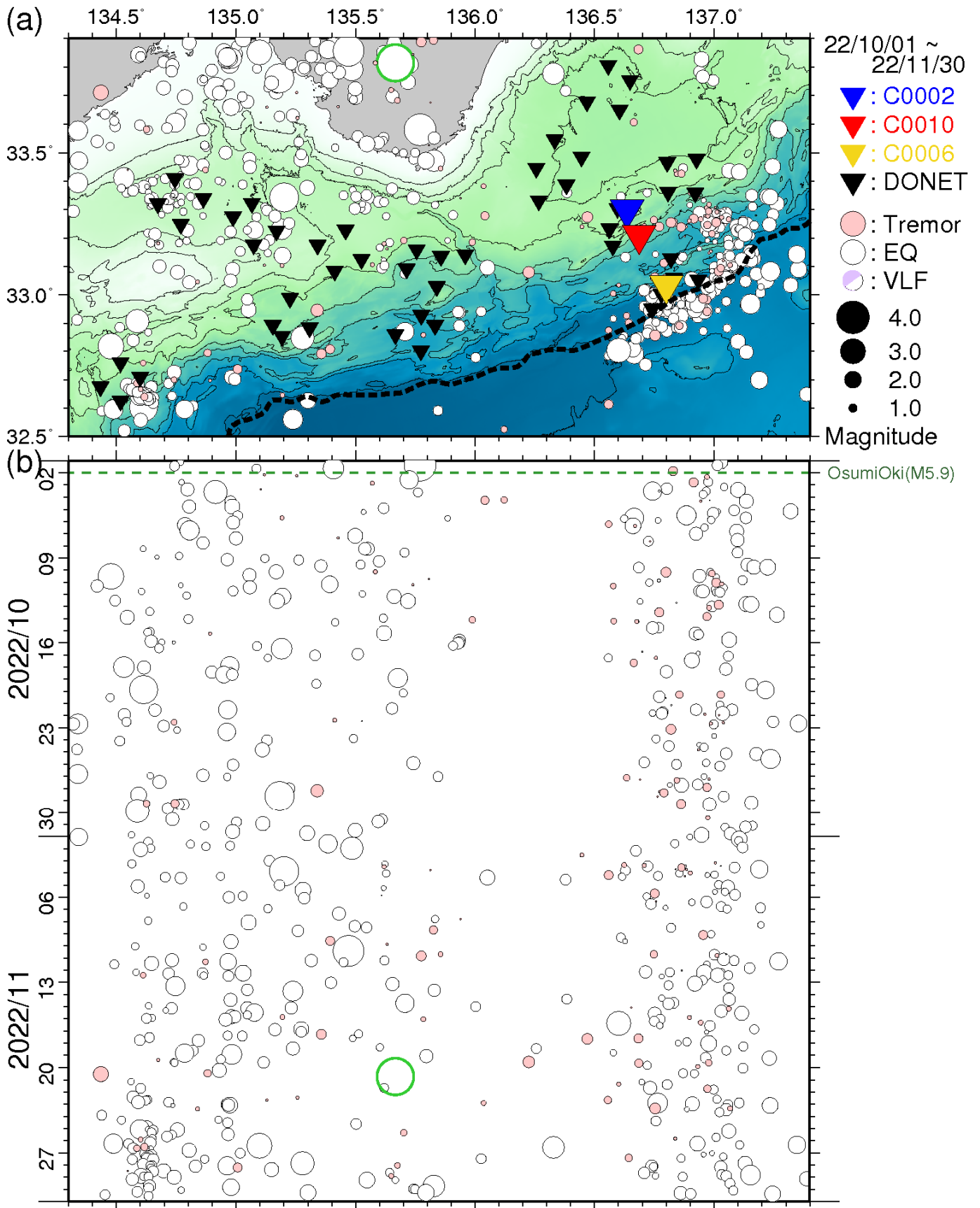
図5 直近2ヵ月間において熊野灘から室戸沖にて発生した低周波微動・通常地震・超低周波地震(2022年10月1日~2022年11月30日)。図3と同様のシンボルにて表示。(a)震央分布図。(b)aに示した震央を経度方向へ投影した時空間分布図。
