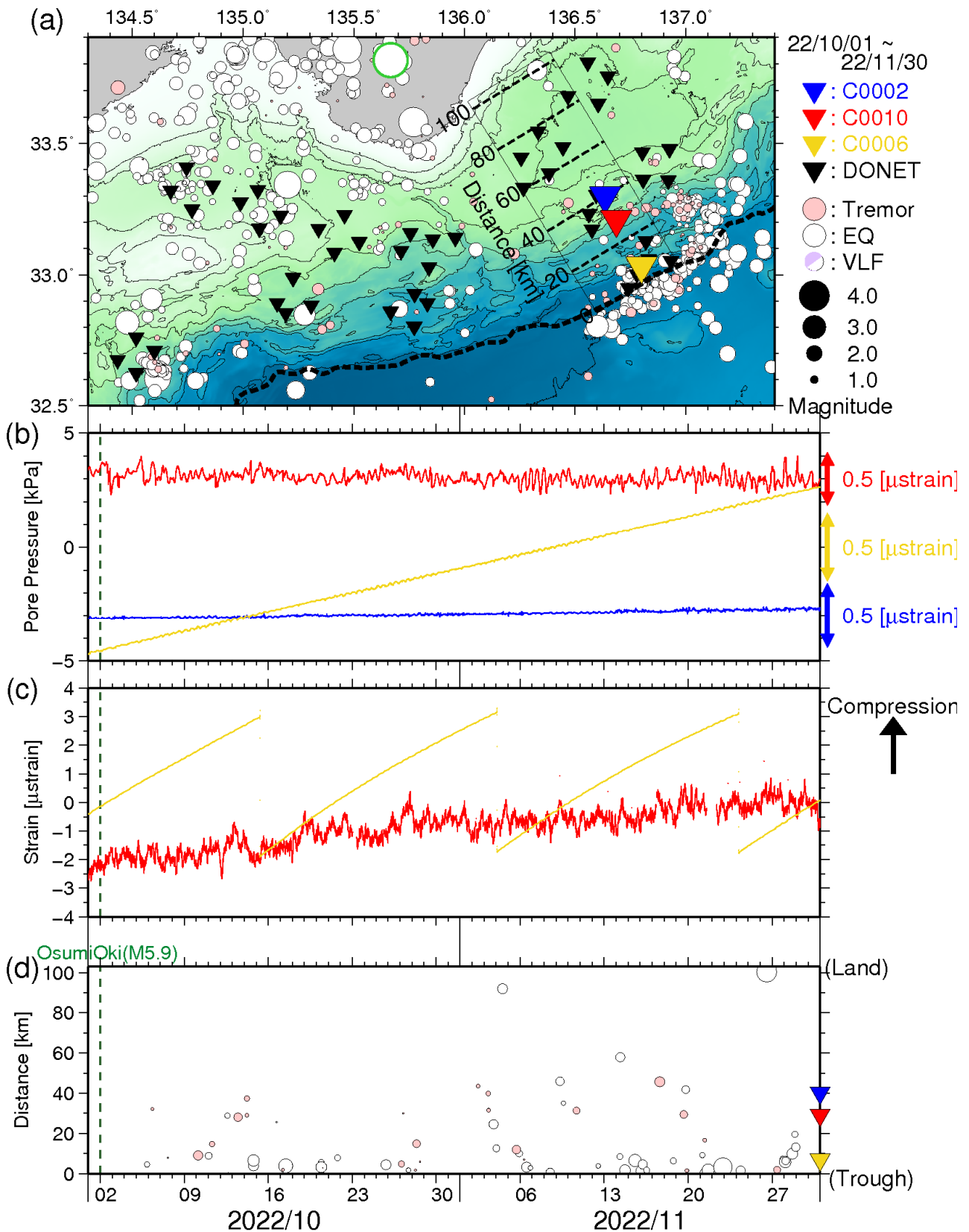
図3 直近2ヶ月間のSSE・低周波微動モニタリング(2022年10月1日~2022年11月30日)。 (a) 震央分布図(●:低周波微動(深さ0~15km)、○:通常地震(深さ0~60km)、●:超低周波地震のメカニズム解)。▼▼▼は、それぞれC0002・C0010・C0006・DONET観測点。破線はトラフ軸。(b) 長期孔内観測点における間隙水圧変化(—:C0002、—:C0010、—:C0006)。(c) 長期孔内観測点における体積歪変化(—:C0010、—:C0006)。(d) 図3a中に実線で示した矩形領域内における、低周波微動・通常地震・超低周波地震の時空間分布。灰色はエアガン発振期間。縦軸は、トラフ軸からの距離(km)。(b-d)の緑点線は、10月2日大隅半島東方沖地震を示す。
