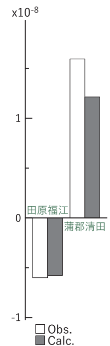
図13 2022/10/11PM-15 の歪・傾斜変化 (図10, 11, 12 [A]) を説明する断層モデル。
