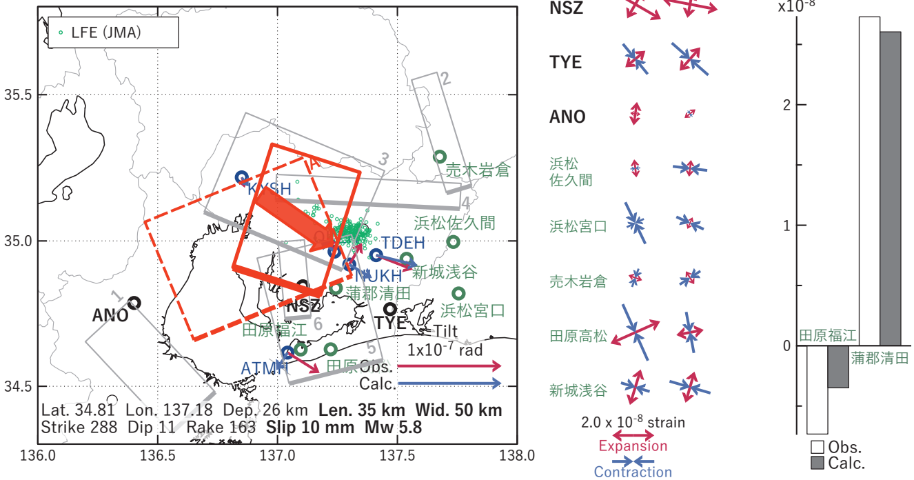
図14 2022/10/16-18の歪・傾斜変化 (図10, 11, 12 [B]) を説明する断層モデル。
