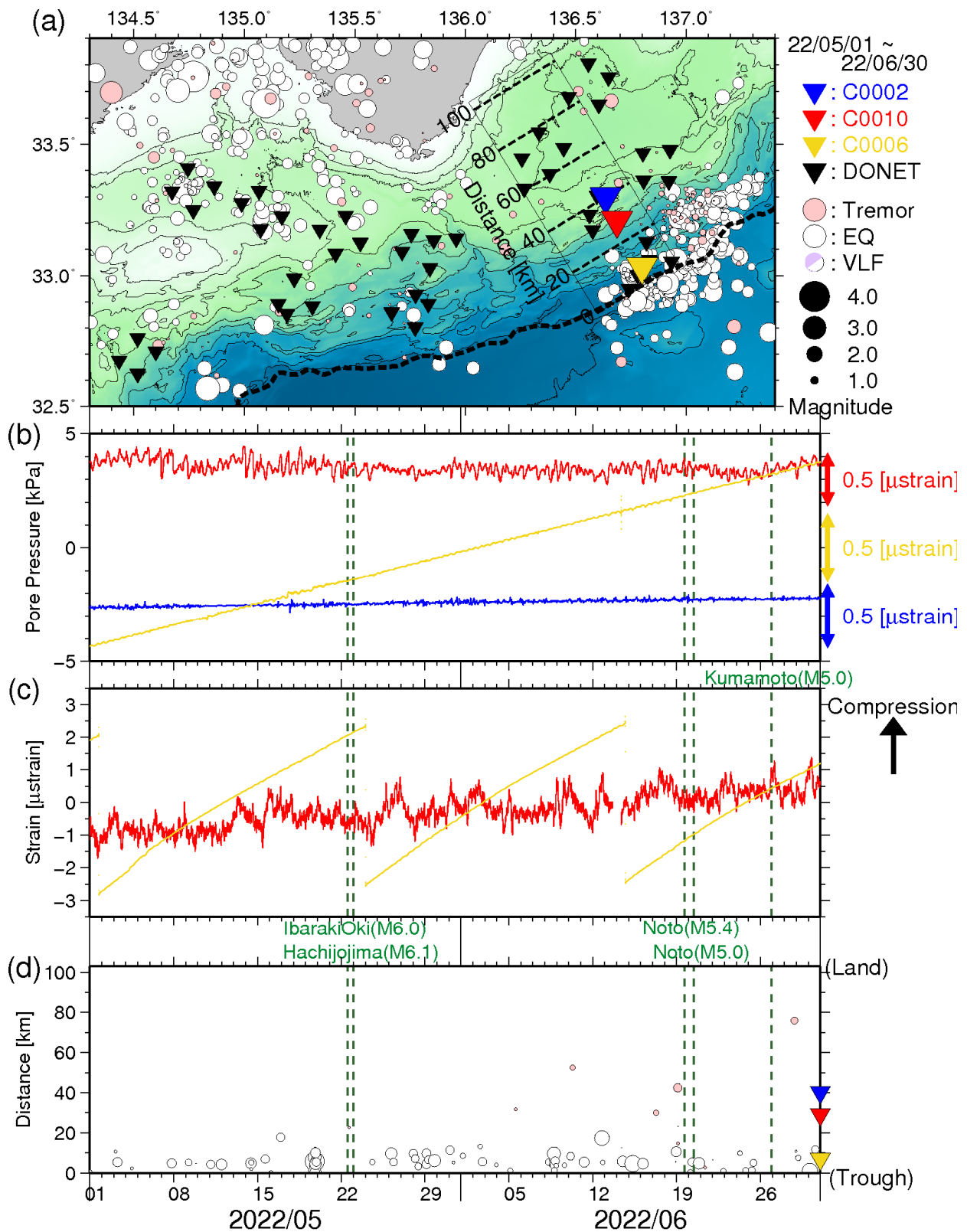
図3 直近2ヶ月間のSSE・低周波微動モニタリング(2022年5月1日~2022年6月30日)。(a) 震央分布図(●:低周波微動(深さ0~15km)、○:通常地震(深さ0~60km)、●:超低周波地震のメカニズム解)。▼、▼、▼、▼は、それぞれC0002・C0010・C0006・DONET観測点。破線はトラフ軸。(b)長期孔内観測点における間隙水圧変化(—:C0002、—:C0010、—:C0006)。(c)長期孔内観測点における体積歪変化(—:C0010、—:C0006)。(d)図3a中に実線で示した矩形領域内における、低周波微動・通常地震・超低周波地震の時空間分布。灰色はエアガン発振期間。縦軸は、トラフ軸からの距離(km)。(b-d)の緑点線は、5月22日茨城県沖地震、5月23日八丈島東方沖地震、6月19日・20日能登地方地震、及び6月26日熊本地方地震。
