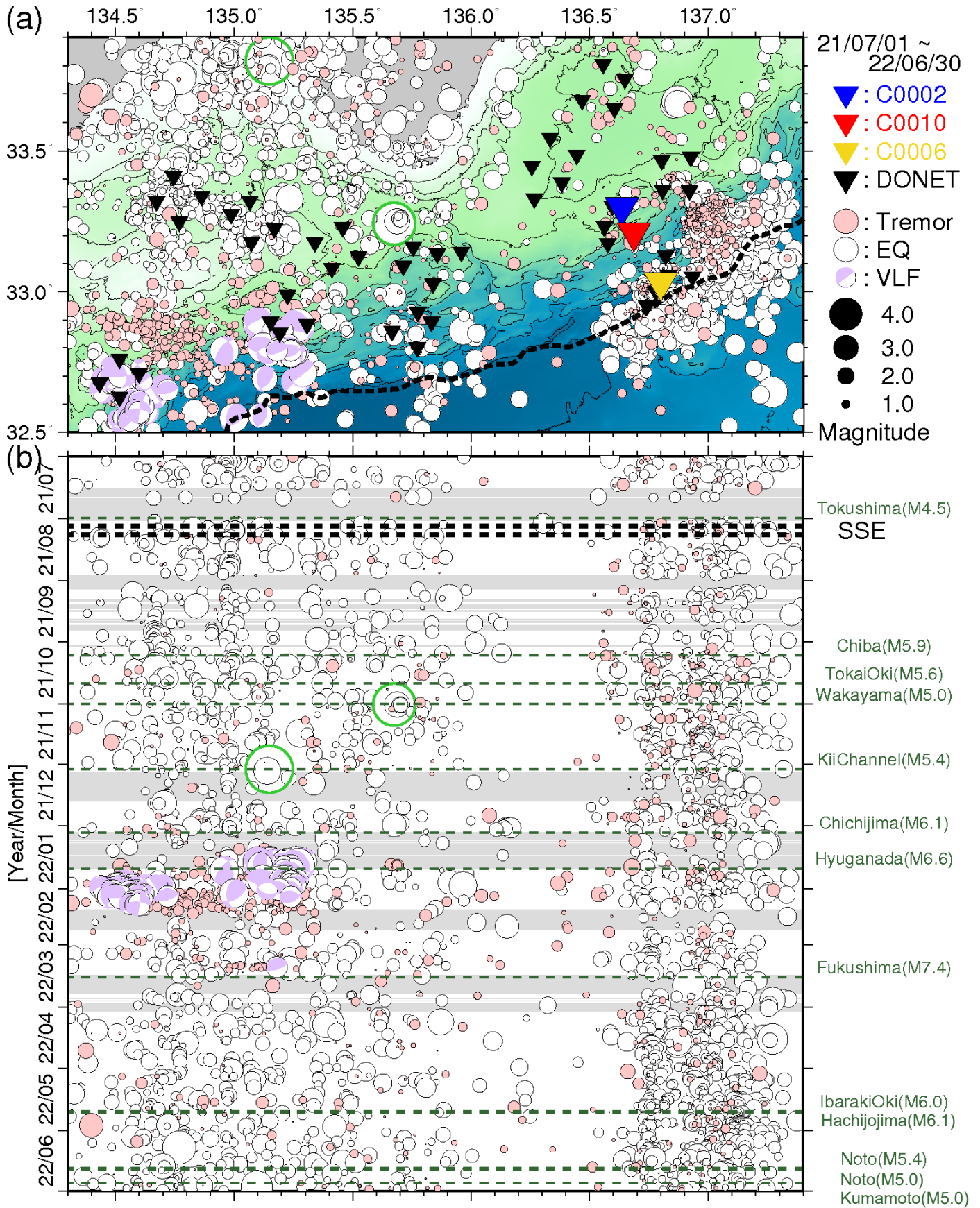
図 6 直近 1 年間に於いて熊野灘から室戸沖にて発生した低周波微動・通常地震・超低周波地震 (2021 年 7 月 1 日~2022 年 6 月 30 日)。図 4 と同様のシンボルにて表示。(a) 震央分布図。(b) a に示した震央を経度方向へ投影した時空間分布図。
