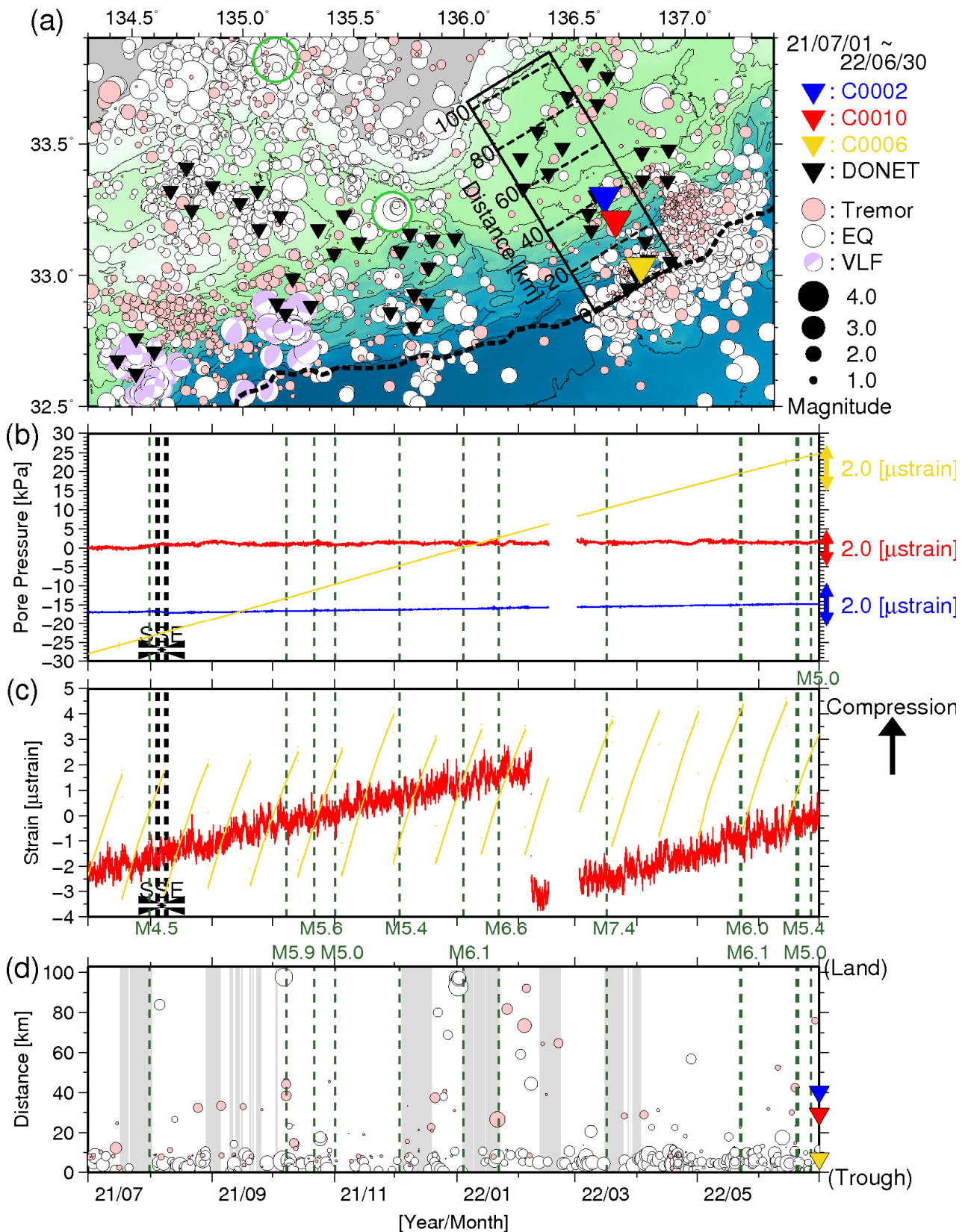
図4 直近1年間のSSE・低周波微動モニタリング(2021年7月1日~2022年6月30日)。(a)低周波微動・通常地震・超低周波地震の震央分布。(b)間隙水圧変化。(c)体積歪変化。(d)時空間分布。灰色はエアガン発振期間を示す。(b-d)の緑点線は、7月31日徳島県南部地震、10月7日千葉県北西部地震、10月21日東海道南方沖地震、11月1日和歌山県南方沖地震、12月3日紀伊水道地震、1月4日父島近海地震、1月22日日向灘地震、3月16日福島県沖地震、5月22日茨城県沖地震、5月23日八丈島東方沖地震、6月19日・20日能登地方地震、及び6月26日熊本地方地震。
