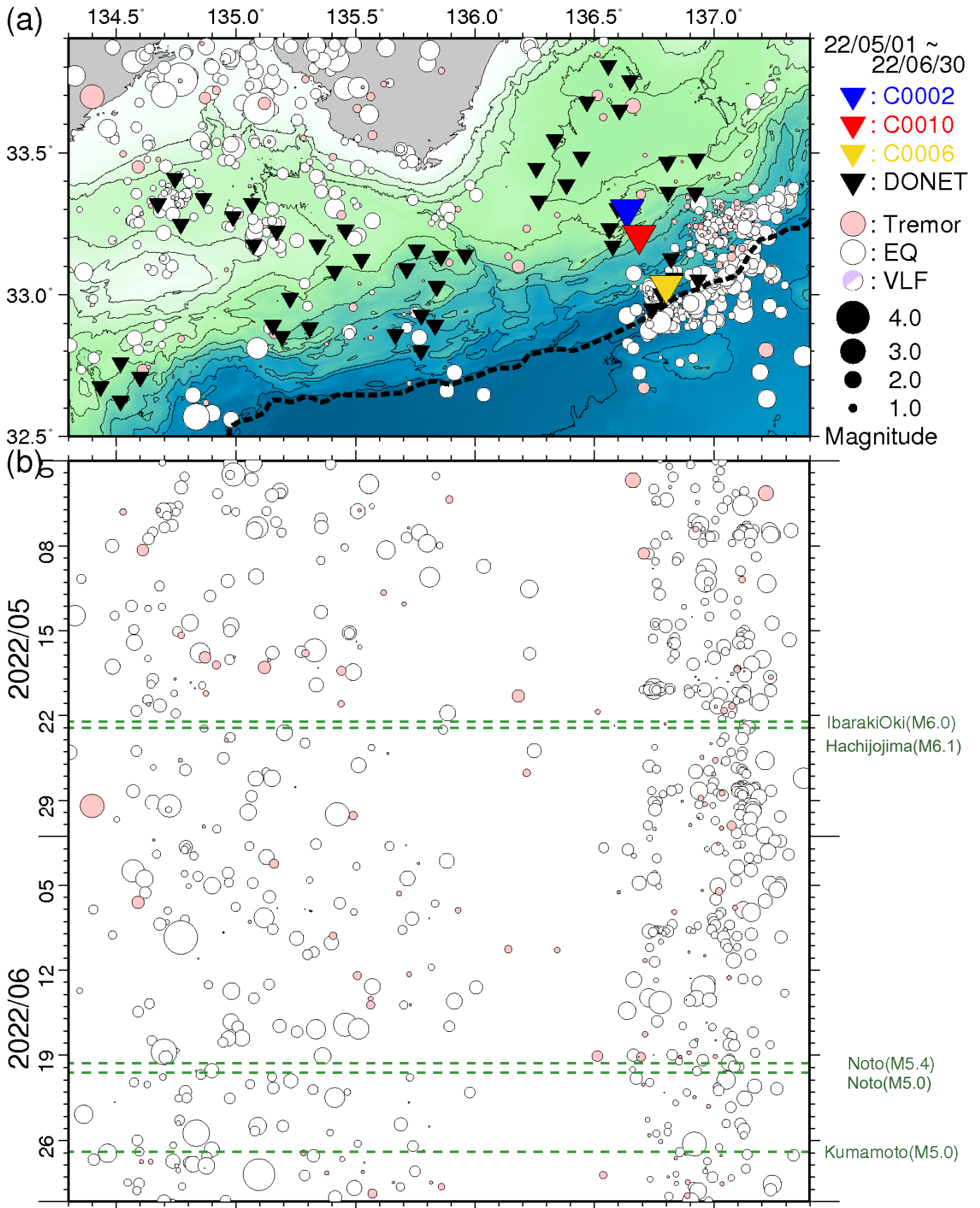
図5 直近2ヵ月間において熊野灘から室戸沖にて発生した低周波微動・通常地震・超低周波地震(2022年5月1日~2022年6月30日)。図3と同様のシンボルにて表示。(a)震央分布図。(b)aに示した震央を経度方向へ投影した時空間分布図。
