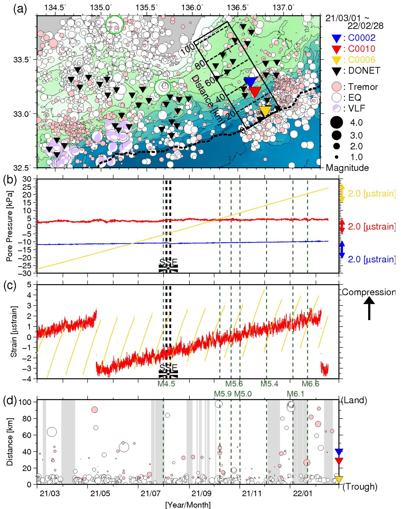
図4 直近1年間のSSE・低周波微動モニタリング(2021年3月1日~2022年2月28日)。図3と同様のシンボルにて表示。(a)低周波微動・通常地震・超低周波地震の震央分布。(b)間隙水圧変化。(c)体積歪変化。(d)時空間分布。灰色はエアガン発振期間を示す。(b-d)の緑点線は、7月31日徳島県南部地震、10月7日千葉県北西部地震、10月21日東海道南方沖地震、11月1日和歌山県南方沖地震、12月3日紀伊水道地震、1月4日父島近海地震、及び1月22日日向灘地震。
