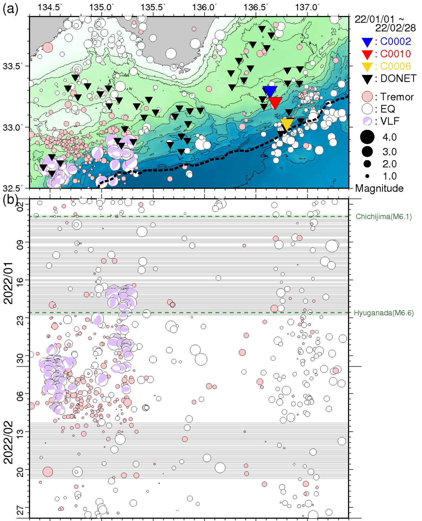
図5 直近2ヵ月間において熊野灘から室戸沖にて発生した低周波微動・通常地震・超低周波地震(2022年1月1日~2022年2月28日)。図3と同様のシンボルにて表示。(a)震央分布図。(b)aに示した震央を経度方向へ投影した時空間分布図。
