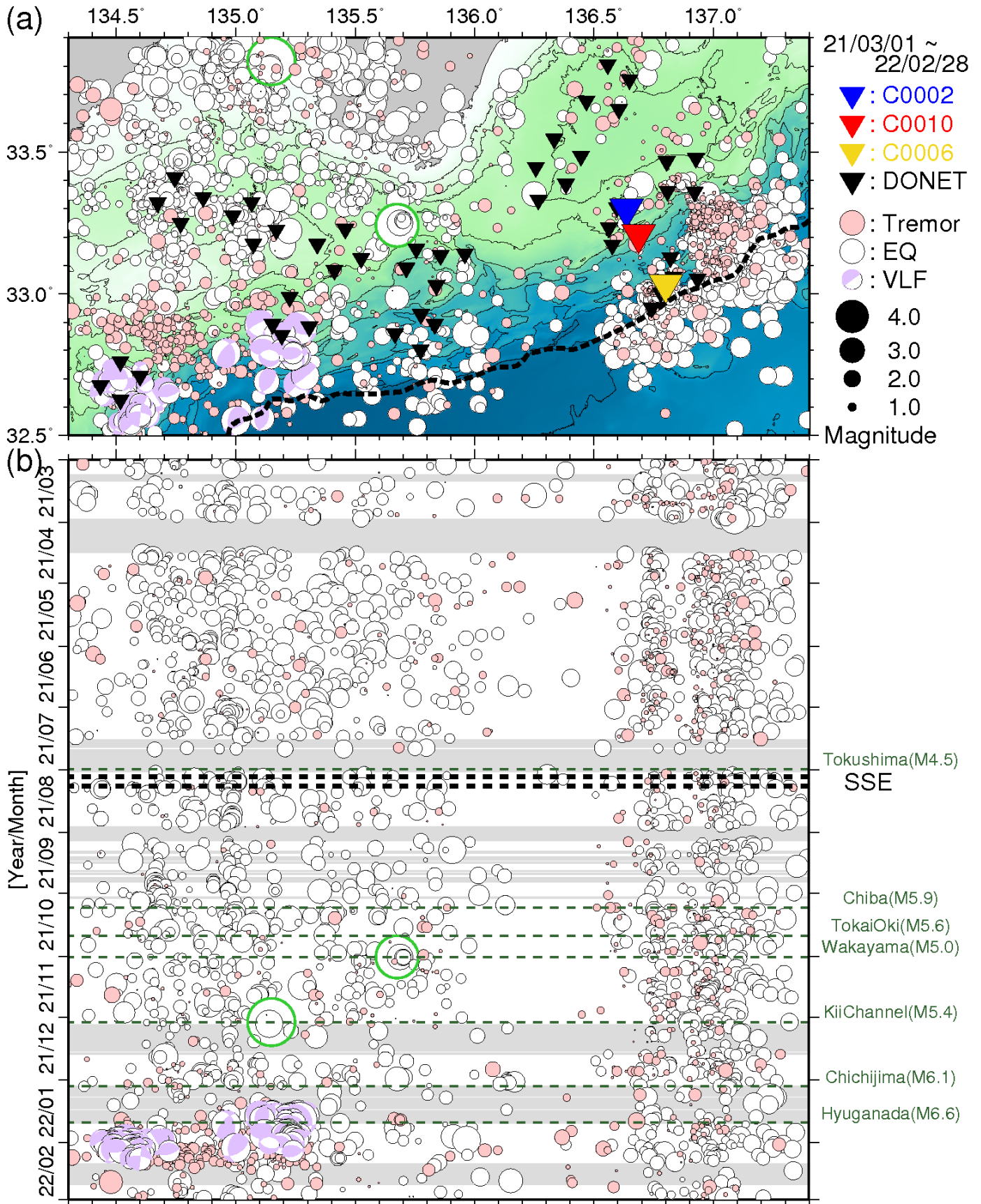
図 6 直近 1 年間に於いて熊野灘から室戸沖にて発生した低周波微動・通常地震・超低周波地震 (2021 年 3 月 1 日~2022 年 2 月 28 日)。図 4 と同様のシンボルにて表示。(a) 震央分布図。(b) a に示した震央を経度方向へ投影した時空間分布図。
