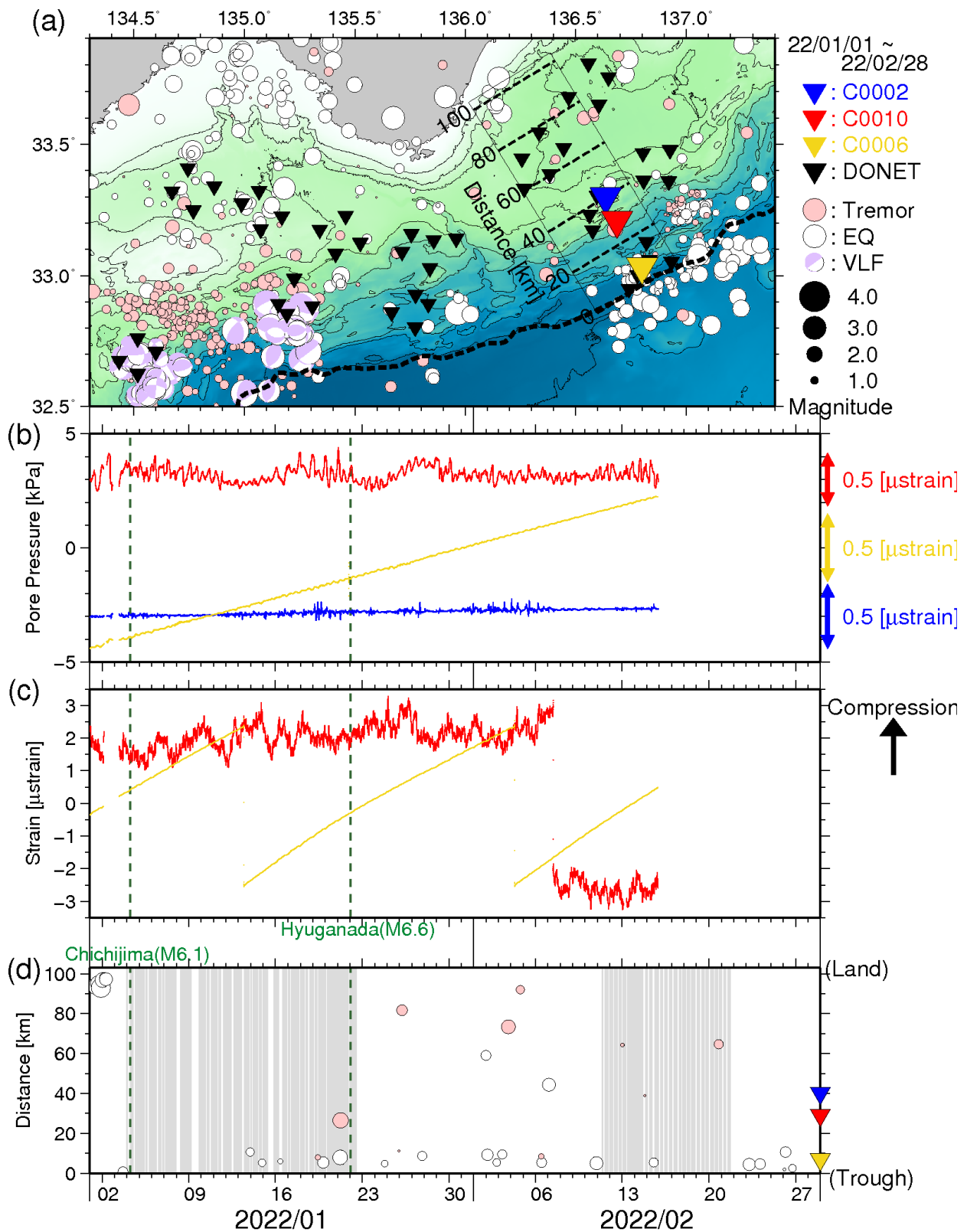
図3 直近2ヶ月間のSSE・低周波微動モニタリング(2022年1月1日~2022年2月28日)。(a)震央分布図(●:低周波微動(深さ0~15km)、○:通常地震(深さ0~60km)、●:超低周波地震のメカニズム解)。(b)長期孔内観測点における間隙水圧変化(—:C0002、—:C0010、—:C0006)。(c)長期孔内観測点における体積歪変化(—:C0010、—:C0006)。(d)図3a中に実線で示した矩形領域内における、低周波微動・通常地震・超低周波地震の時空間分布。灰色はエアガン発振期間。縦軸は、トラフ軸からの距離(km)。(b-d)の緑点線は、1月4日父島近海地震、及び1月22日日向灘地震。
