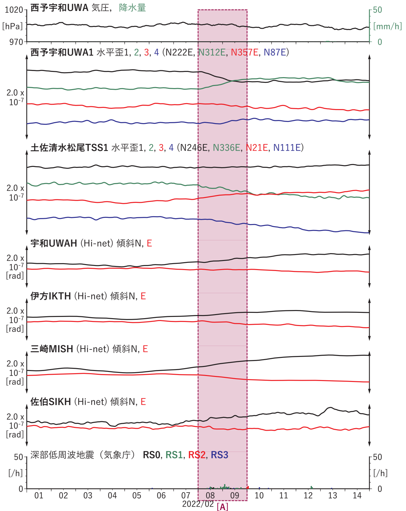
図5 歪・傾斜の時間変化 (2022/02/01 00:00-2022/02/15 00:00 (JST))
