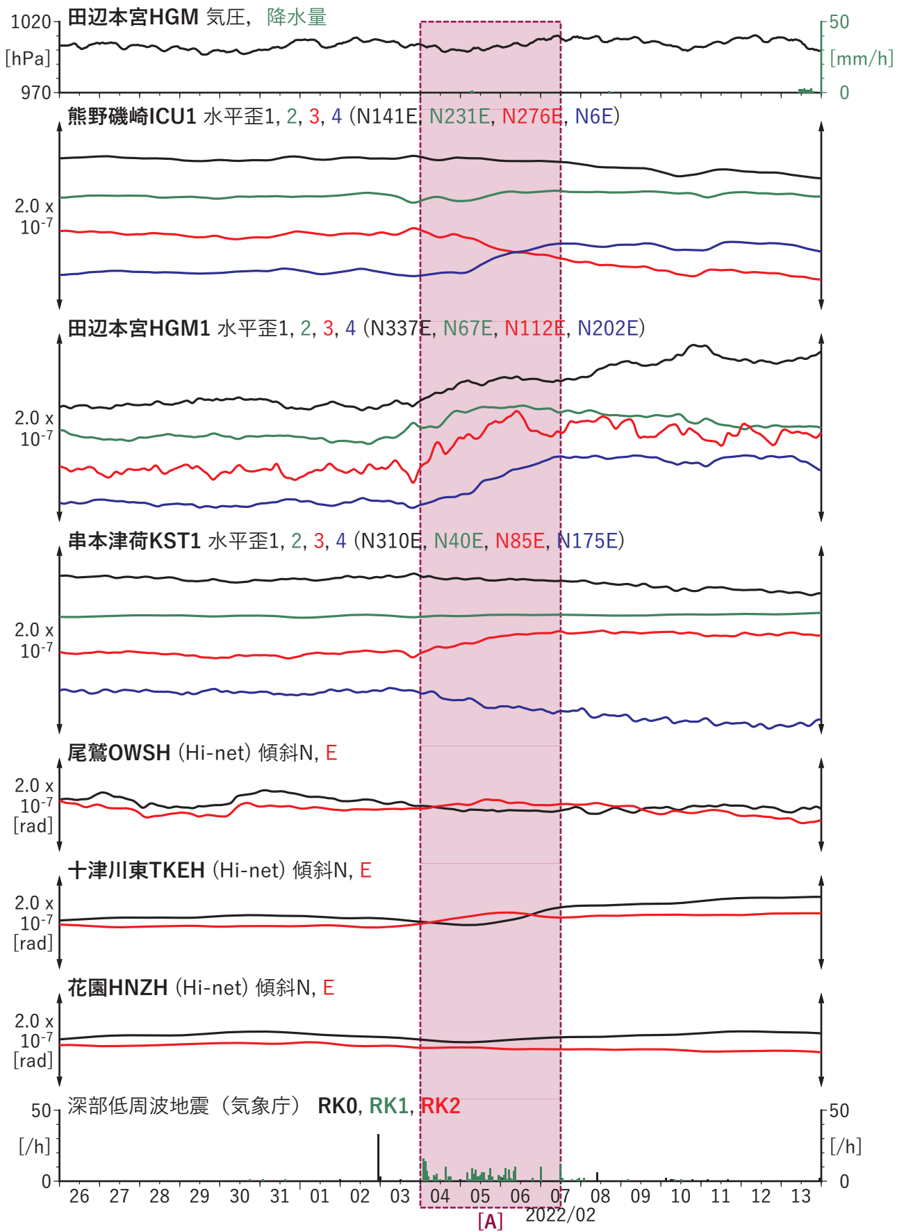
図2 歪・傾斜の時間変化 (2022/01/26 00:00-2022/02/14 00:00 (JST))
