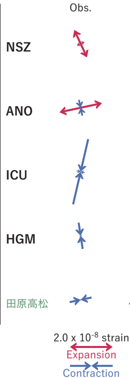
図3 2021/11/27-30の歪・傾斜・水位変化（図2[A]）を説明する断層モデル。
