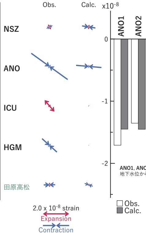
図4 2021/12/01-02の歪・傾斜・水位変化（図2[B]）を説明する断層モデル。
