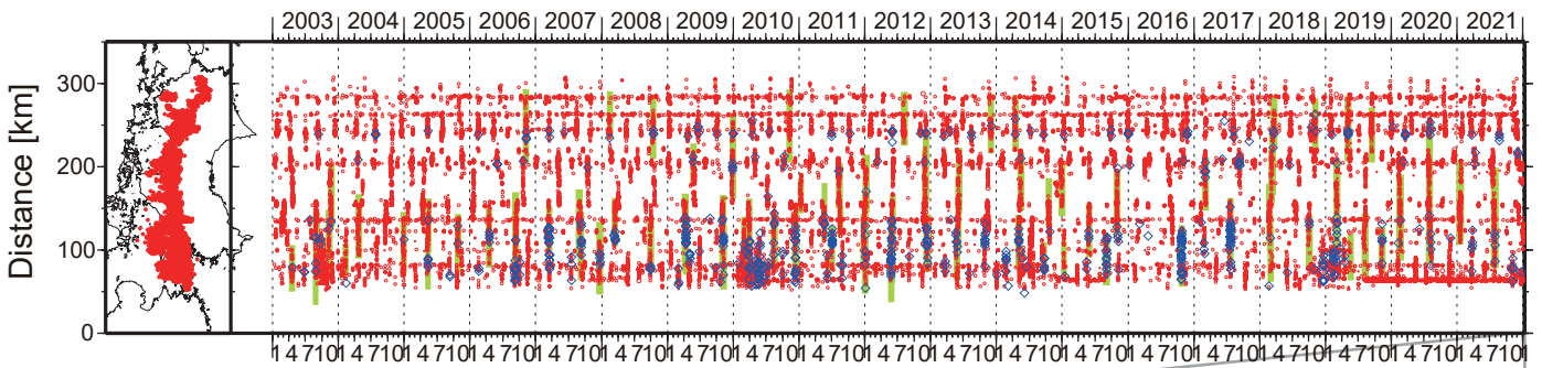
図1. 四国における2003年1月～2022年1月4日までの深部低周波微動の時空間分布(上図). 赤丸はエンベロープ相関・振幅ハイブリッド法 (Maeda and Obara, 2009) およびクラスタ処理 (Obara et al., 2010) によって1時間毎に自動処理された微動分布の重心である. 青菱形は周期20秒に卓越する超低周波地震 (Ito et al., 2007) である. 黄緑色太線は、これまでに検出された短期的スロースリップイベント (SSE) を示す. 下図は2021年12月を中心とした期間の拡大図である.
