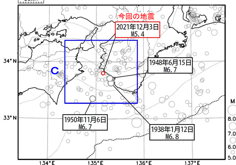
震央分布図 (1919年1月1日～2021年12月31日、 深さ0～100km、 M \geq 5.0 )
