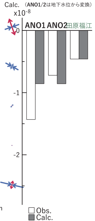
(b3) 体積歪
