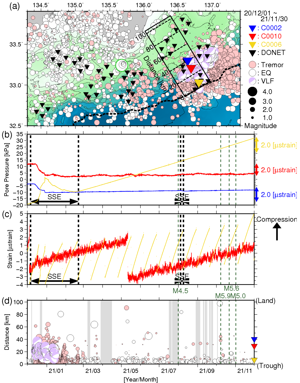
図4 直近1年間のSSE・低周波微動モニタリング(2020年12月1日~2021年11月30日)。図3と同様のシンボルにて表示。(a)低周波微動と通常地震の震央分布図。(b)間隙水圧変化。(c)体積歪変化。(d)時空間分布。超低周波地震のメカニズム解(●)も合わせて示す。体積歪変化は、基準値を超えると歪計内のバルブを開けてリセットするため、相対値のみを使用。灰色は、2020年12月7日~8日、21日~24日はサーバ不具合・入替期間、その他はエアガン発振期間を示す。(b-d)の緑点線は、2021年7月31日徳島県南部地震、2021年10月7日千葉県北西部地震、2021年10月21日東海道南方沖地震、および2021年11月1日和歌山県南方沖地震を示す。
