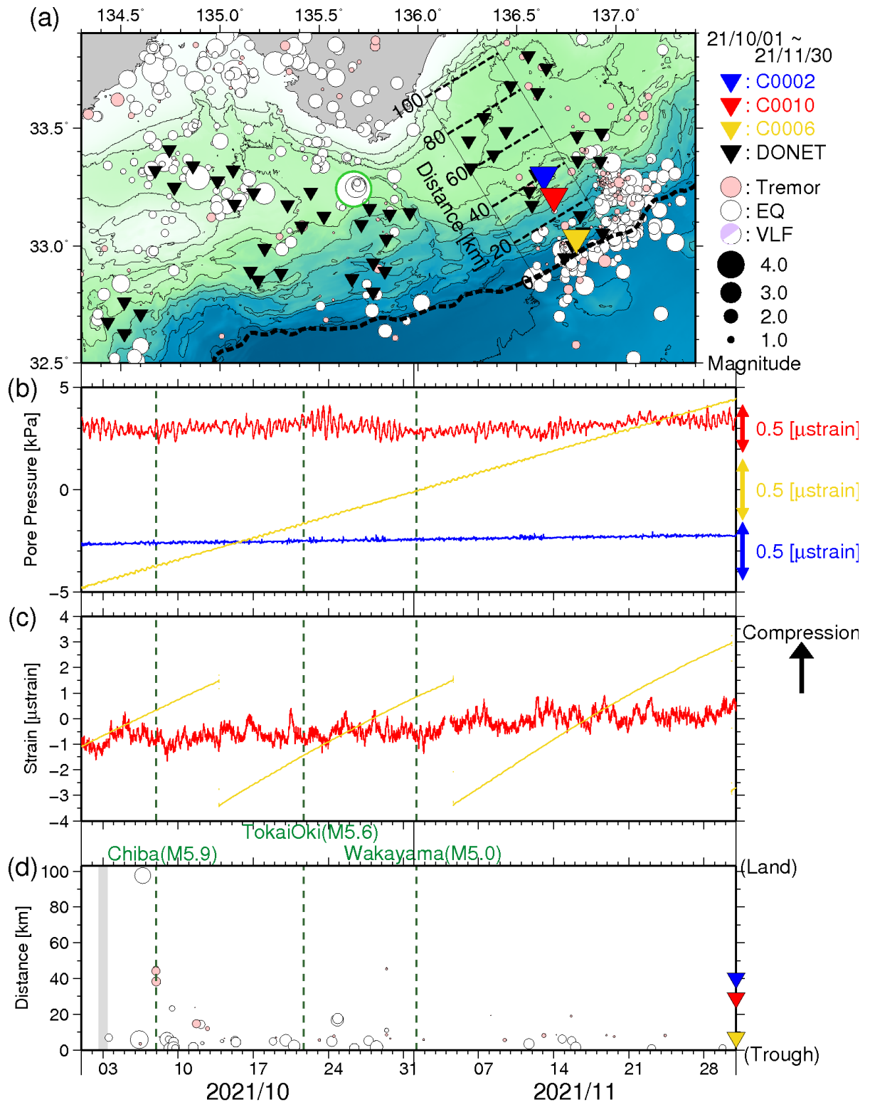
図3 直近2ヶ月間のSSE・低周波微動モニタリング(2021年10月1日~2021年11月30日)。(a)低周波微動と通常地震の震央分布図(●:低周波微動、○:通常地震)。それぞれ震源深さが、0~15km及び0~60kmの範囲に決まったイベントのみを表示。○は2021年11月1日和歌山県南方沖地震(M5.0)。▼▼▼は、それぞれC0002・C0010・C0006・DONET観測点を示す。破線はトラフ軸を示す。(b)長期孔内観測点における間隙水圧変化(—:C0002、—:C0010、—:C0006)。(c)長期孔内観測点における体積歪変化(—:C0010、—:C0006)。(d)図3a中に実線で示した矩形領域内における、低周波微動と通常地震の時空間分布。灰色はエアガン発振期間。縦軸は、トラフ軸からの距離(km)を示す。(b-d)の緑点線は、2021年10月7日千葉県北西部地震、2021年10月21日東海道南方沖地震、および2021年11月1日和歌山県南方沖地震を示す。
