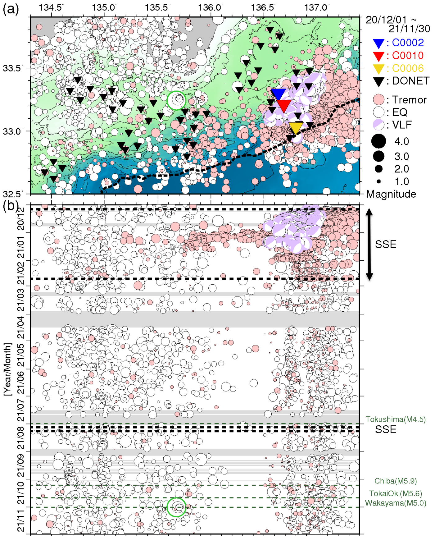
図 6 直近 1 年間に於いて熊野灘から室戸沖にて発生した低周波微動と通常地震の時空間分布 (2020 年 12 月 1 日~2021 年 11 月 30 日)。図 4 と同様のシンボルにて表示。(a) 震央分布図。(b) a に示した震央を経度方向へ投影した時空間分布図。超低周波地震のメカニズム解も合わせて示す。
