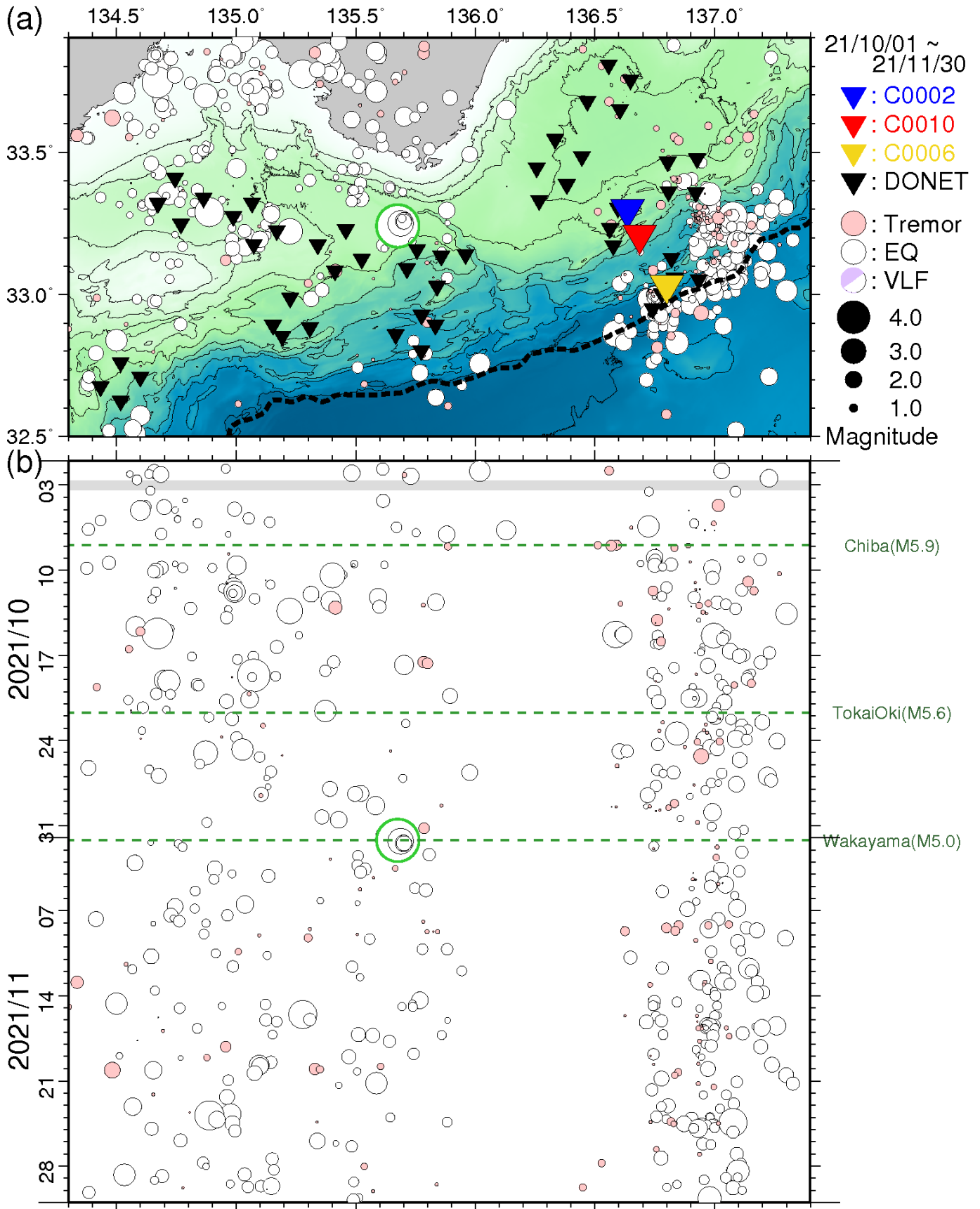
図 5 直近 2 ヶ月間において熊野灘から室戸沖にて発生した低周波微動と通常地震の時空間分布 (2021 年 10 月 1 日~2021 年 11 月 30 日)。図 3 と同様のシンボルにて表示。(a) 震央分布図。(b) a に示した震央を経度方向へ投影した時空間分布図。
